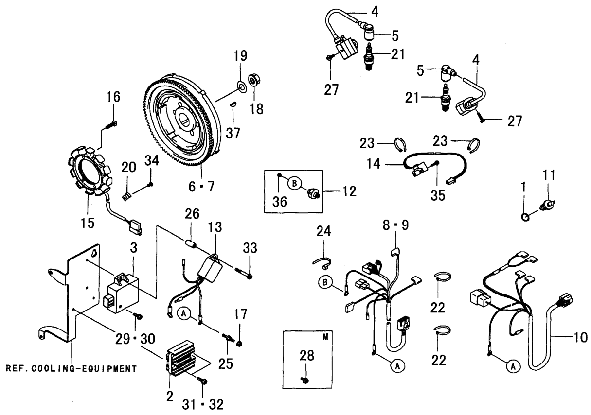
FIG. 6 ELECTRIC-EQUIPMENT
