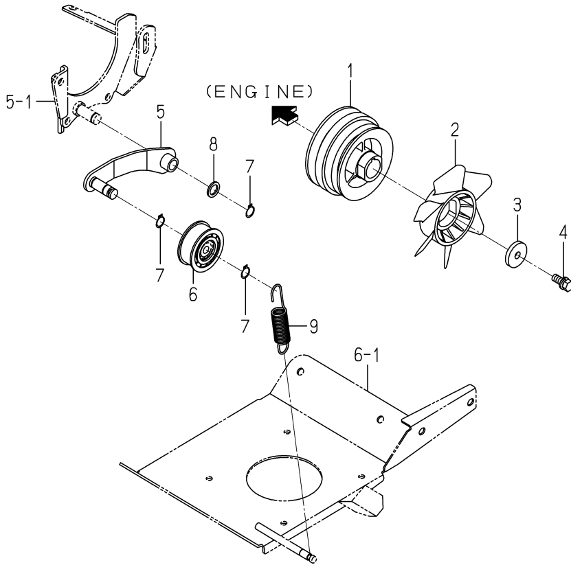
FIG. 7 PULLEY(ENGINE)SYSTEM(GF TYPE)
