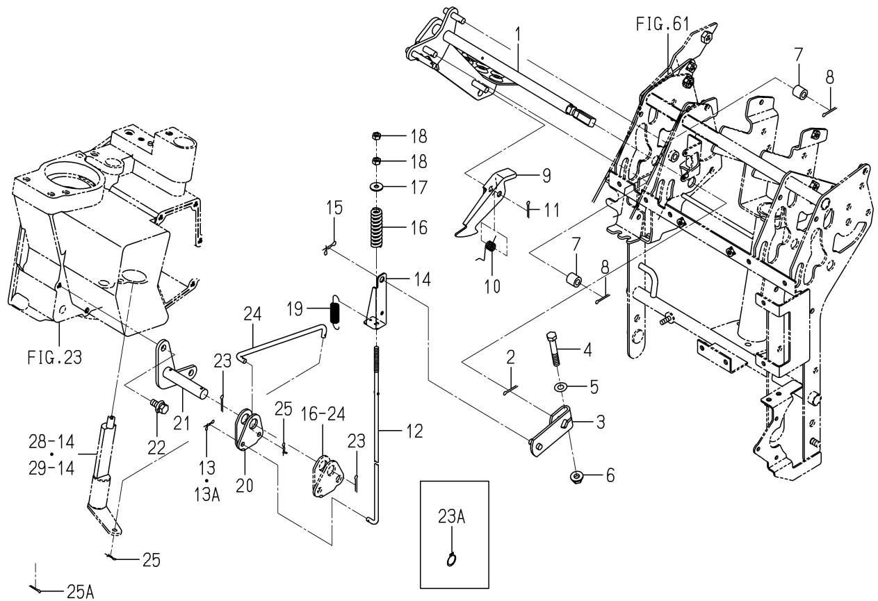
FIG. 62 CASE(REAR)SYSTEM
