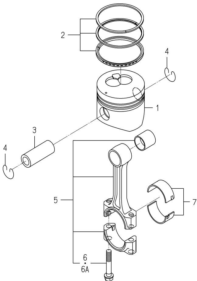
FIG. 14 PISTON
