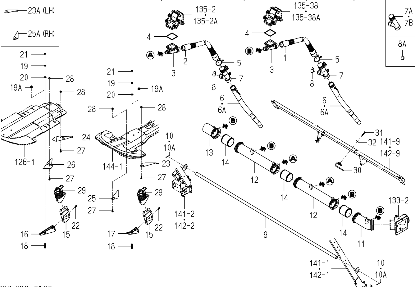
FIG.137 PIPING(FERTILIZER)SYSTEM(F TYPE)
