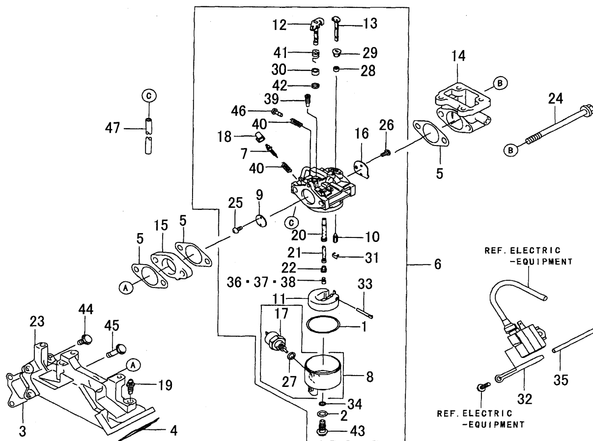
FIG. 8 CARBURETOR
