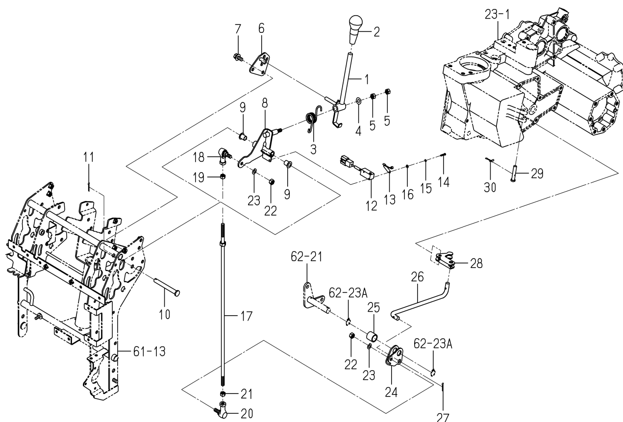
FIG. 16 LEVER(SUB)SYSTEM
