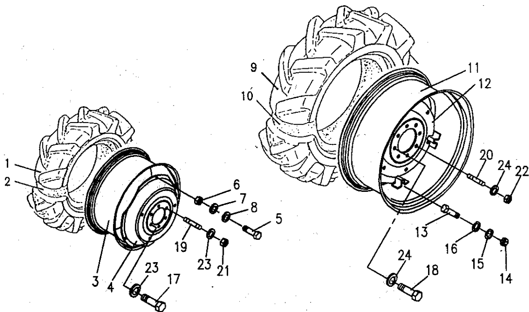
앞, 뒤 타이어 FRONT & REAR WHEEL (490)
