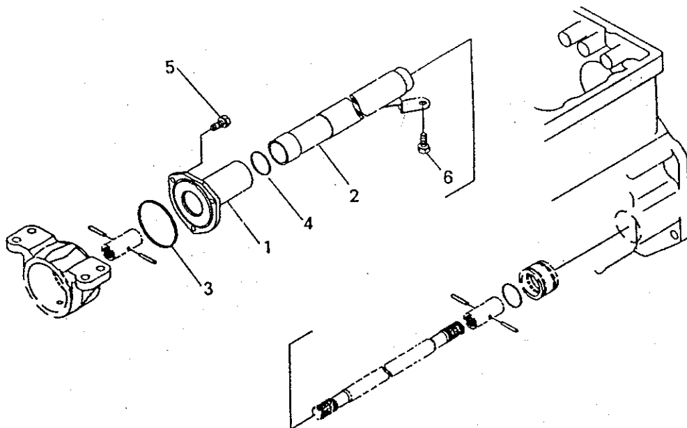
4륜 구동 카버 4WD PROP. COVER (380)
