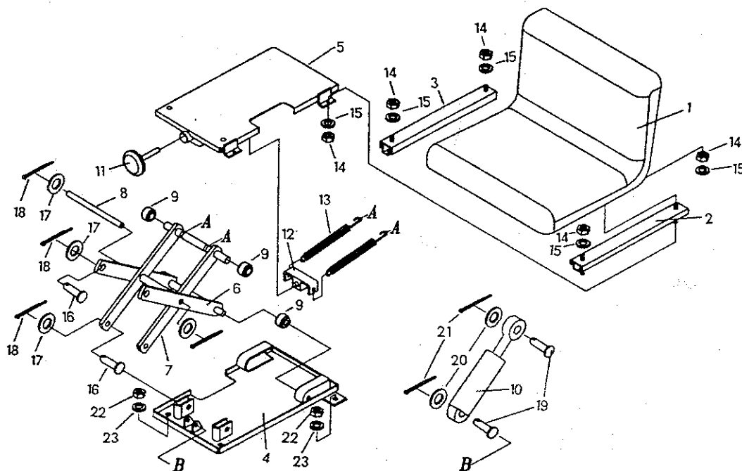
시트 조합 SEAT ASSY(850)
