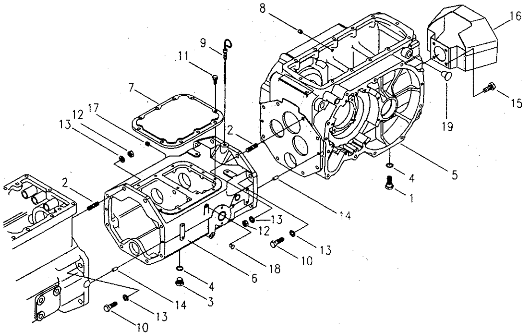
트랜스 미션 케이스 FIG 3-5 TRANSMISSION CASE (280)
