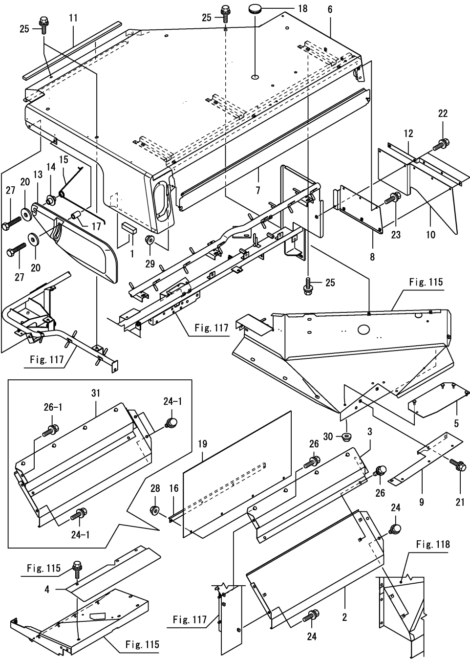
Fig.116. 상단 몸체(배출구)(2)
