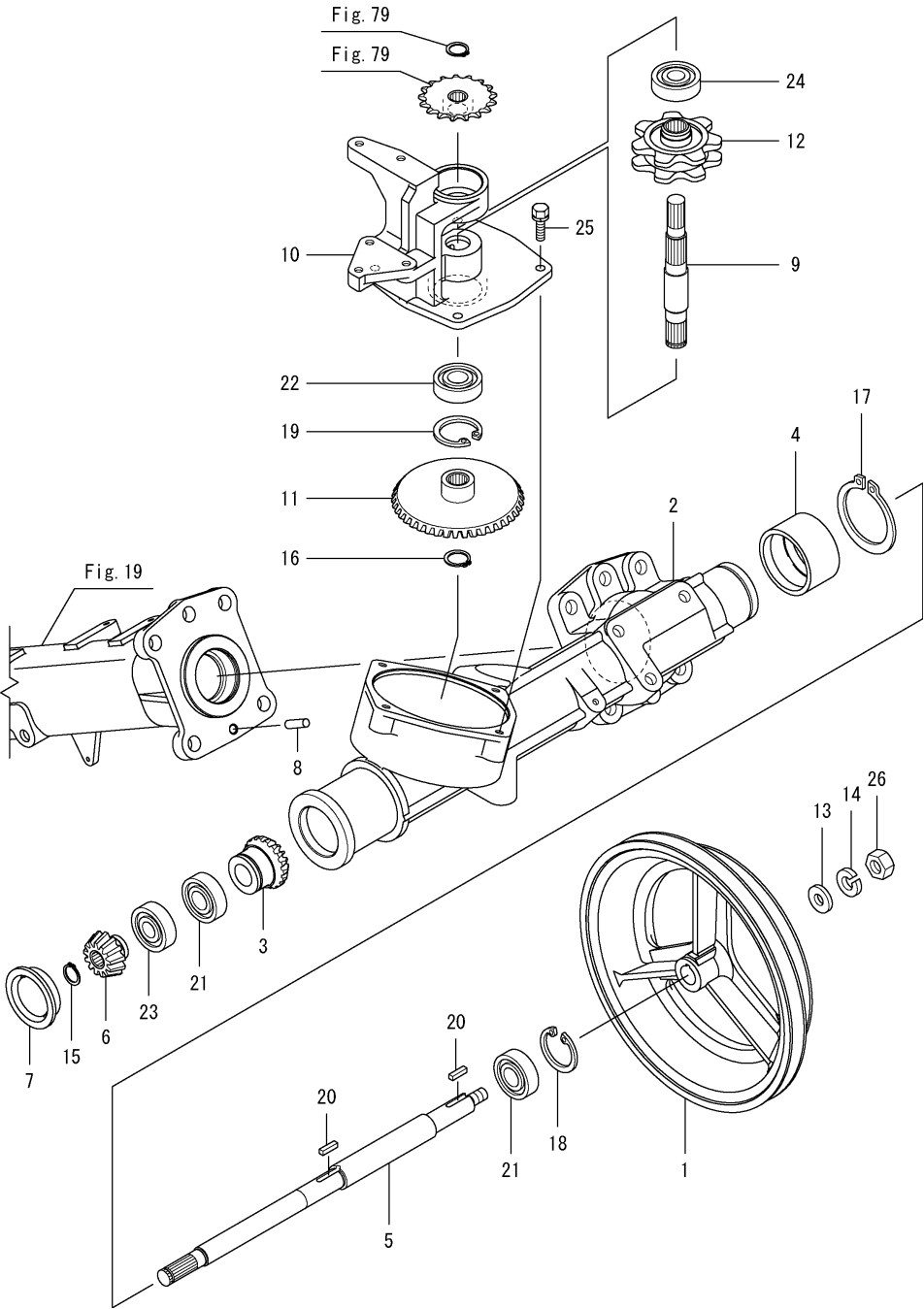
Fig.17. 입력구동케이스
