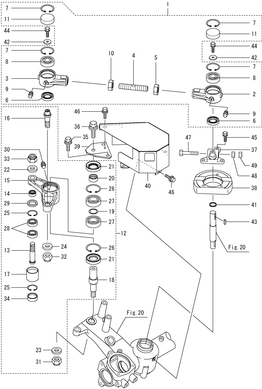
Fig.48. 예취날구동(좌)
