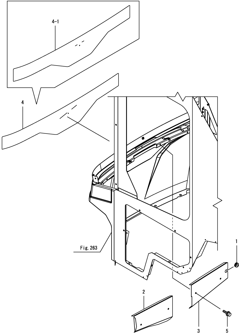
Fig.267. 캐빈의장(앞-하)
