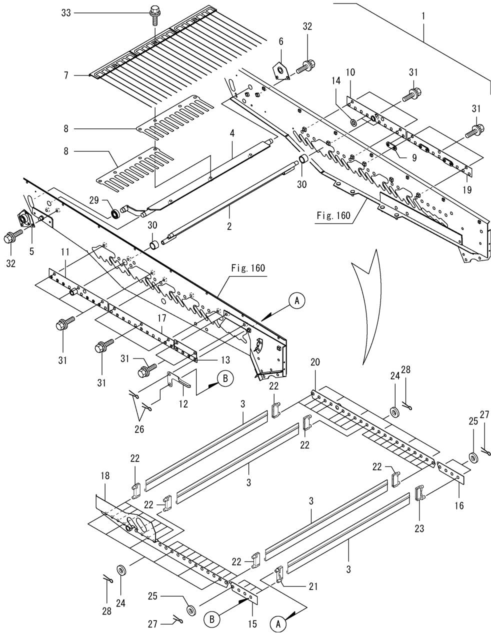
Fig.161. 요동선별판(2)
