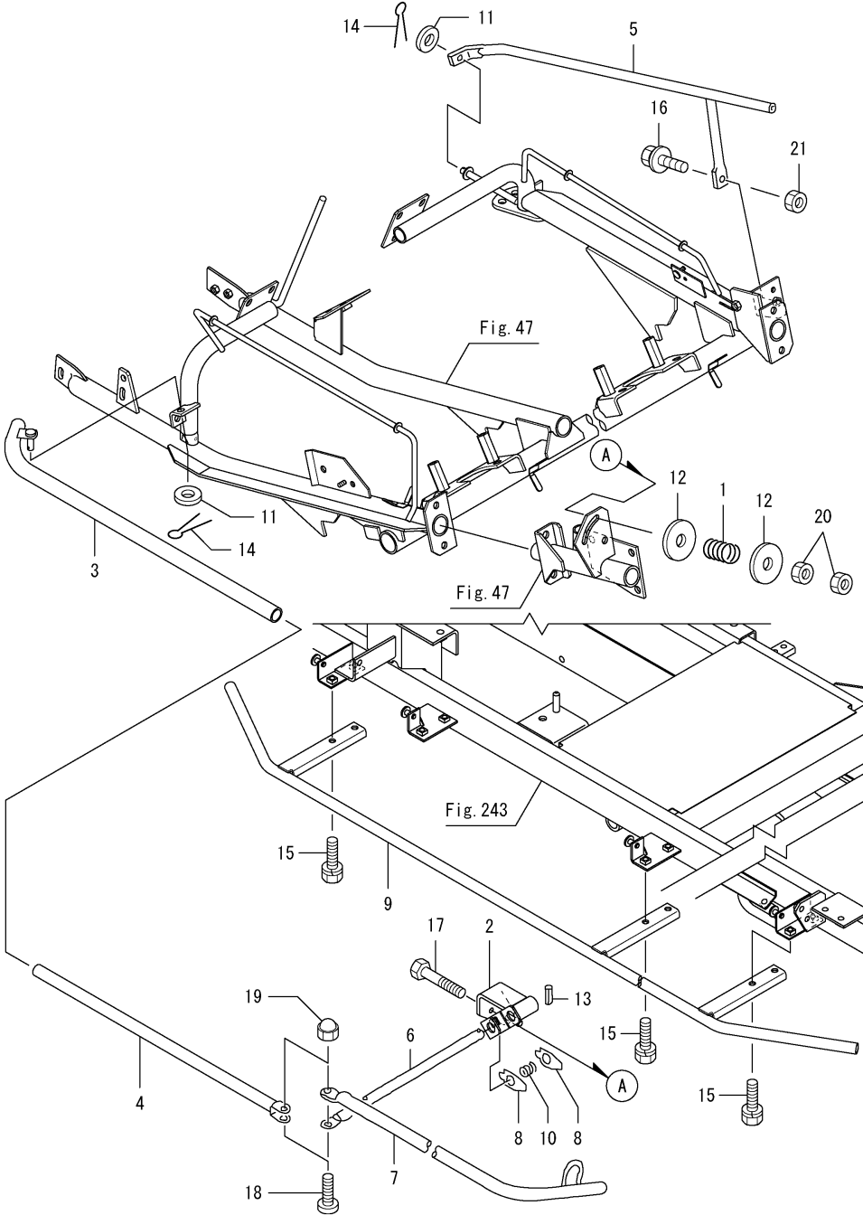
Fig.55. 보조분초간
