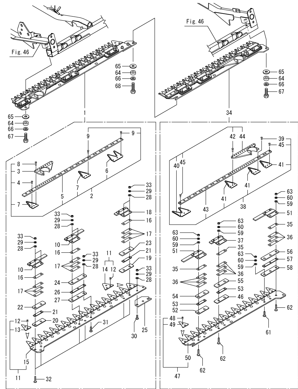
Fig.51. 예취날
