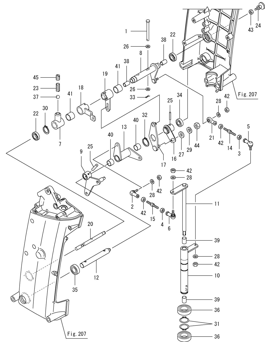
Fig.211. 스티어링 조작(3)
