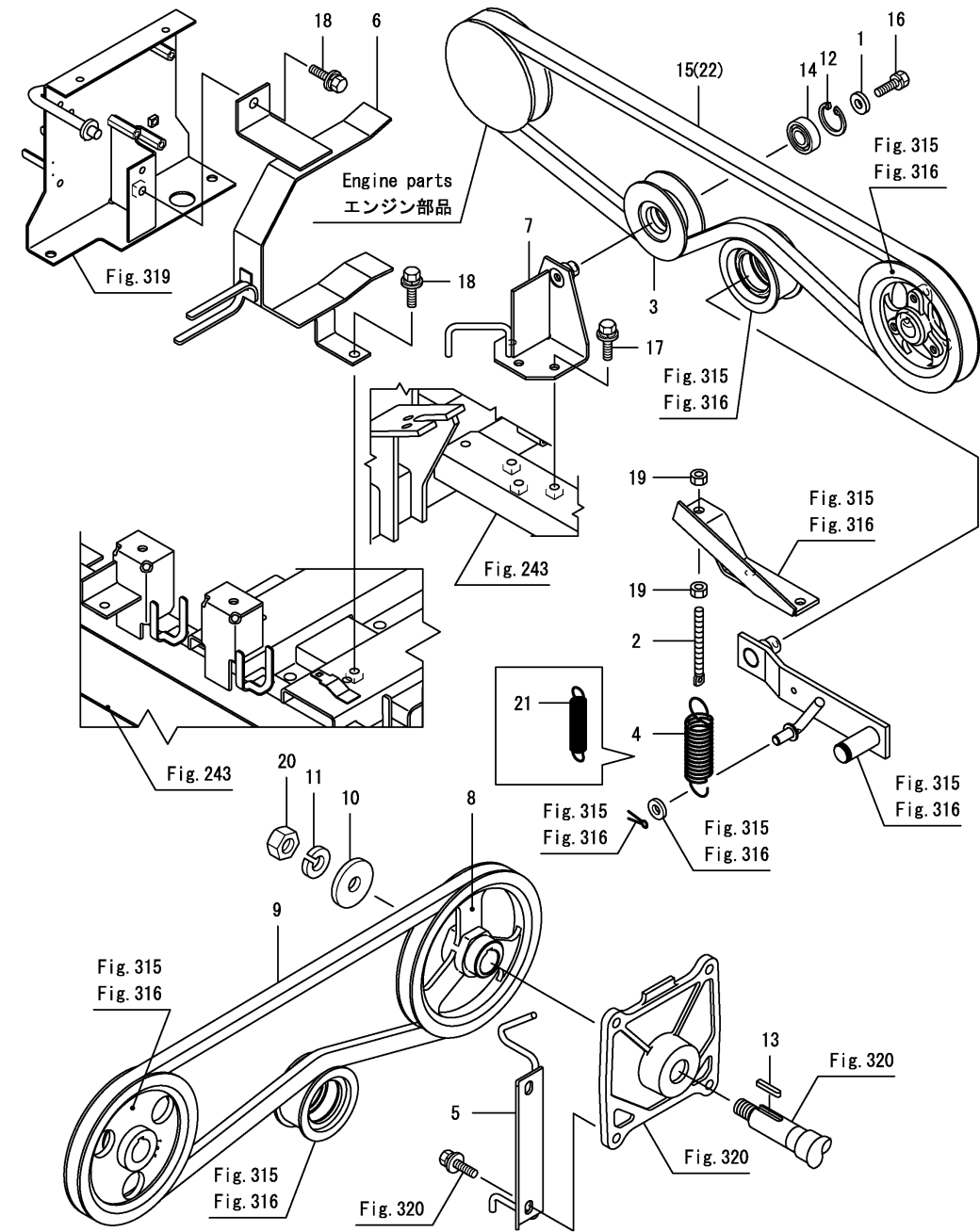
Fig.318. 오거 벨트
