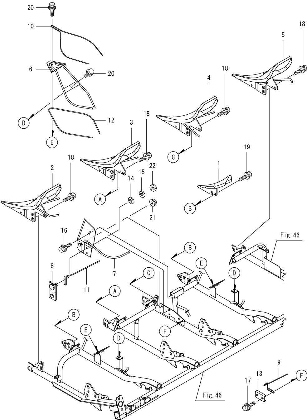
Fig.53. 분초판
