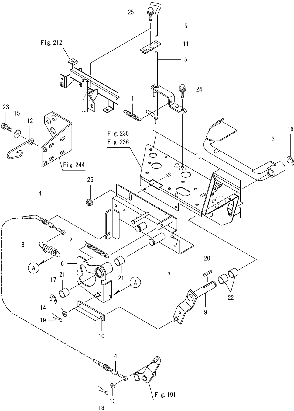
Fig.218. 브레이크조작
