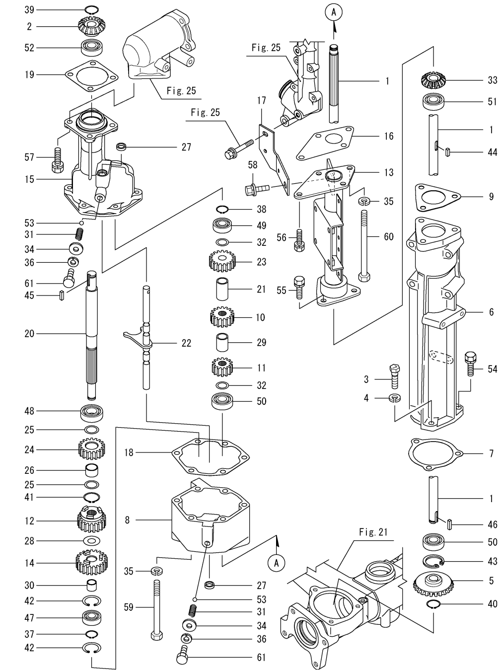
Fig.24. 픽업 수직 드라이브
