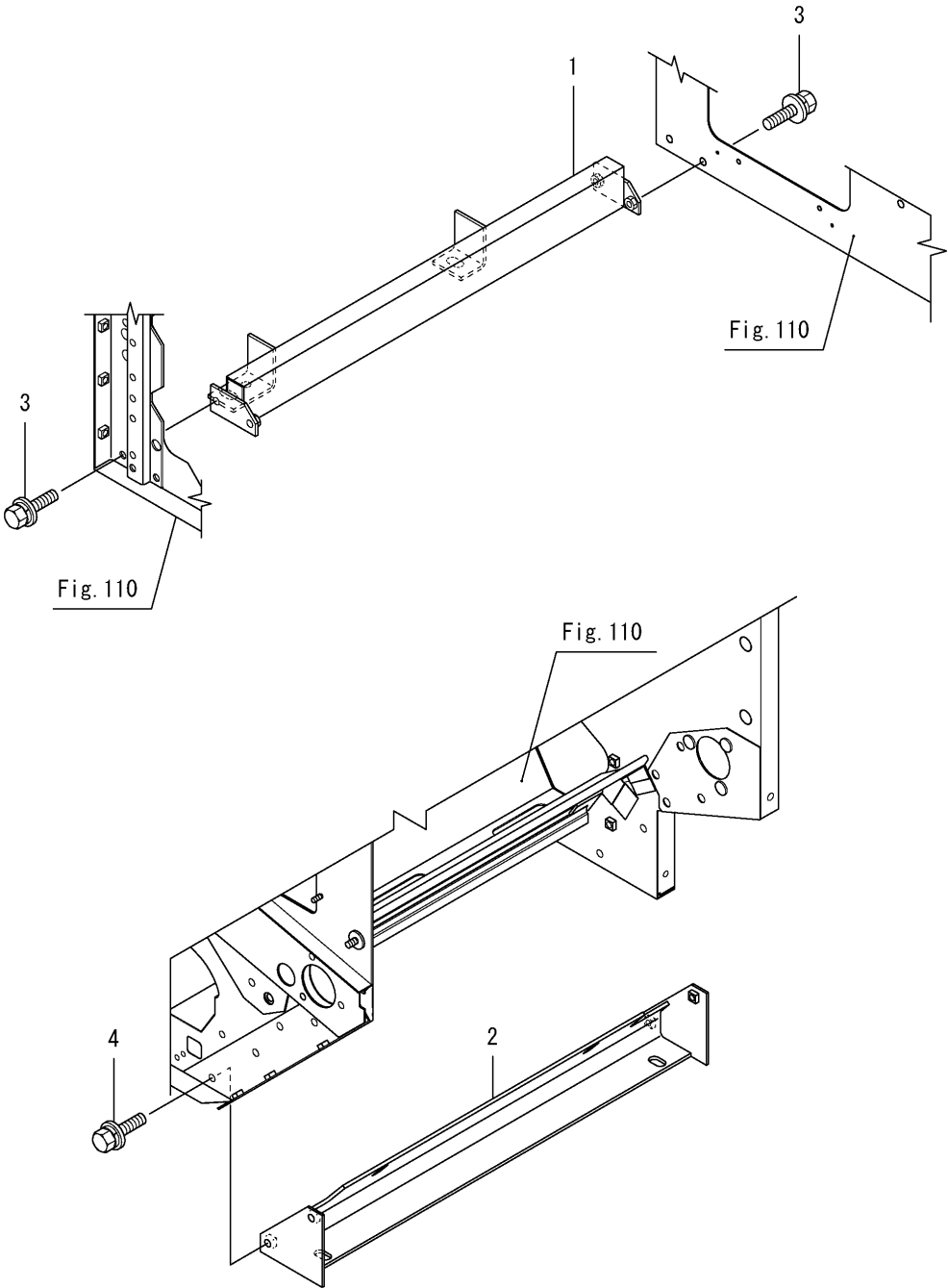
Fig.112. 탈곡취부(1)
