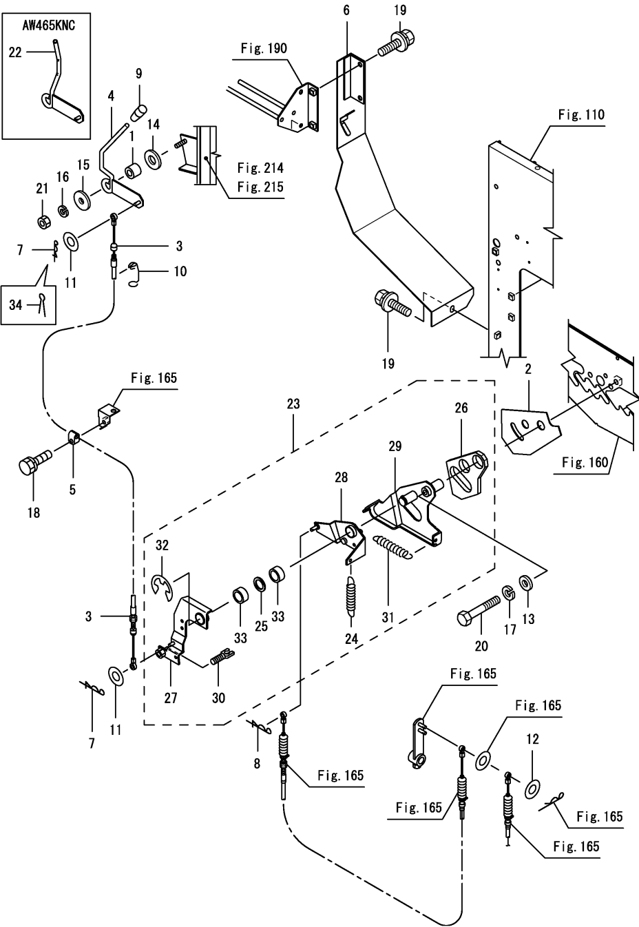
Fig.163. 요동선별조작(1)
