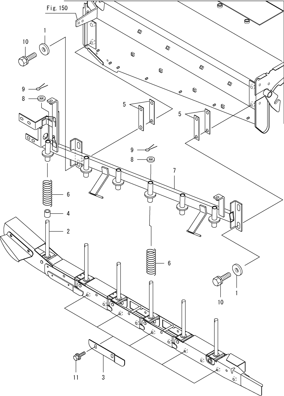
Fig.183. 쥔 고정 플레이트
