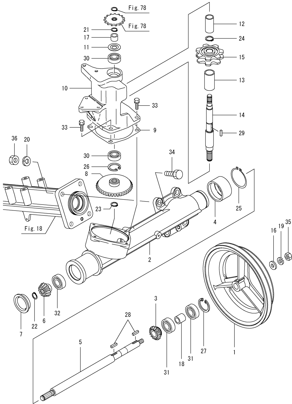
Fig.16. 입력구동케이스
