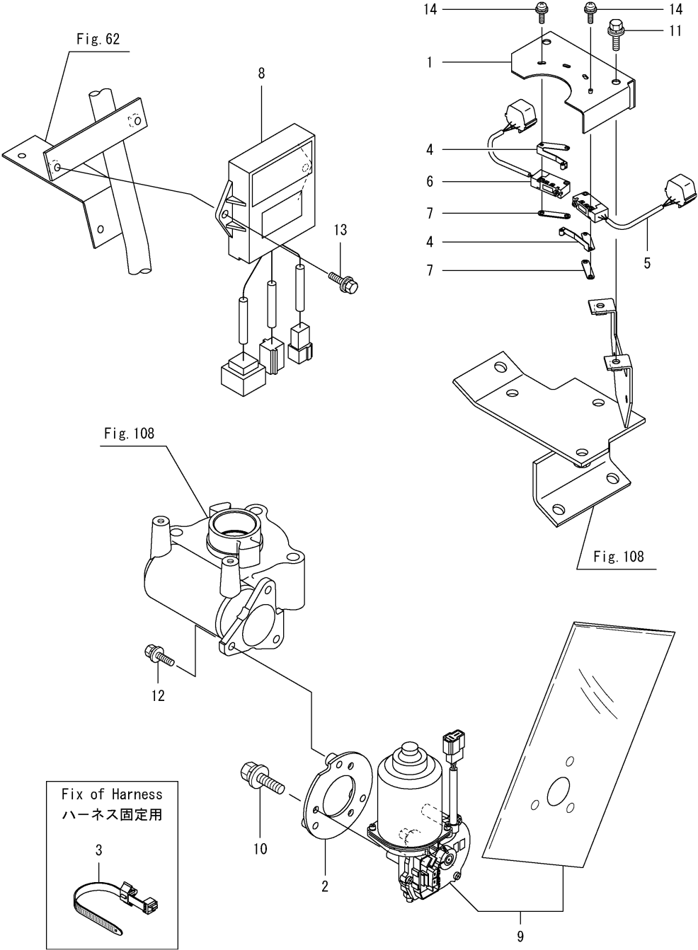
Fig.304. 공급 깊이 조작
