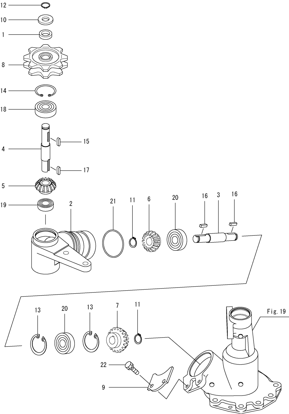
Fig.98. 수직 이송 케이스
