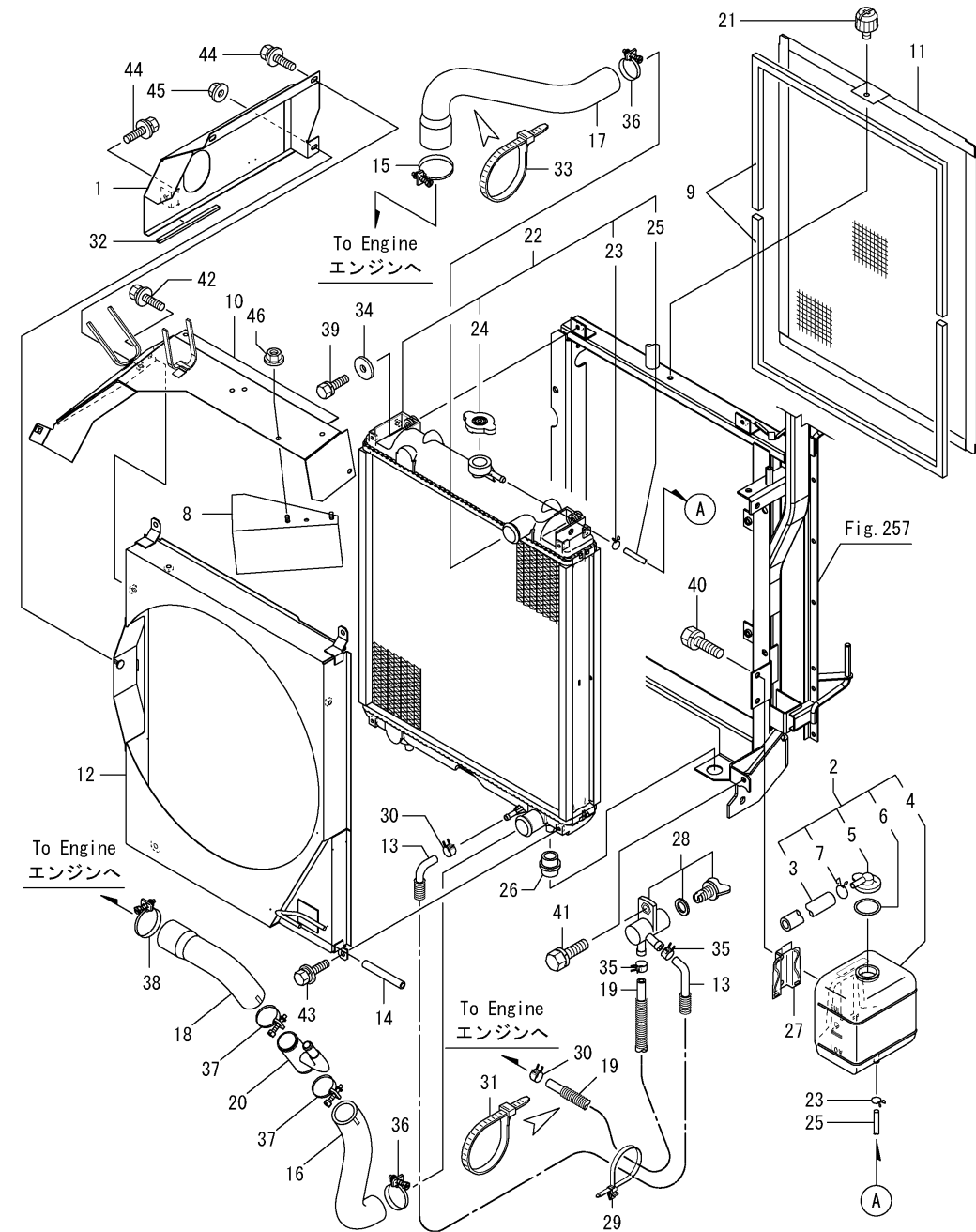
Fig.13. 라디에이터(캐빈)
