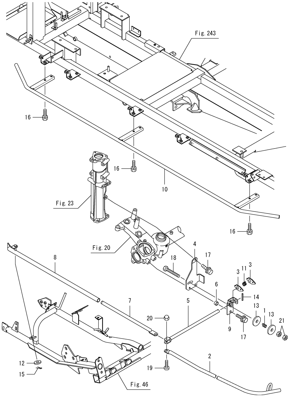
Fig.56. 보조분초간
