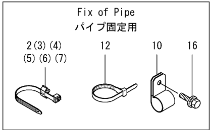
Fig.341. 주유장치(1)
