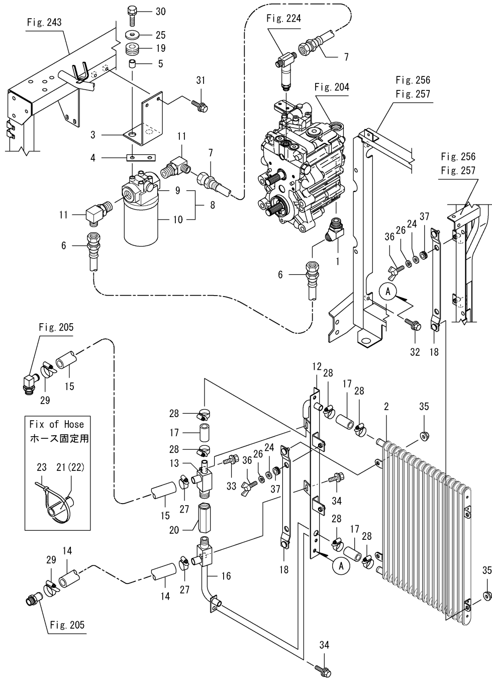
Fig.225. 배관(H.S.T.)
