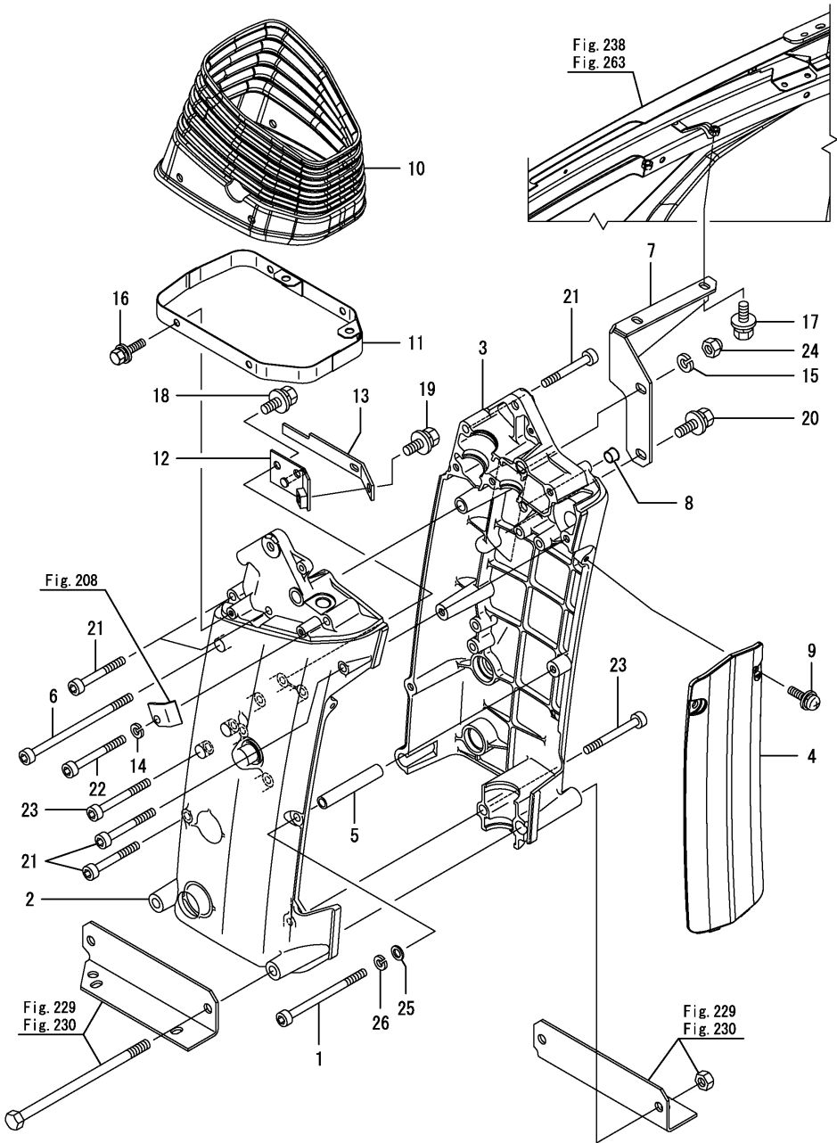
OCNP5-M34400 이동(2) Fig.207. 스티어링칼럼
