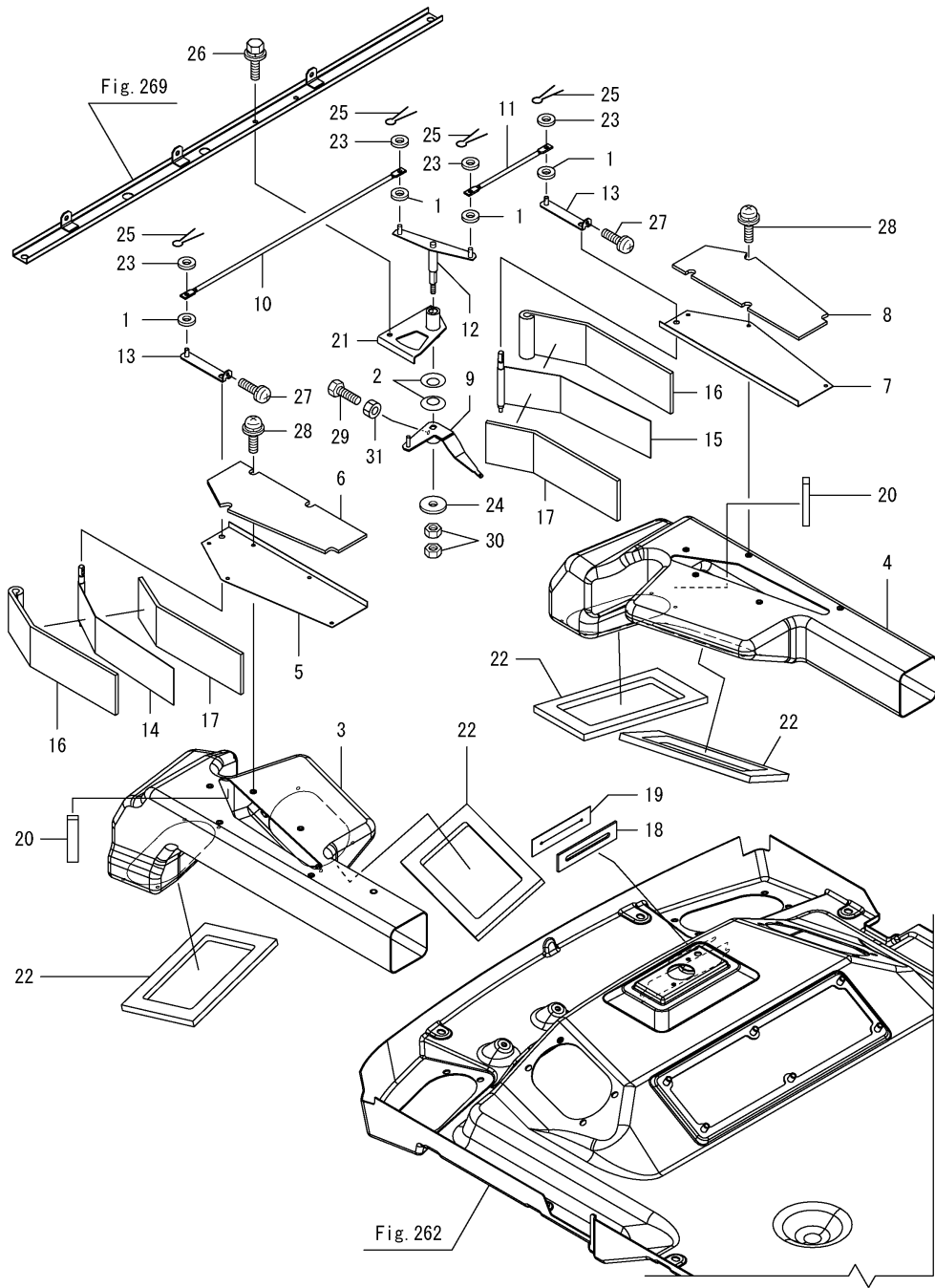
Fig.272. 에어컨덕트
