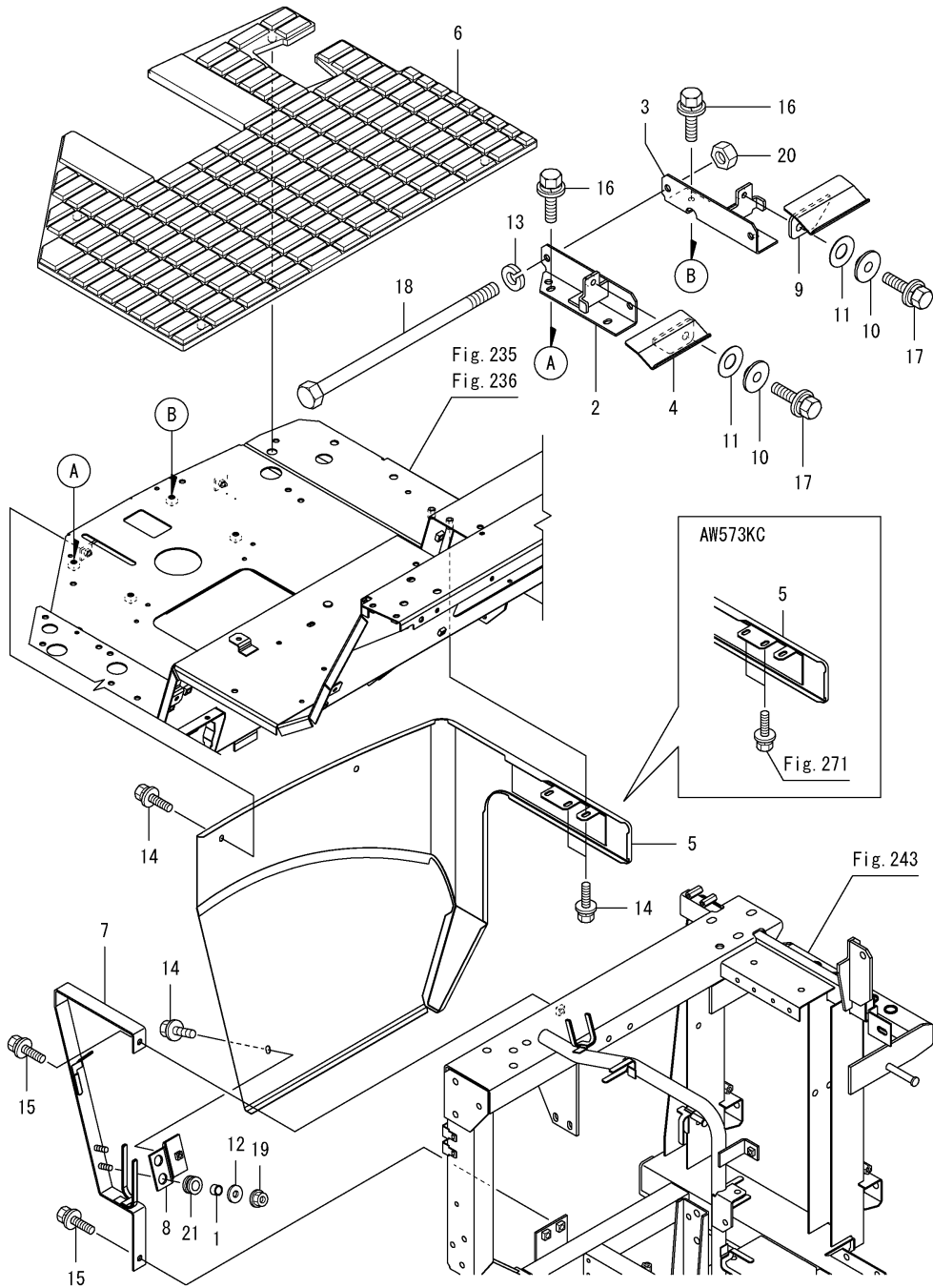
Fig.230. 발판
