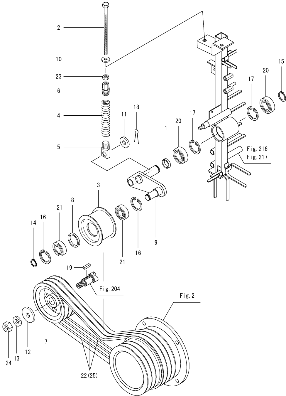
Fig.188. 이동 벨트
