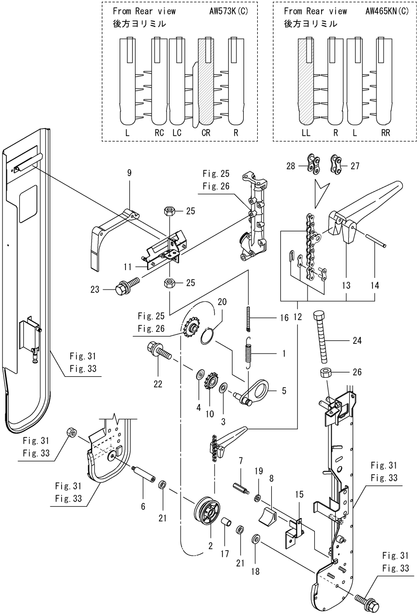
Fig.37. 인기체인롤러(중-우)
