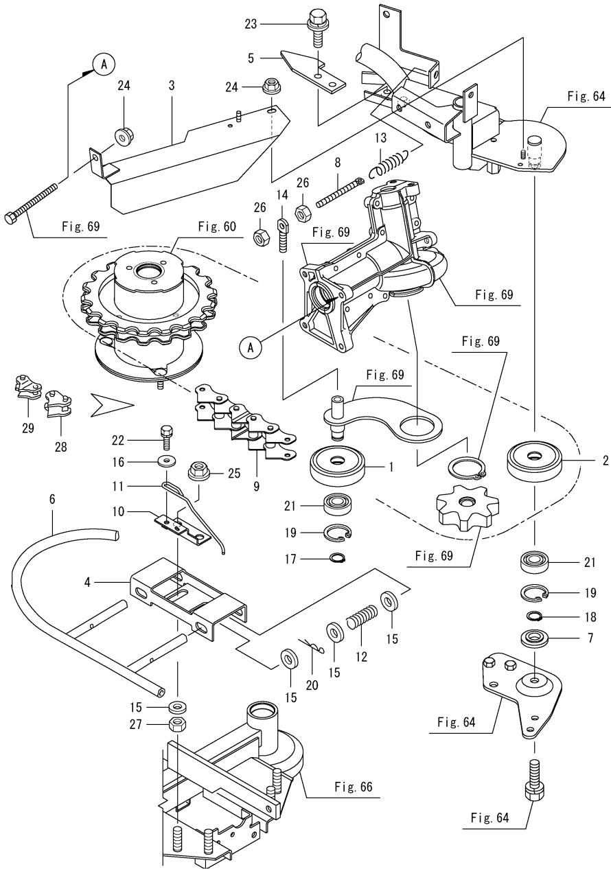
0CNP5-M34400 수확(2) Fig.76. 하단 이송 가이드(왼쪽)
