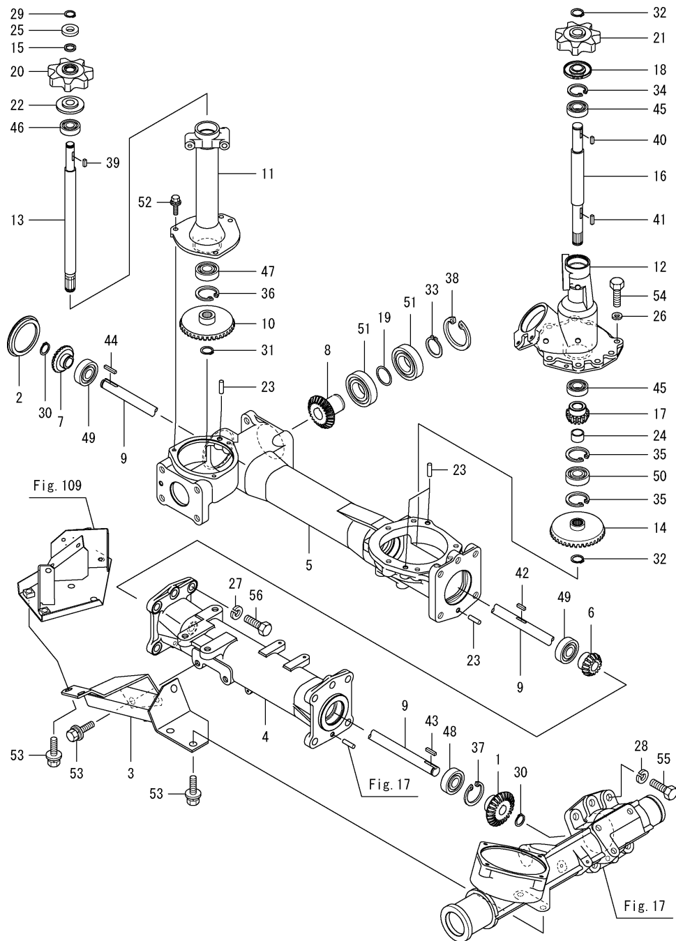
Fig.19. 축 케이스(2차)
