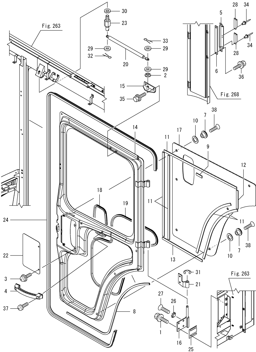
Fig.273. 캐빈(문)(1)
