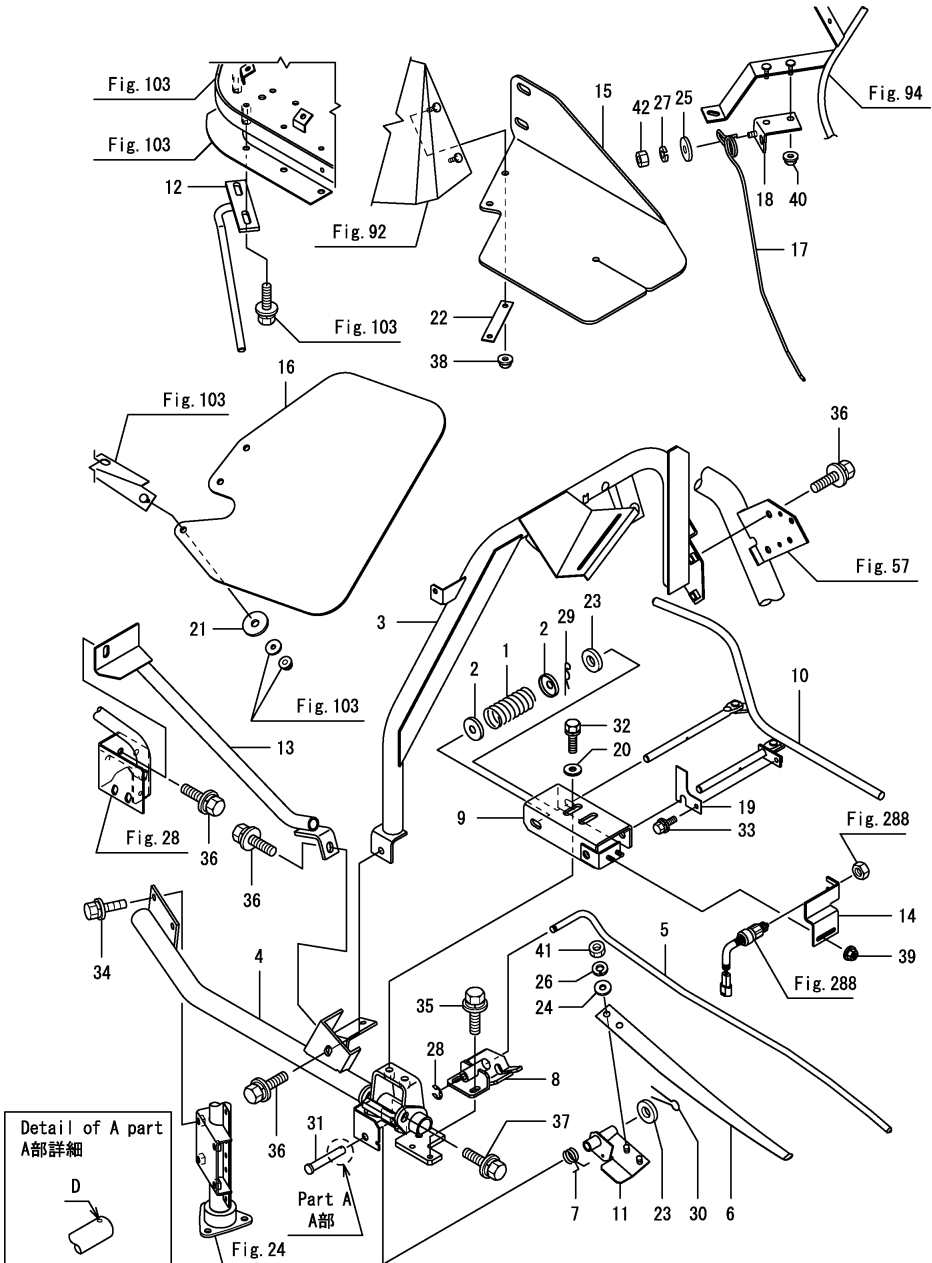
OCNP5-M34400 수확(2) Fig.106. 보조반송가이드(캐빈)
