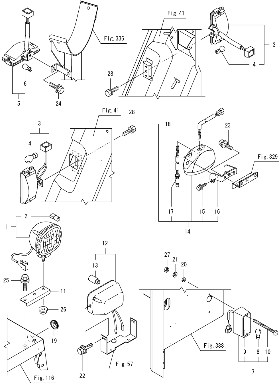
Fig.281. 램프(곡물탱크)
