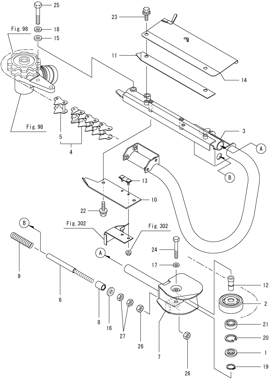
Fig.100. 수직 체인 케이스
