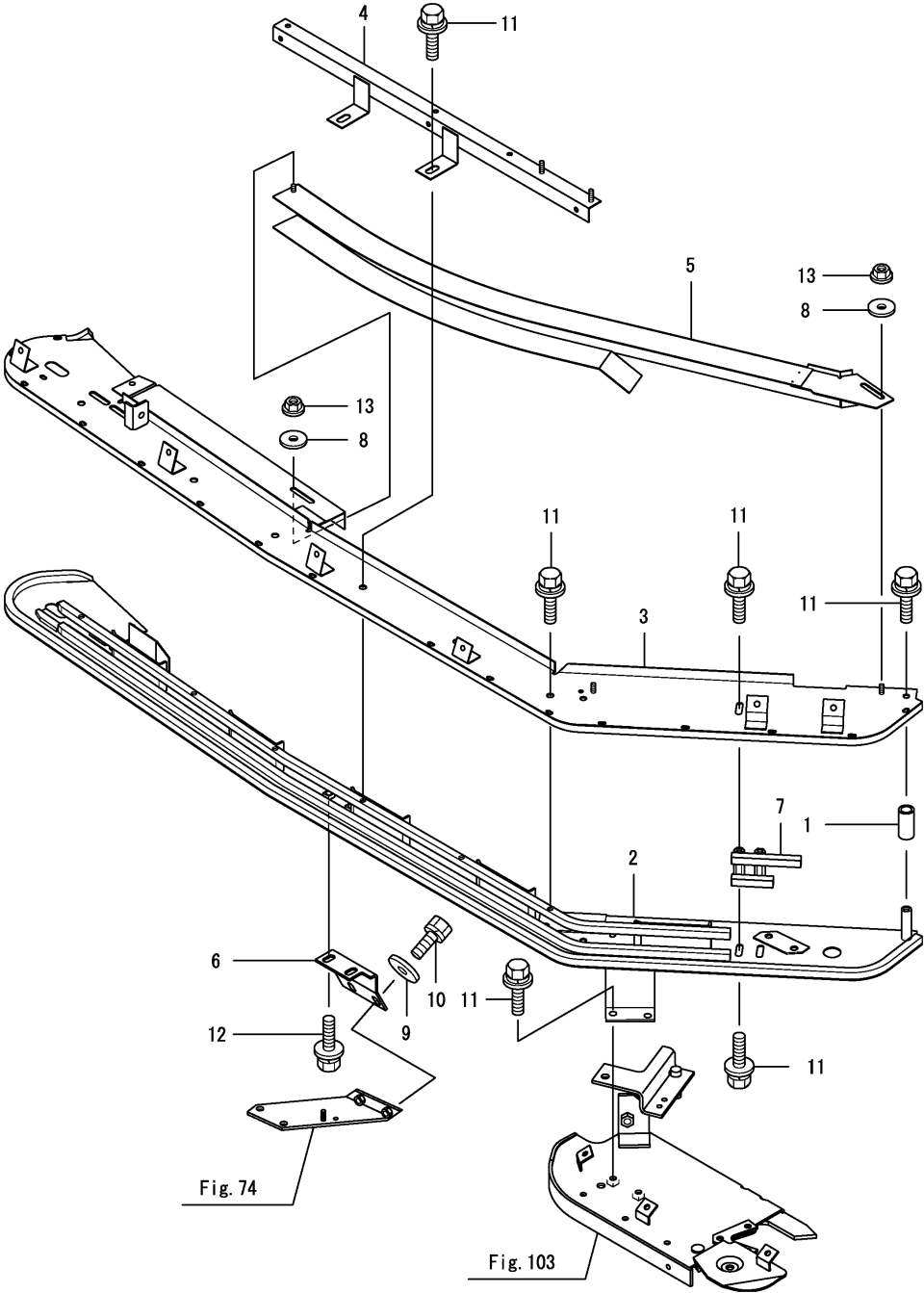
Fig.80. 상단 이송 케이스(오른쪽)
