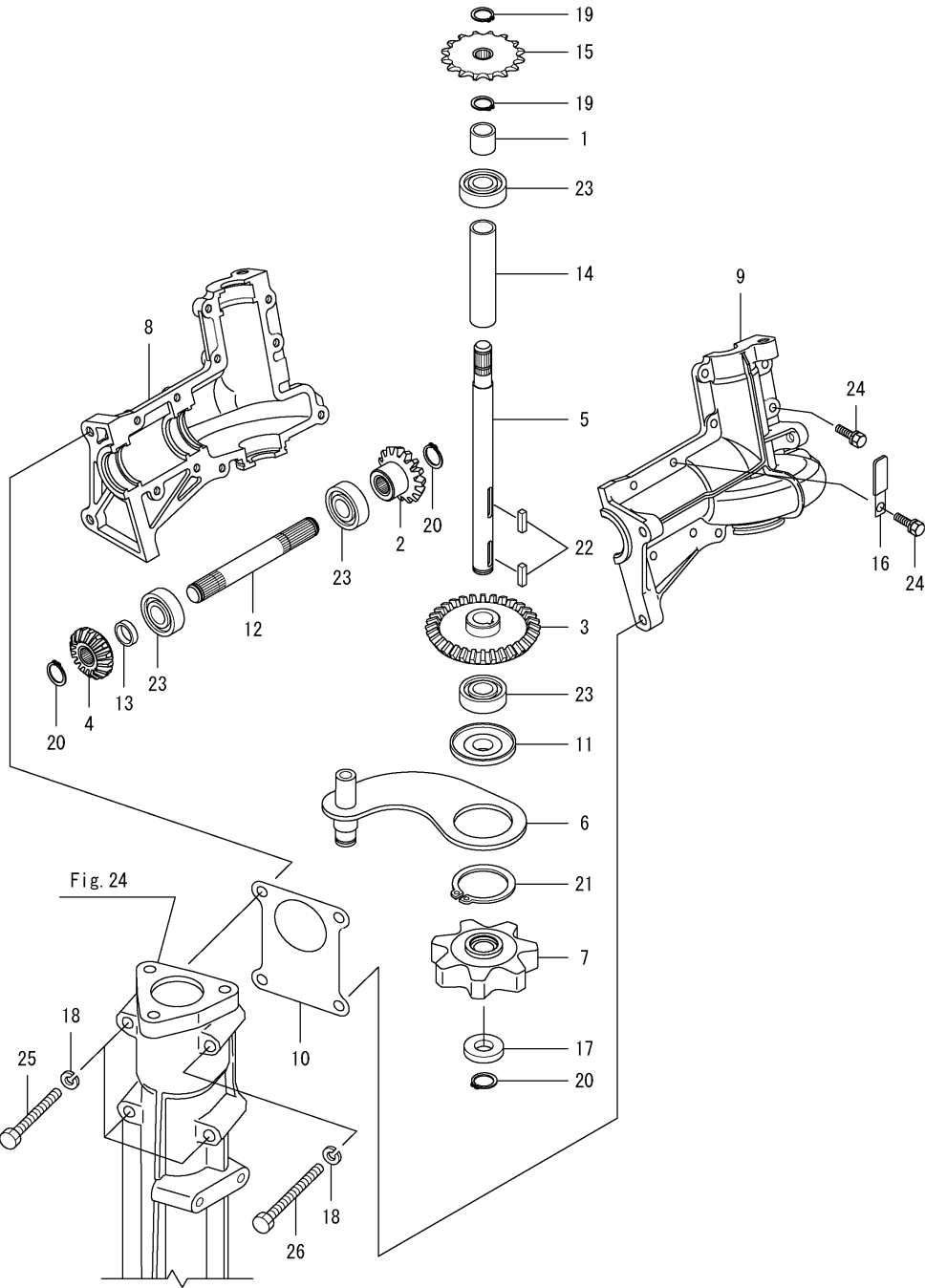
0CNP5-M34400 수확(2) Fig.69. 하단 이송 케이스(왼쪽)
