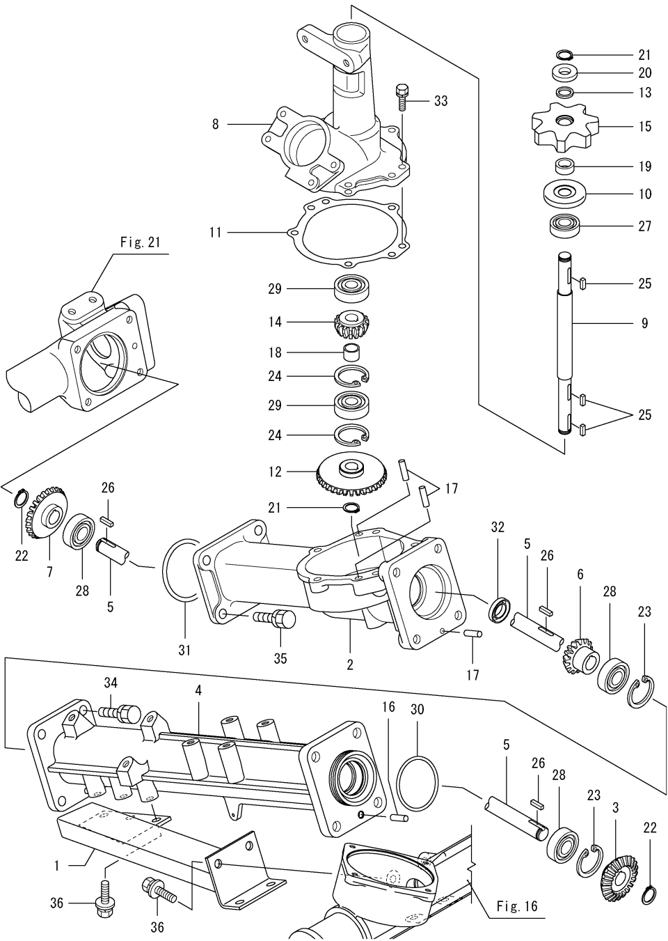
Fig.18. 축 케이스(2차)
