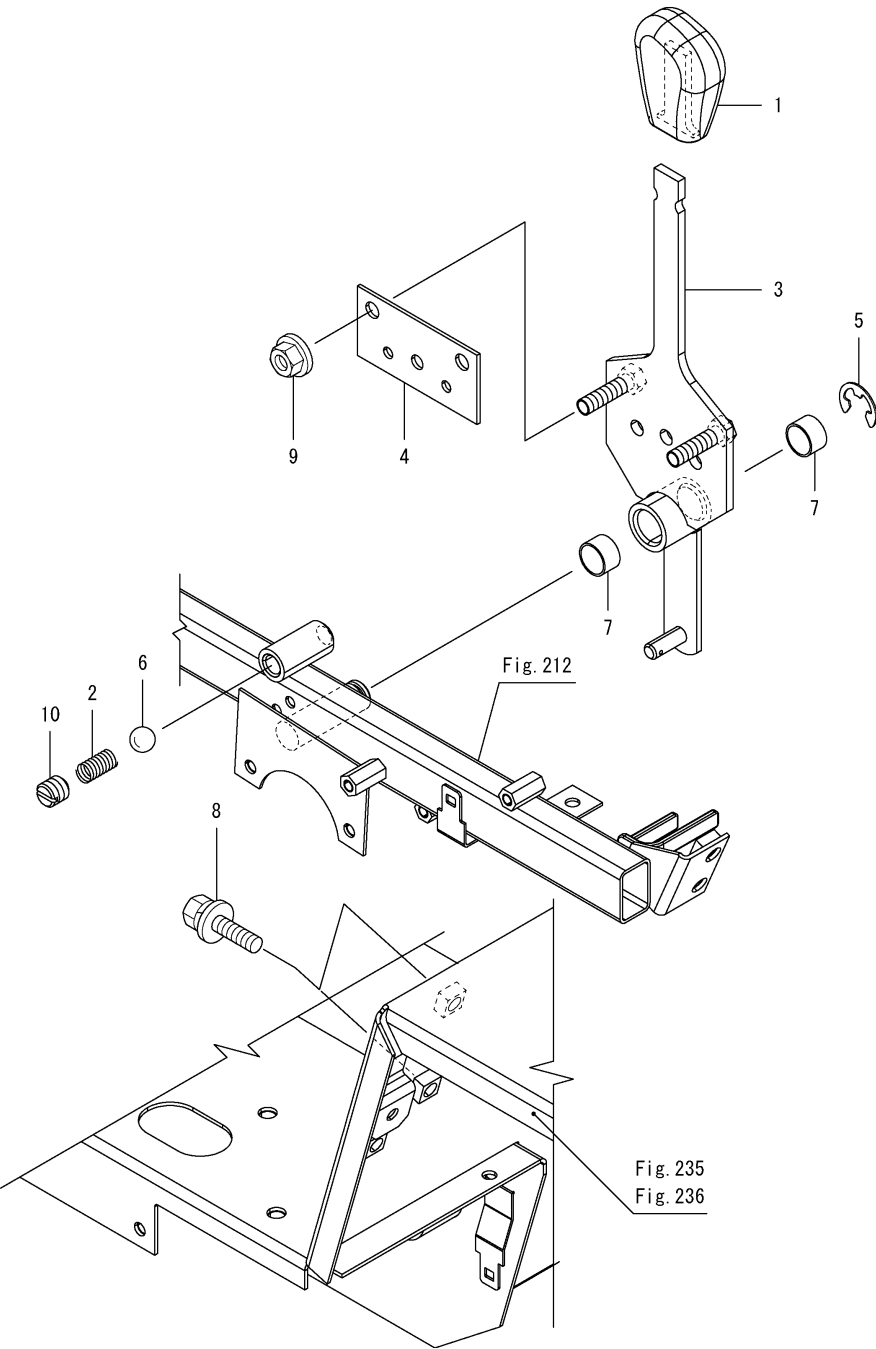
Fig.222. 클러치조작(탈곡)
