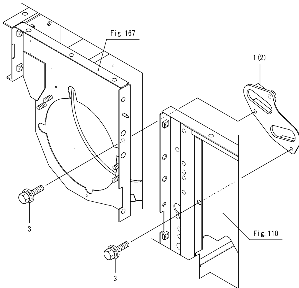
Fig.158. 스윙 암(전면)
