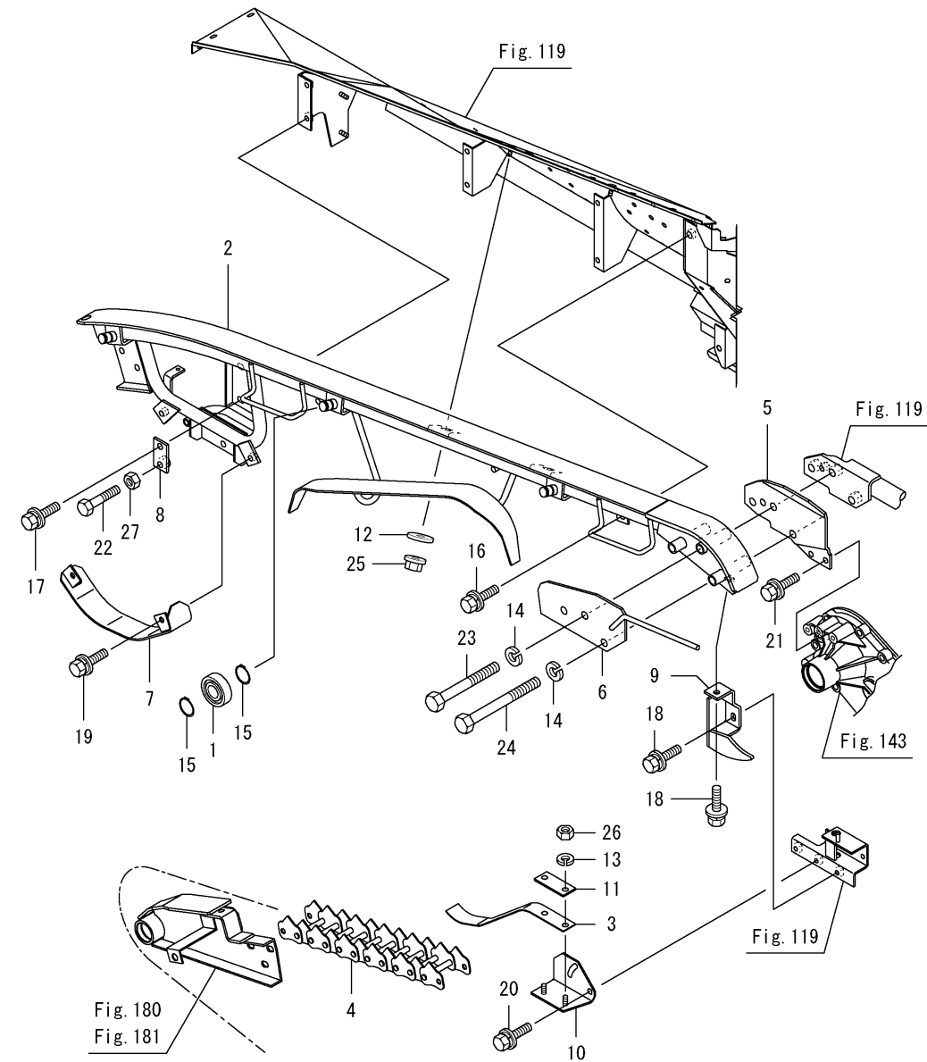
OCNP5-M34400 탈곡(2) Fig.179. 공급 체인(1)
