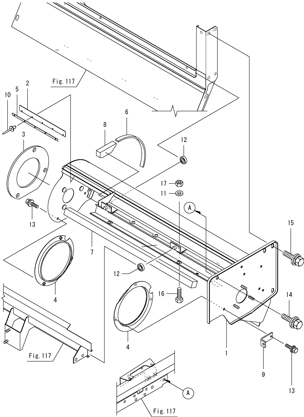
Fig.155. 처리 드럼 커버
