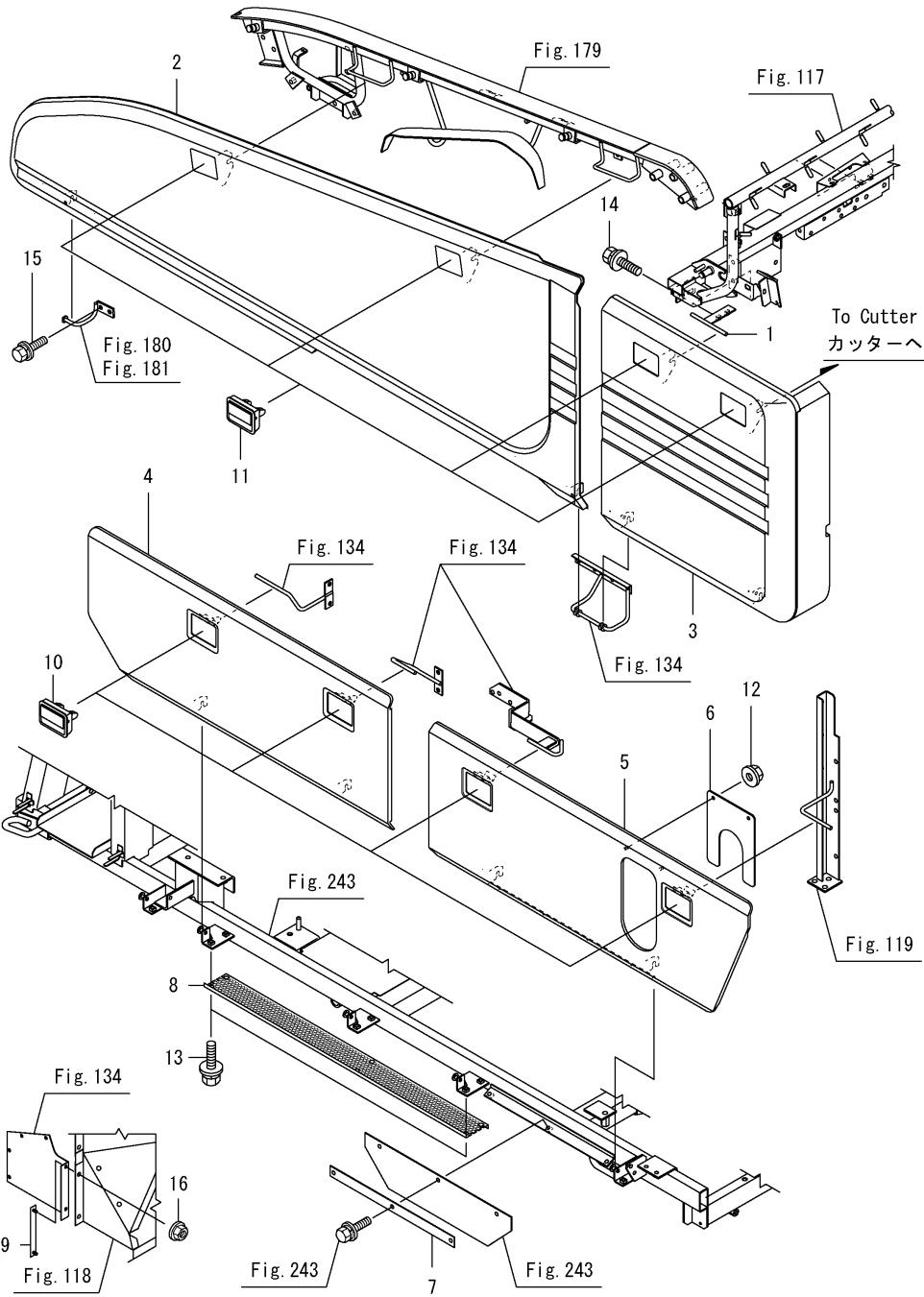
Fig.133. 측면 커버(왼쪽)(1)
