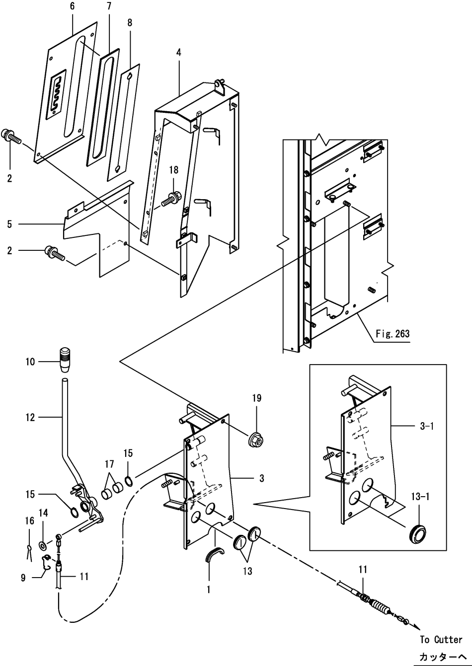
Fig.215. 스위칭 조작(캐빈)
