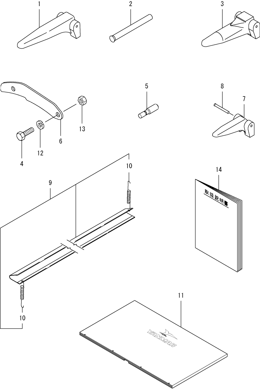
Fig.355. 부대품
