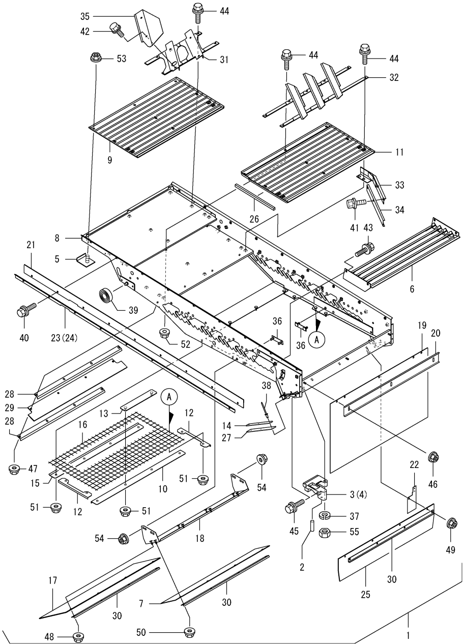
Fig.160. 요동선별판(1)
