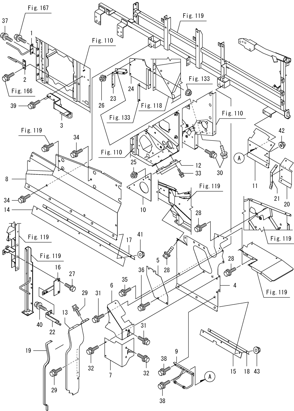
Fig.134. 측면 커버(왼쪽)(2)
