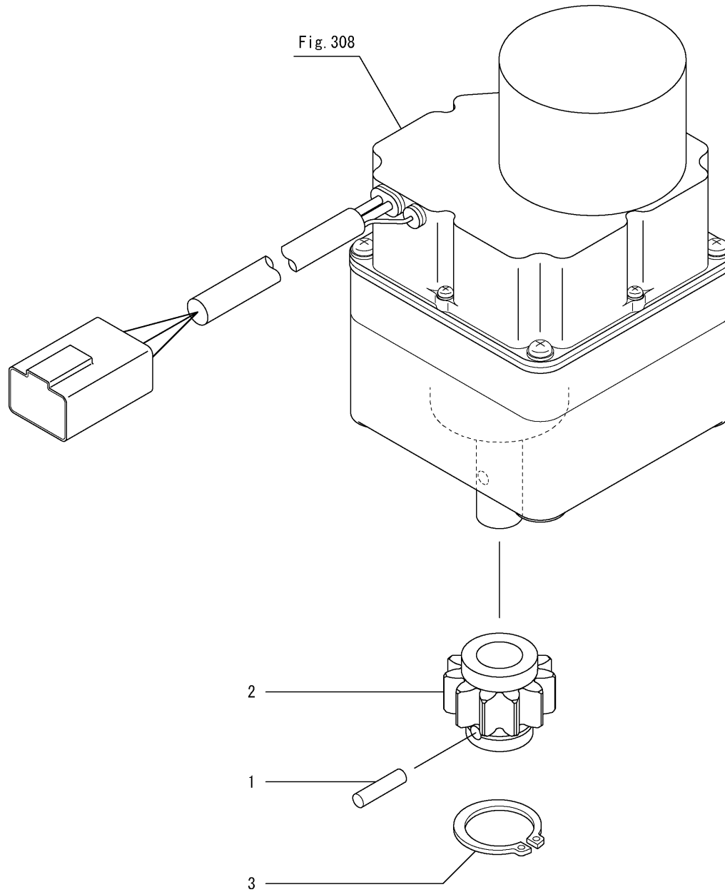
Fig.335. 오거제어(회동)
