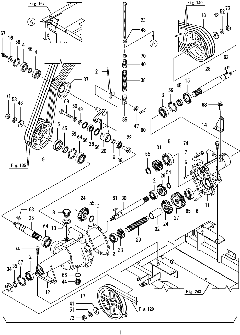
Fig.141. 탈곡입력케이스
