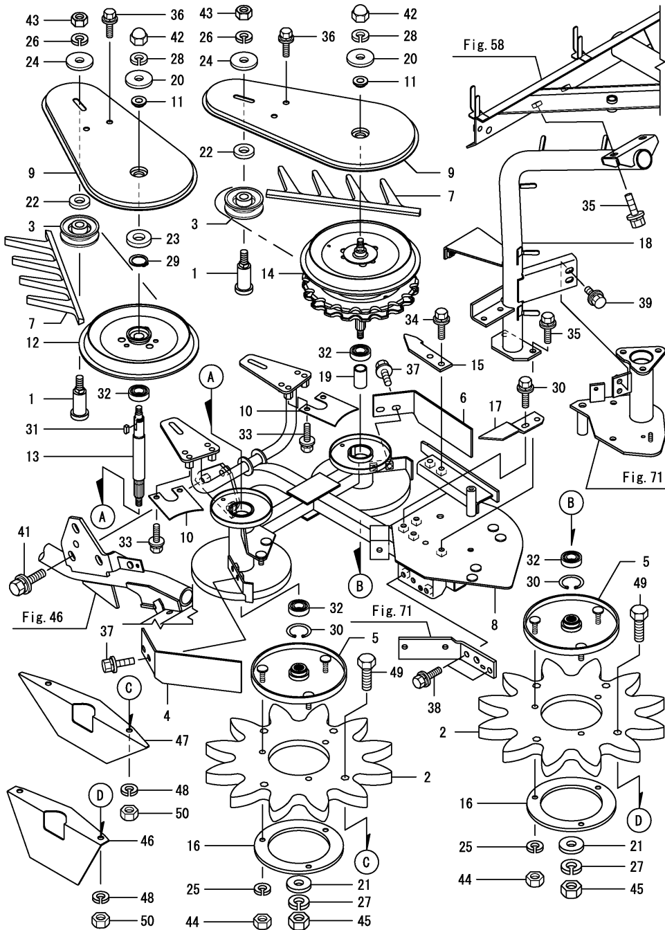
Fig.68. 끌어모음벨트(중-좌)
