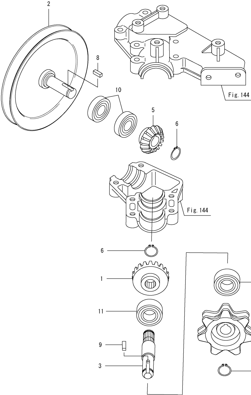
Fig.147. 짚 방출 드라이브 축
