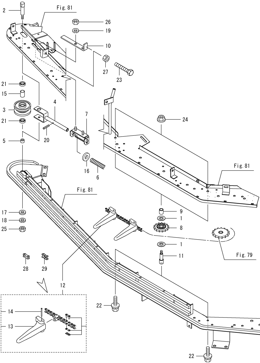
Fig.83. 상반송롤러(우-후)
