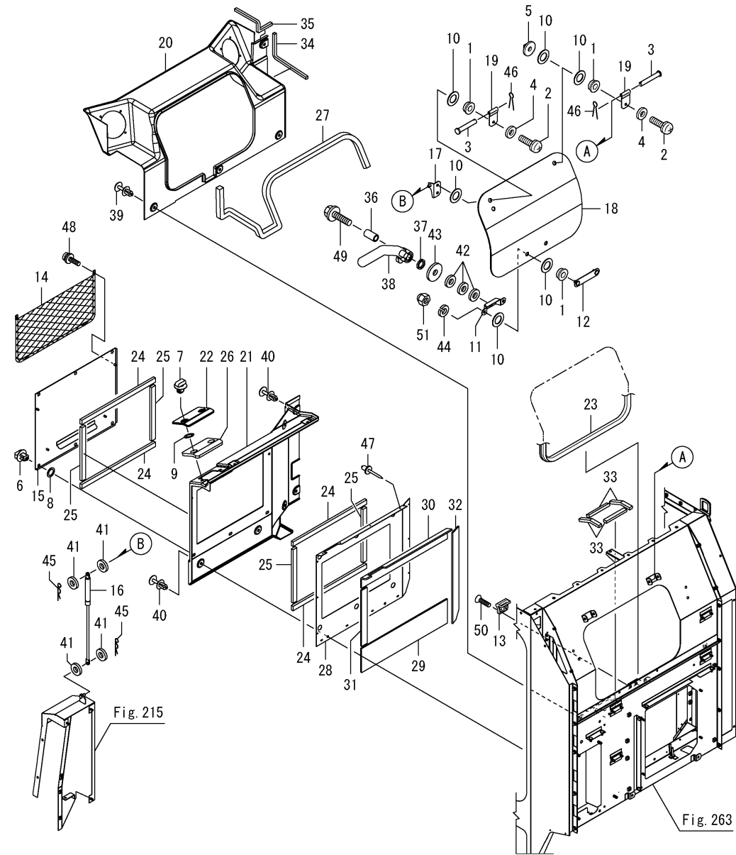
Fig.265. 캐빈 삭구(후면)
