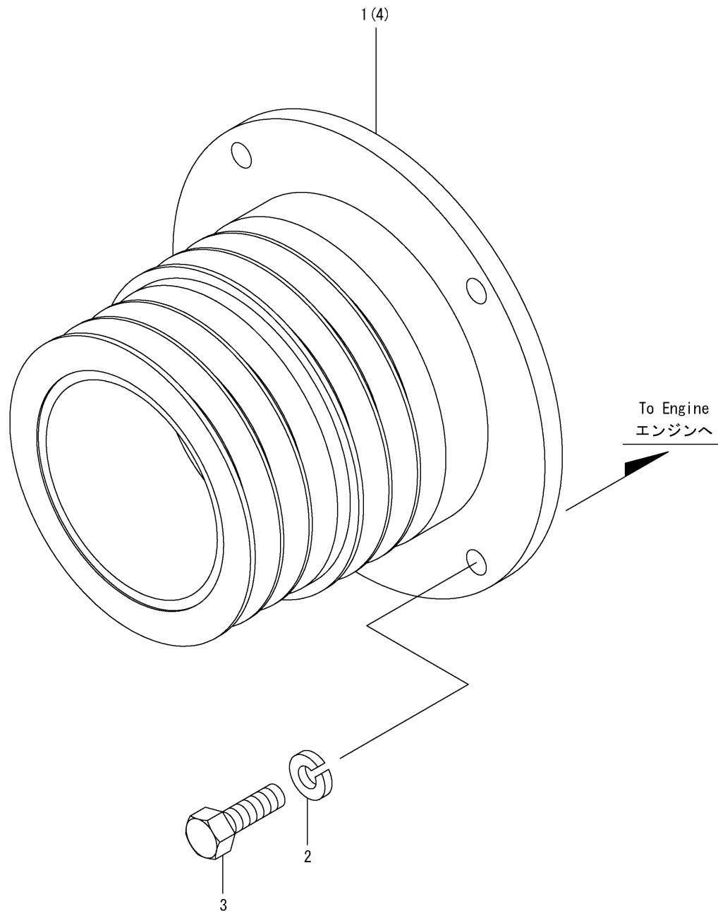
Fig.2. 엔진풀리
