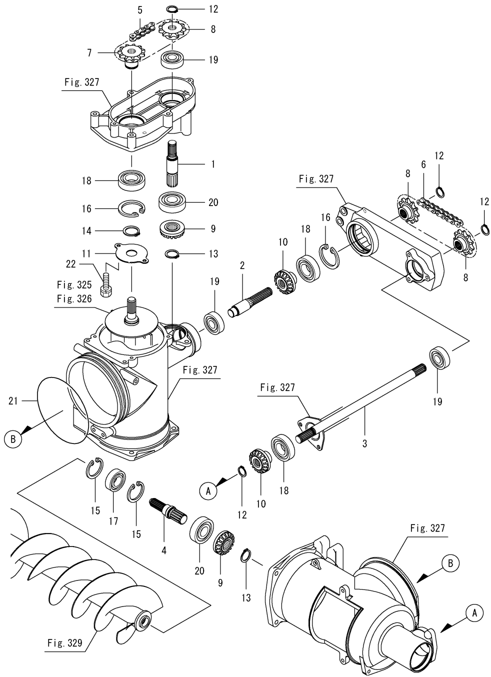
Fig.328. 오거연결케이스(2)
