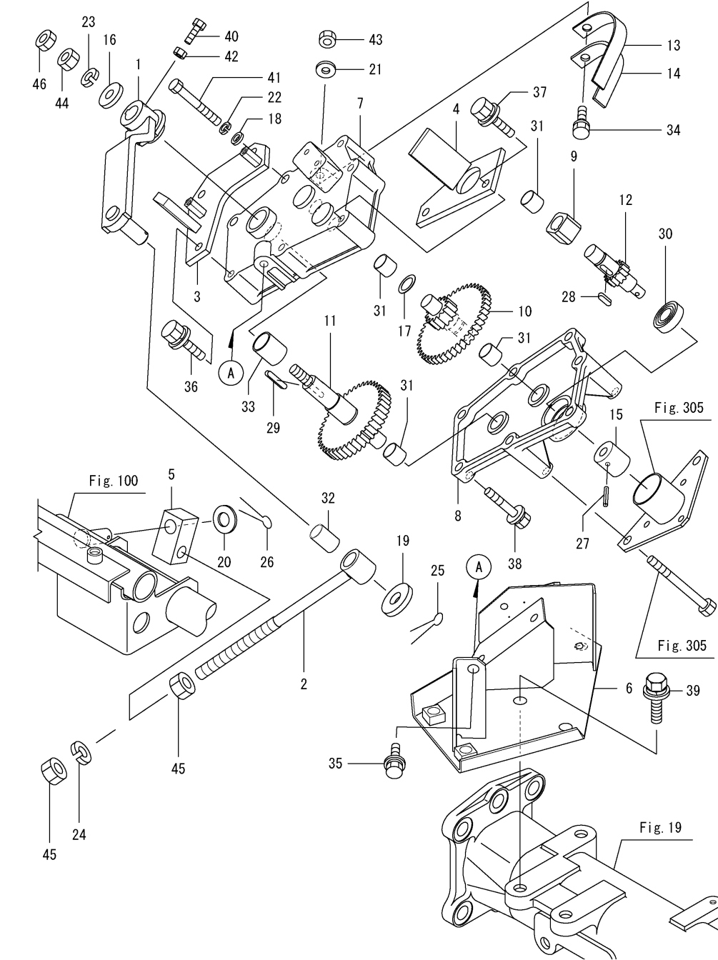
Fig.109. 탈곡깊이조절
