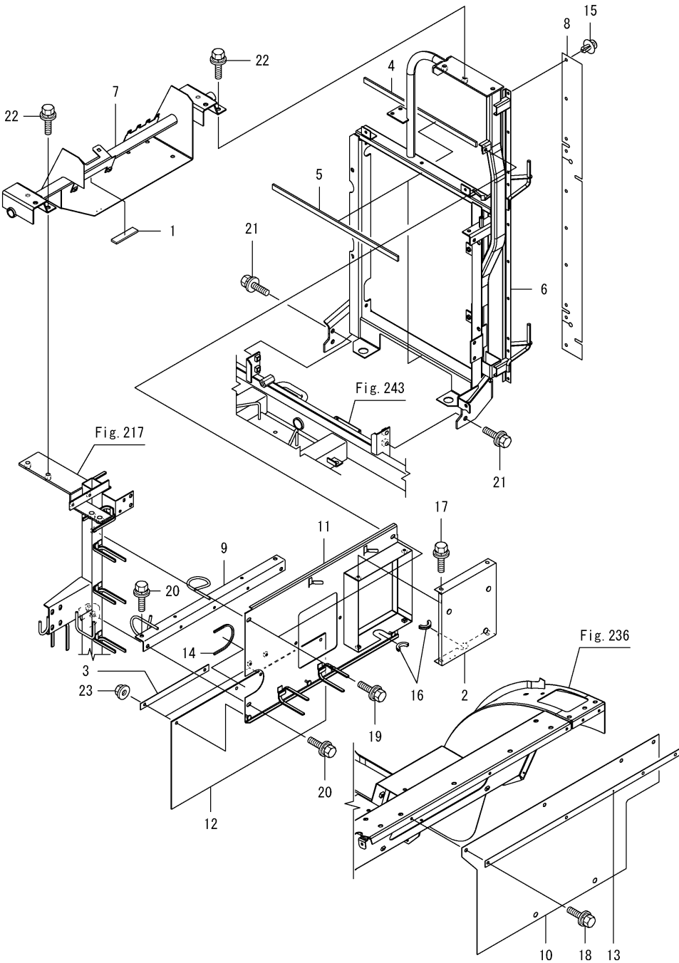
Fig.257. 엔진실프레임(캐빈)
