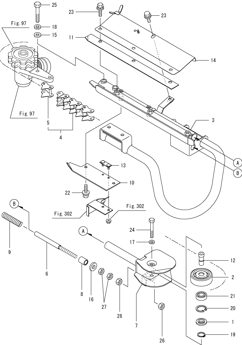
Fig.99. 수직 체인 케이스
