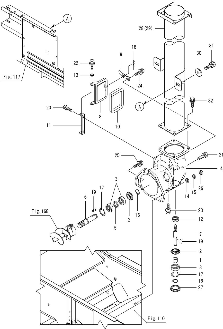
Fig.169. 양곡컨베이어케이스
