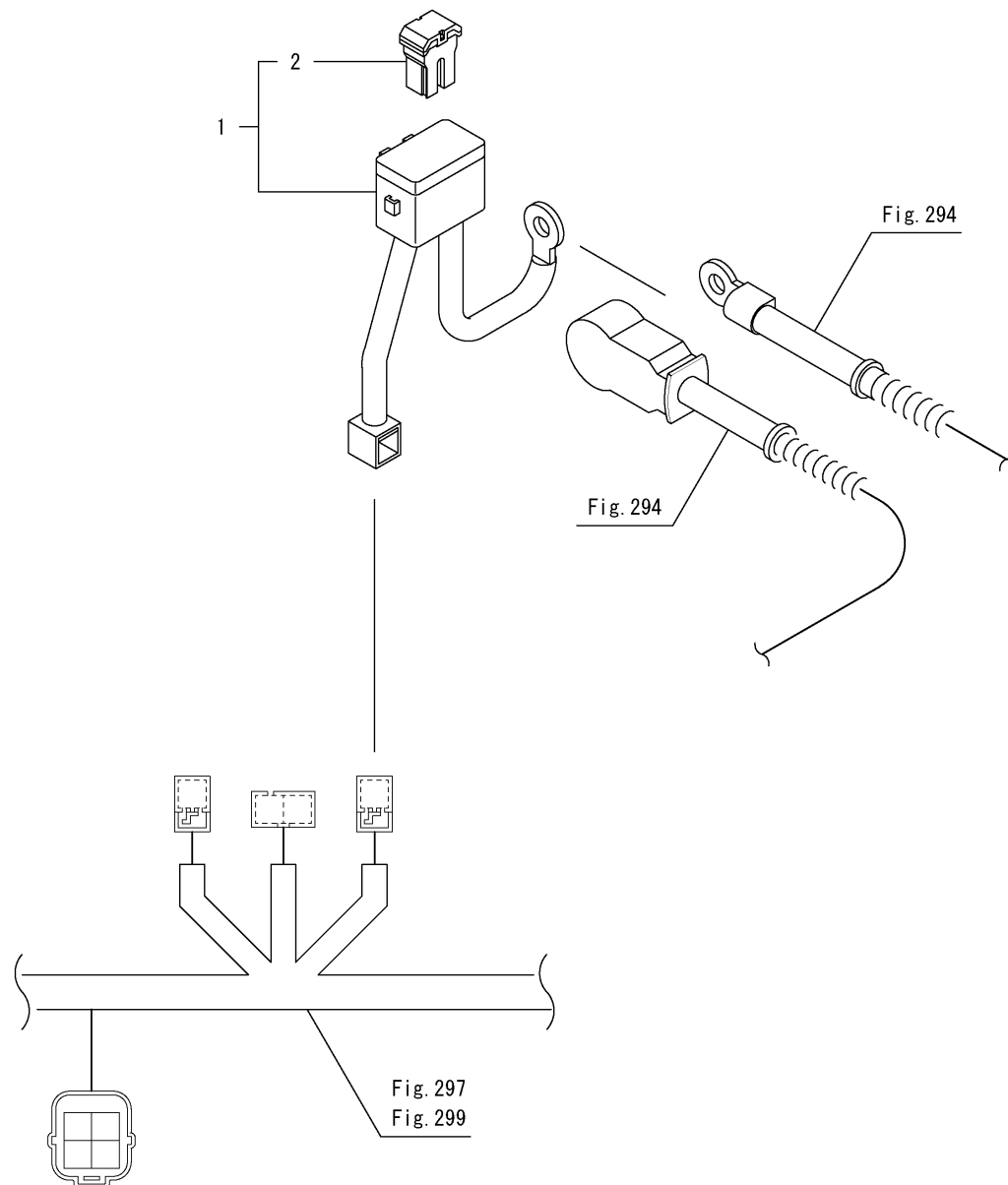
Fig.295. 캐빈(전력 공급)
