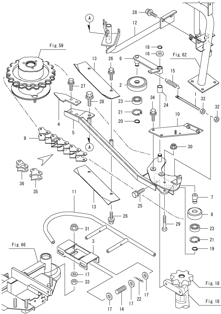
Fig.74. 하단 이송 가이드(오른쪽)
