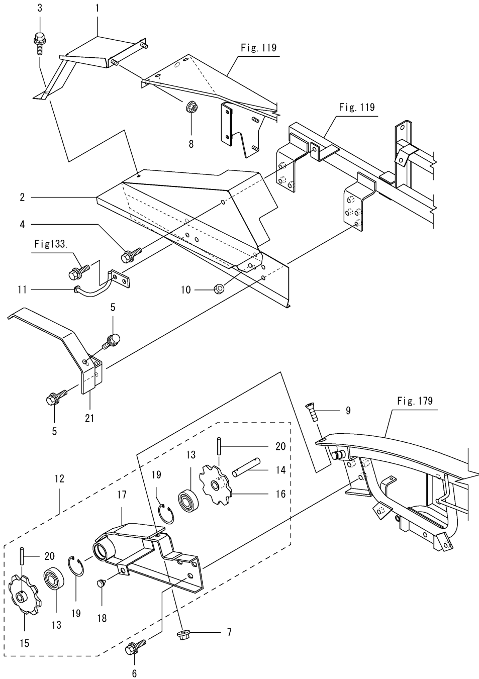
Fig.180. 공급 체인(2)
