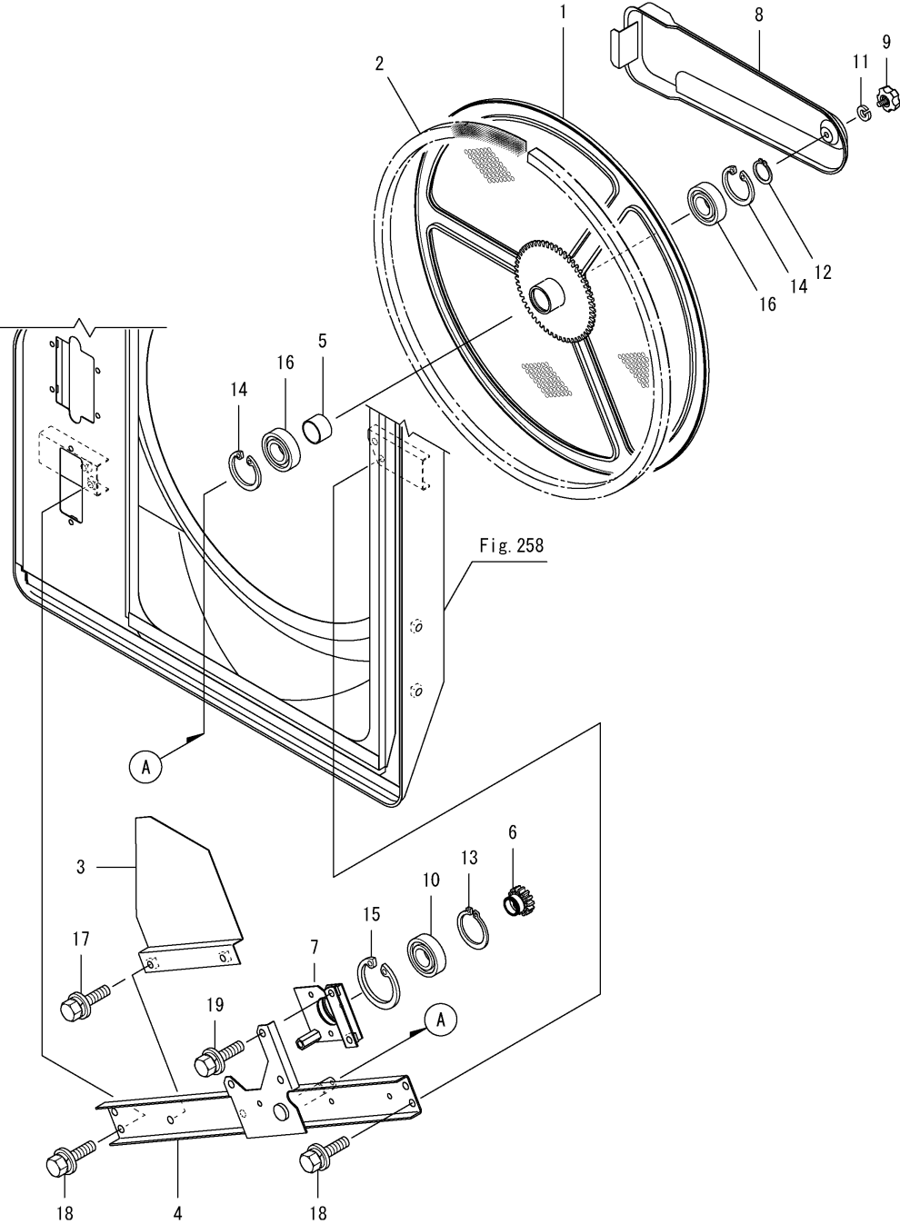
Fig.14. 회전 스크린
