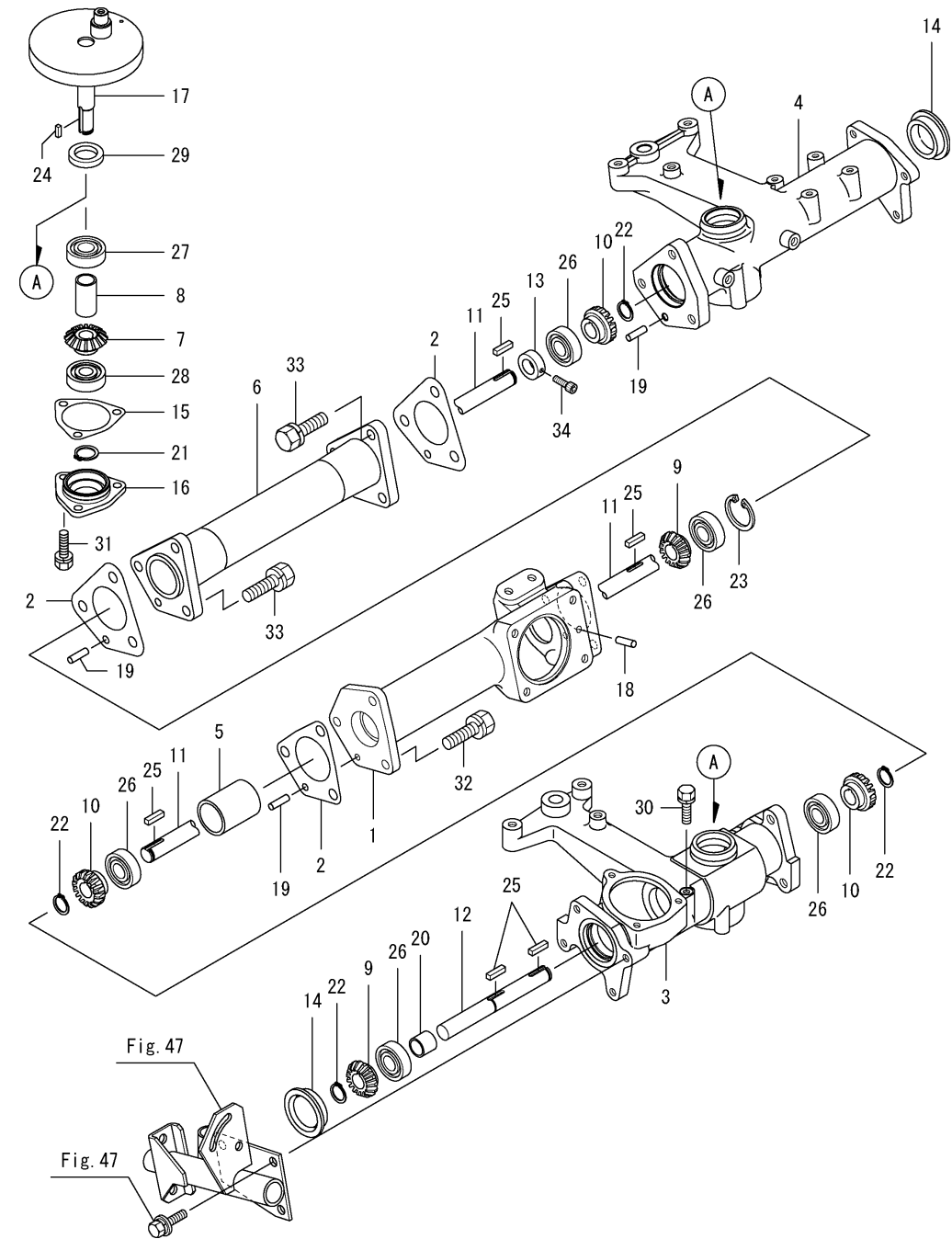
OCNP5-M34400 수확(1) Fig.21. 하단 케이스
