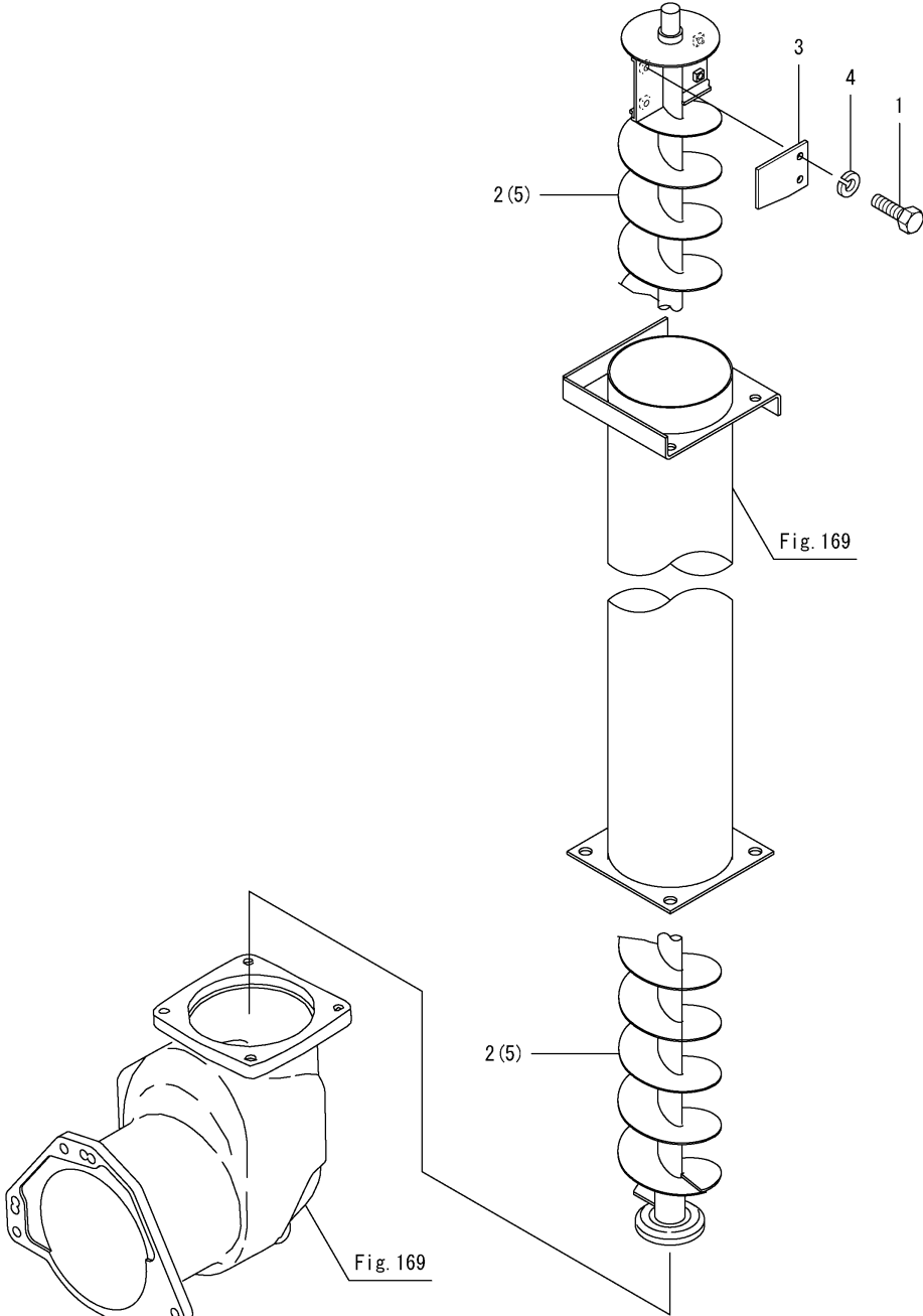
Fig.170. 곡물 상승 오거
