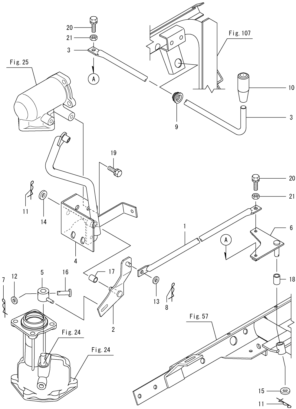
Fig.27. 인기변속
