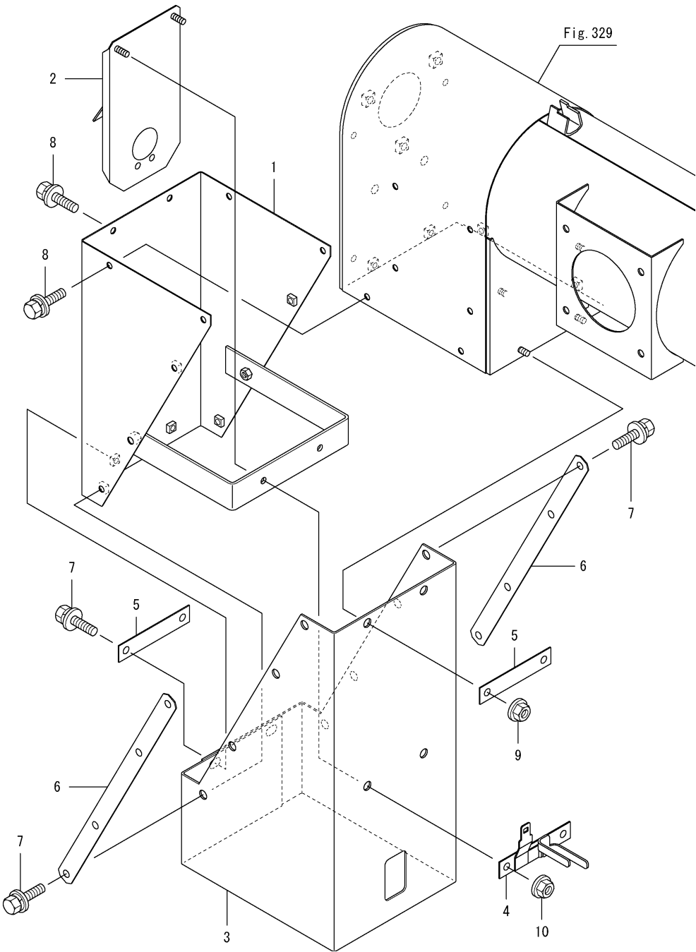
Fig.330. 오거배출구
