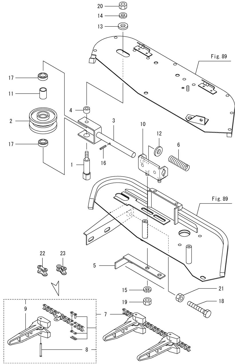
Fig.90. 상반송롤러(중)
