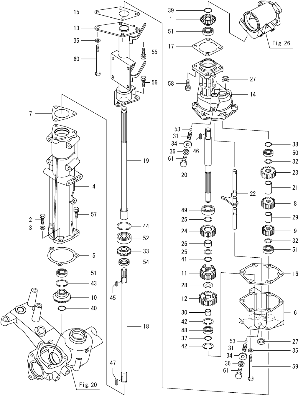
Fig.23. 픽업 수직 드라이브
