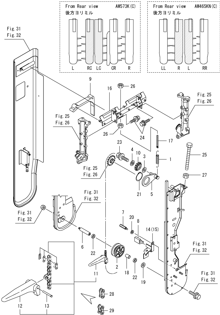
Fig.35. 인기체인롤러(중)
