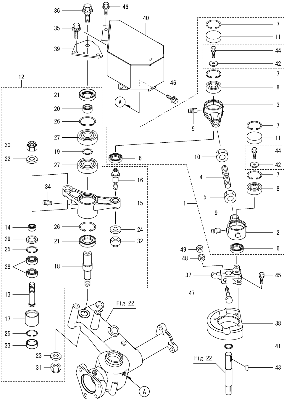
Fig.50. 예취날구동(우)
