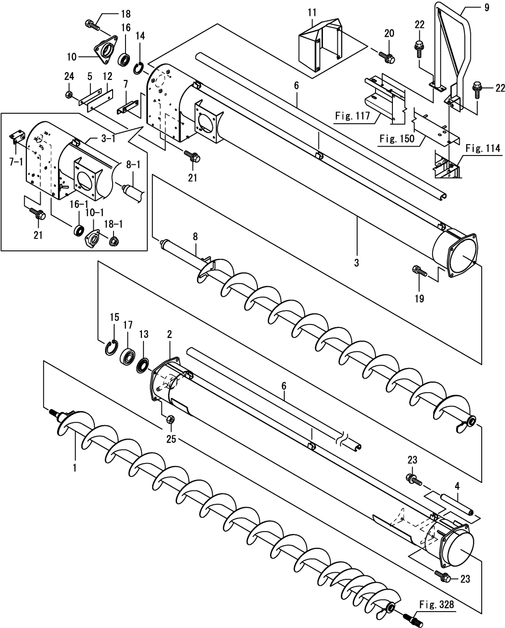
Fig.329. 오거(측면)
