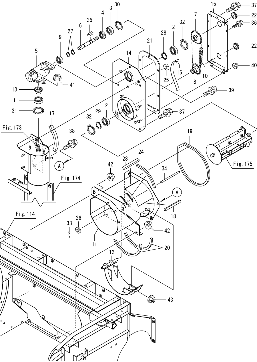
Fig.176. 처리 드럼 케이스(2차)
