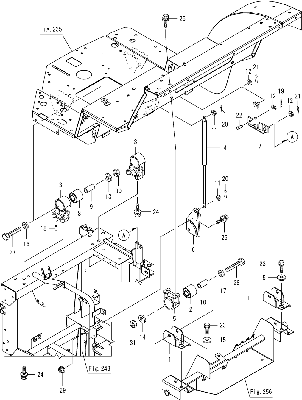
Fig.231. 발판방진
