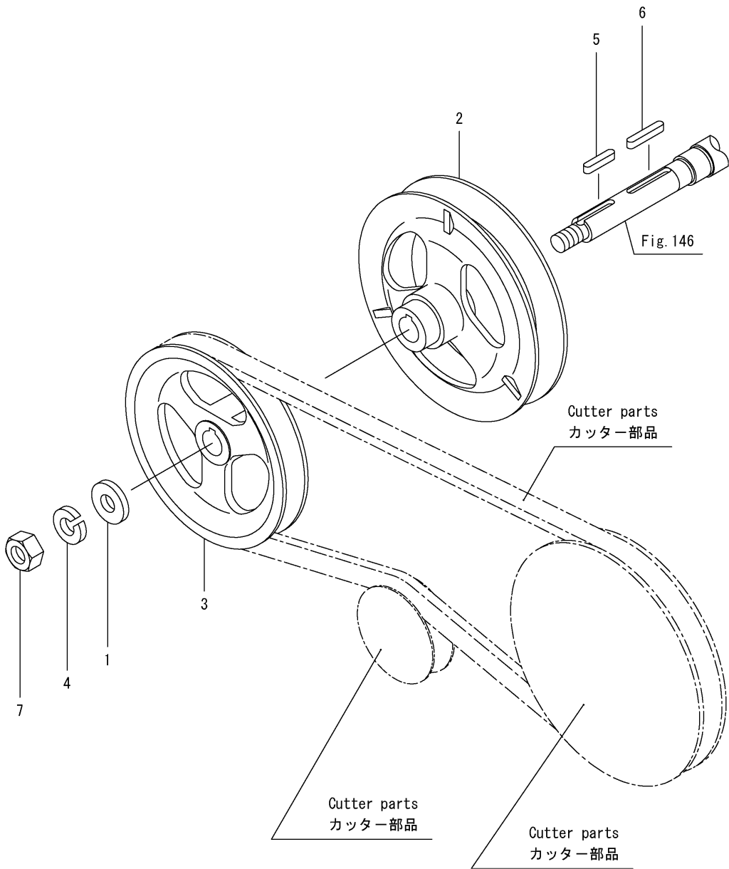
Fig.132. 흡입 벨트
