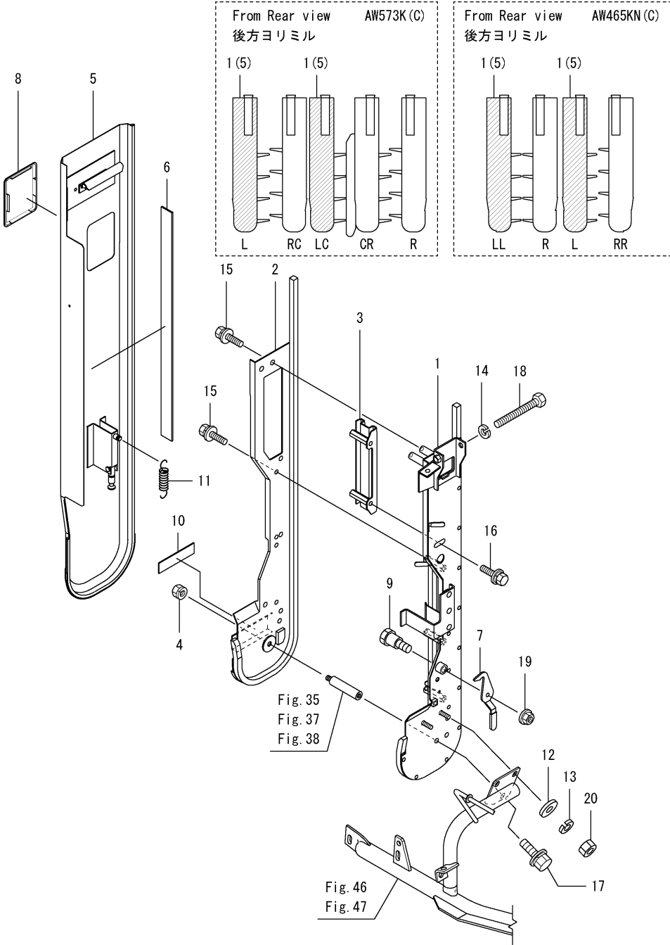
Fig.31. 픽업 케이스(왼쪽)
