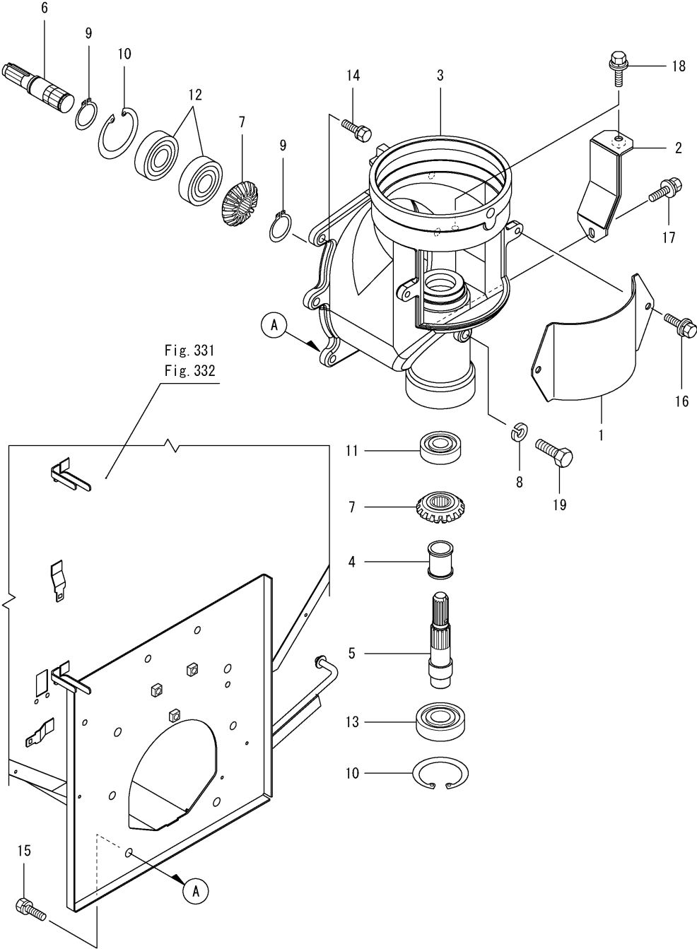
Fig.322. 하부컨베이어연결
