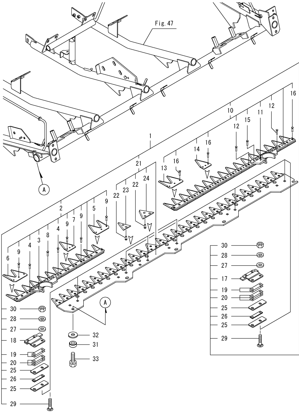
Fig.52. 예취날
