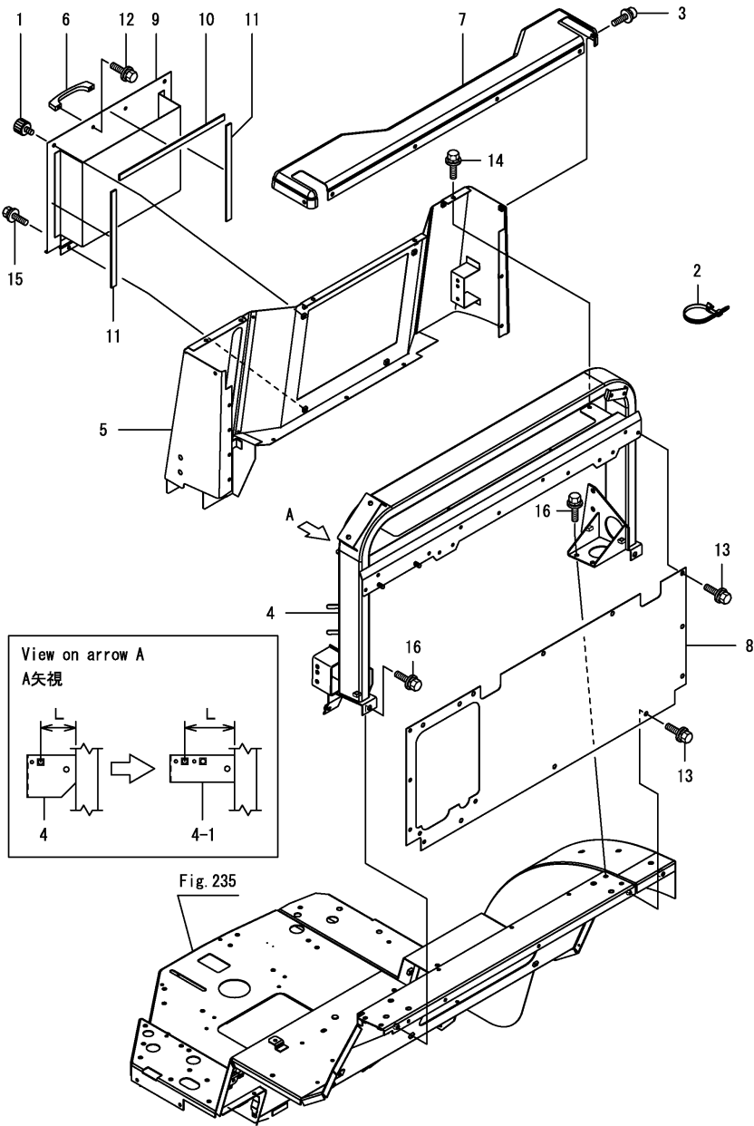
Fig.237. 후면 칼럼
