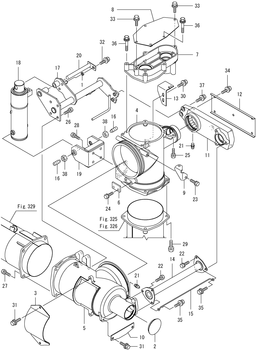
Fig.327. 오거연결케이스(1)
