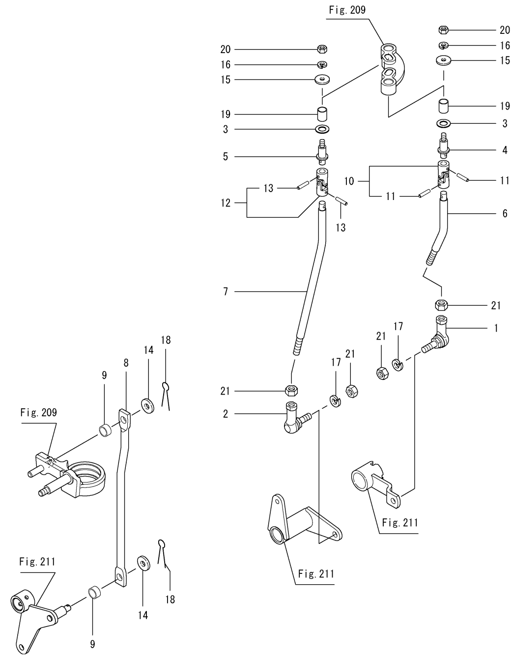
Fig.210. 스티어링 조작(2)
