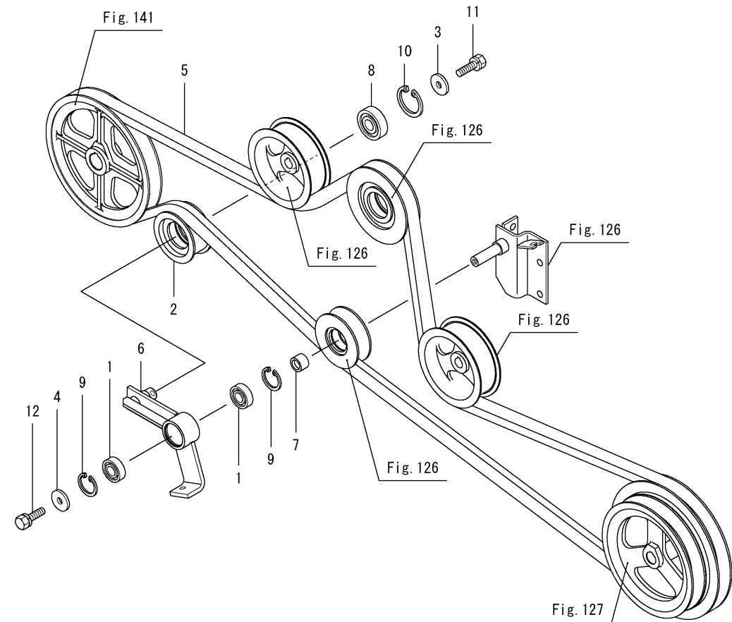
Fig.129. 카운터 벨트(2)
