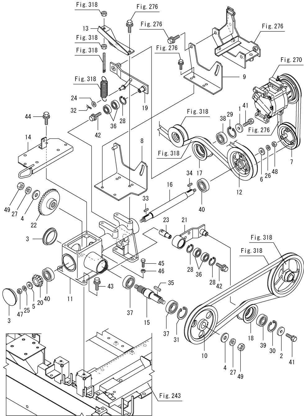
Fig.316. 입력케이스(곡물탱크)(캐빈)
