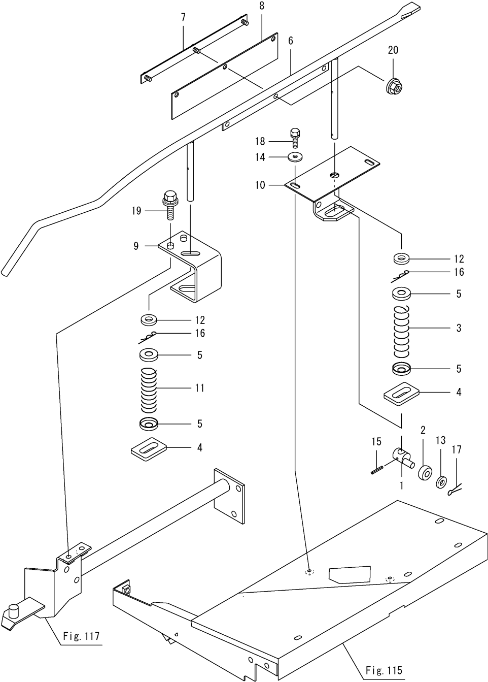
OCNP5-M34400 탈곡(2) Fig.187. 쥘배출잡이
