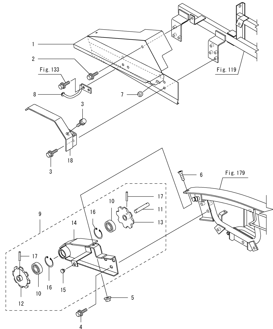
OCNP5-M34400 탈곡(2) Fig.181. 공급 체인(2)
