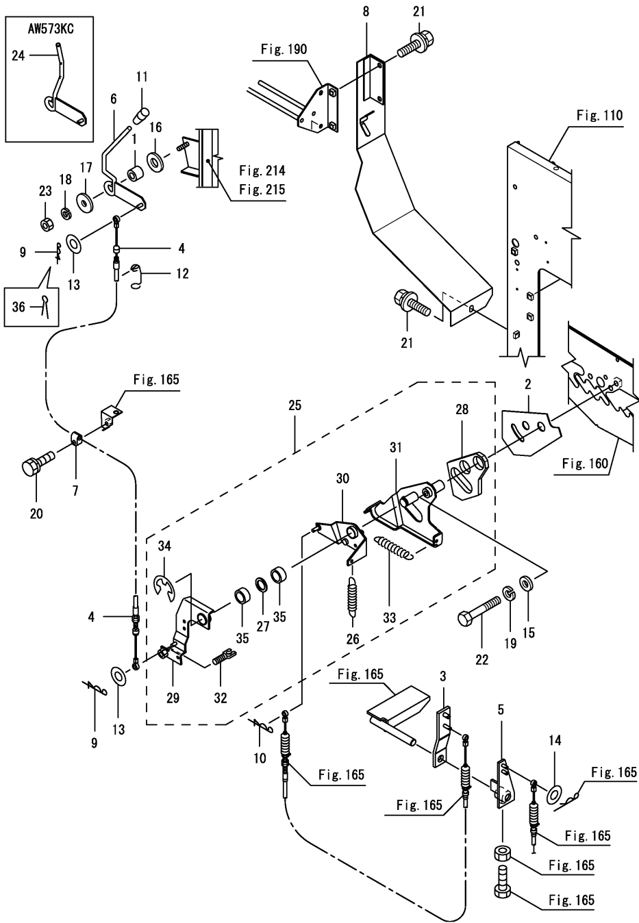
Fig.164. 요동선별조작(1)
