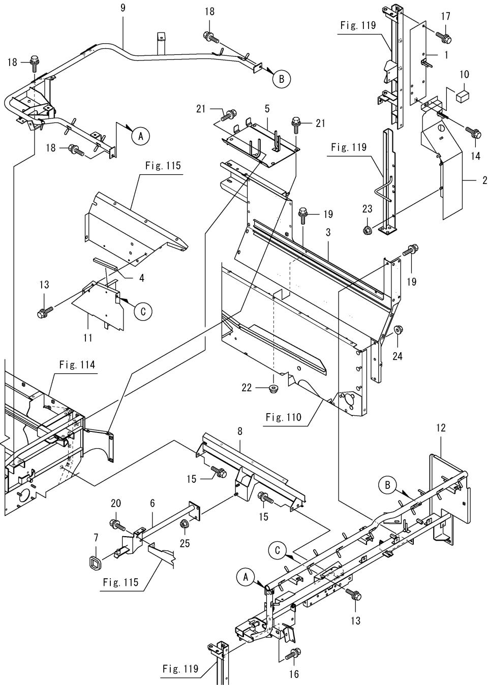
Fig.117. 상단 몸체(후면)(1)
