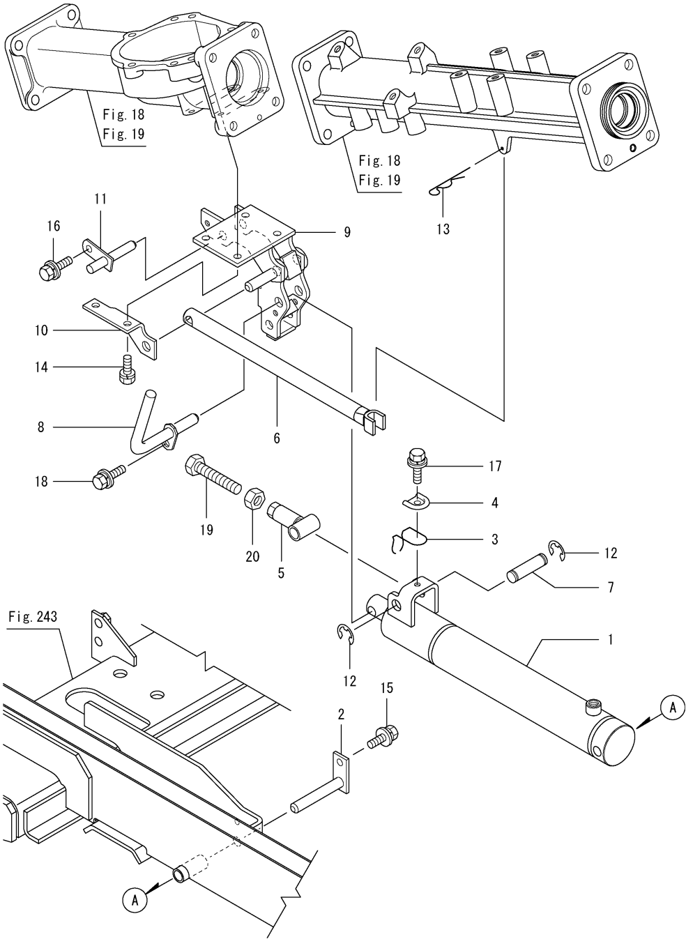
Fig.227. 상하유압실린더
