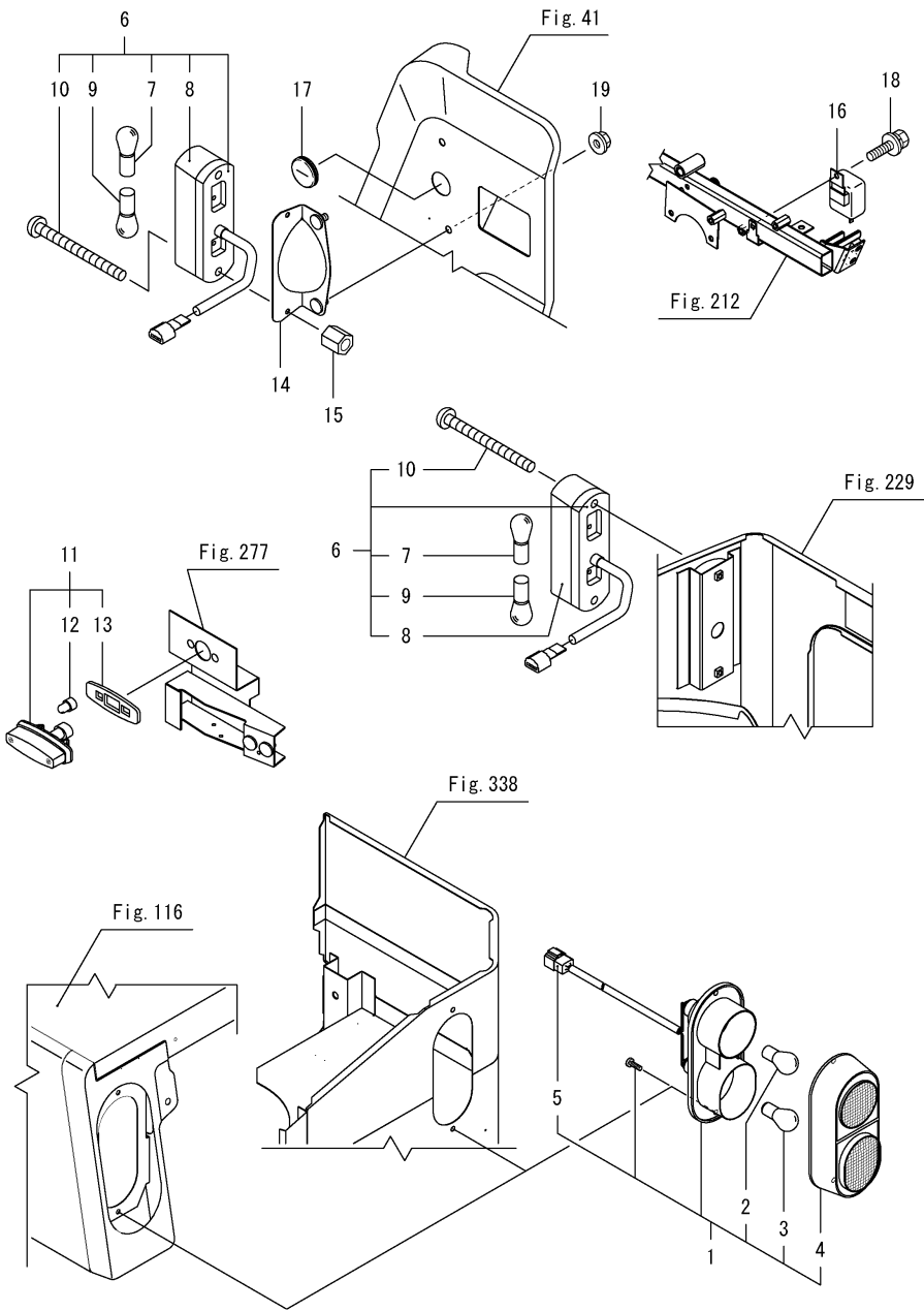
Fig.285. 방향지시등
