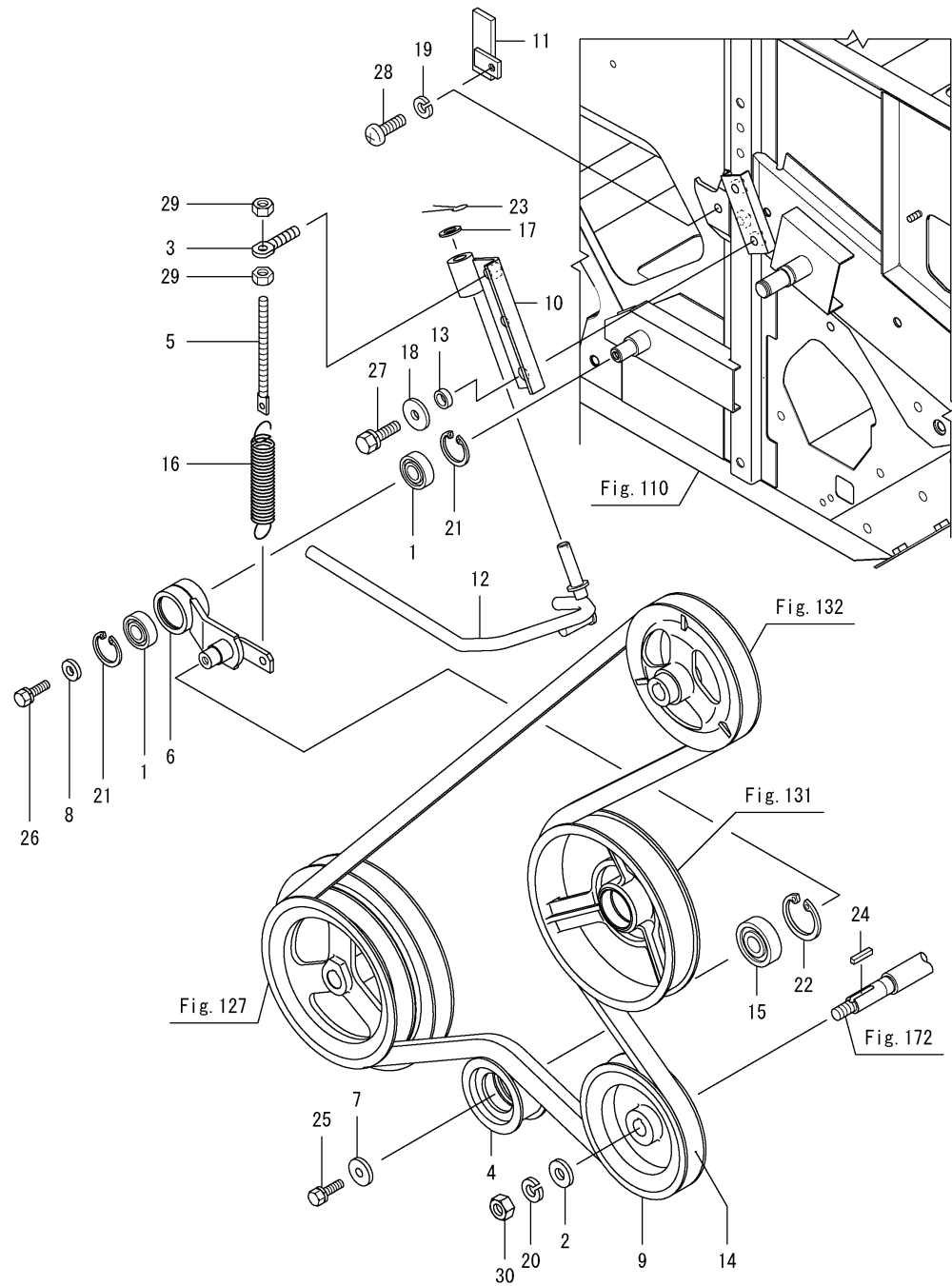
OCNP5-M34400 탈곡(1) Fig.130. 벨트(2차)
