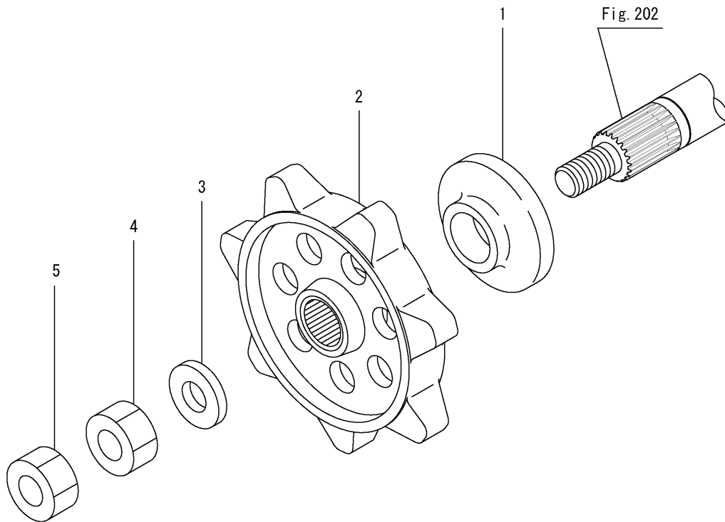
Fig.250. 스프로킷
