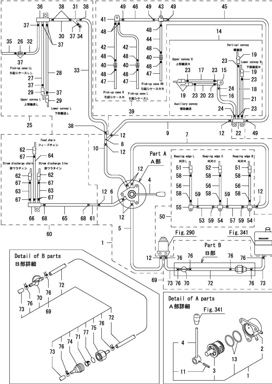
Fig.342. 주유장치(2)
