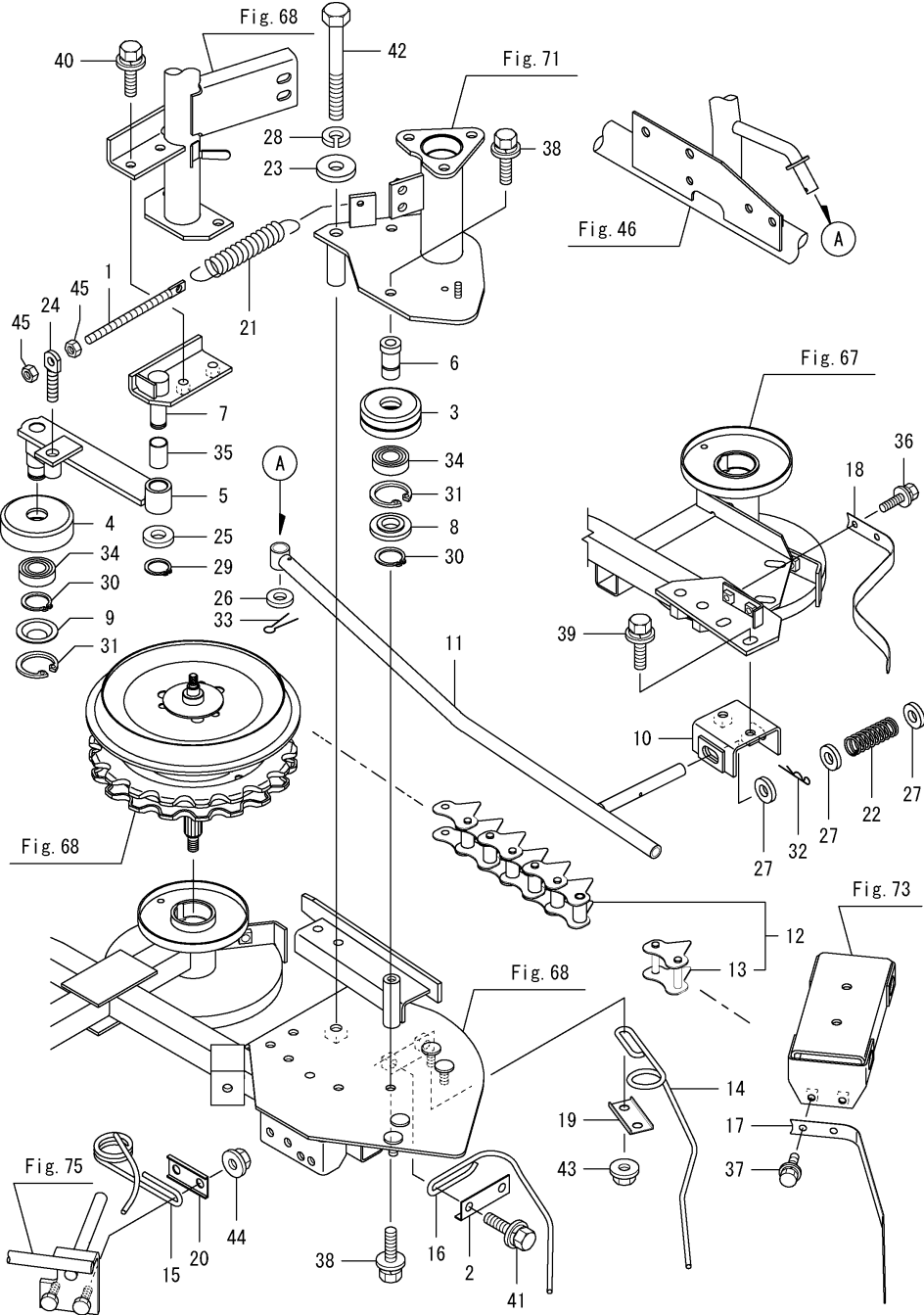
Fig.77. 하부반송가이드(중)
