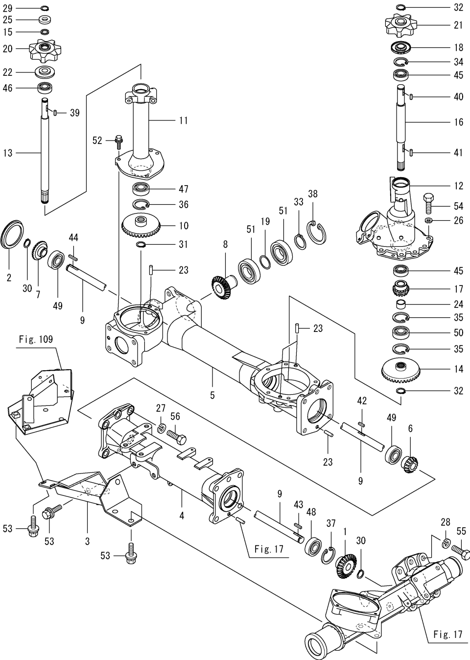
Fig.19. 축 케이스(2차)
