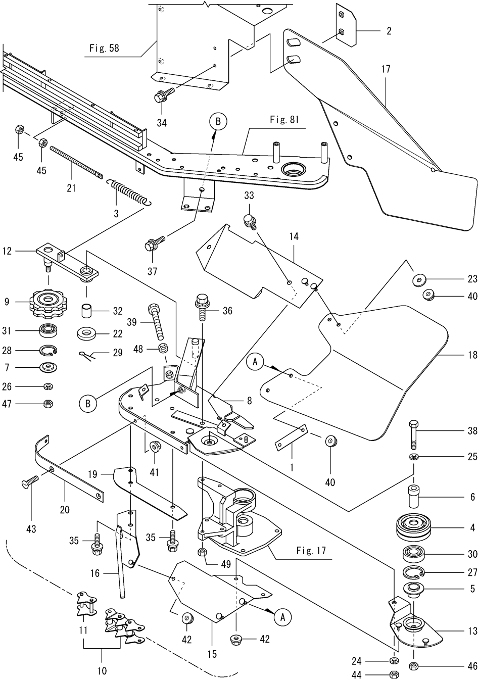
Fig.104. 보조반송
