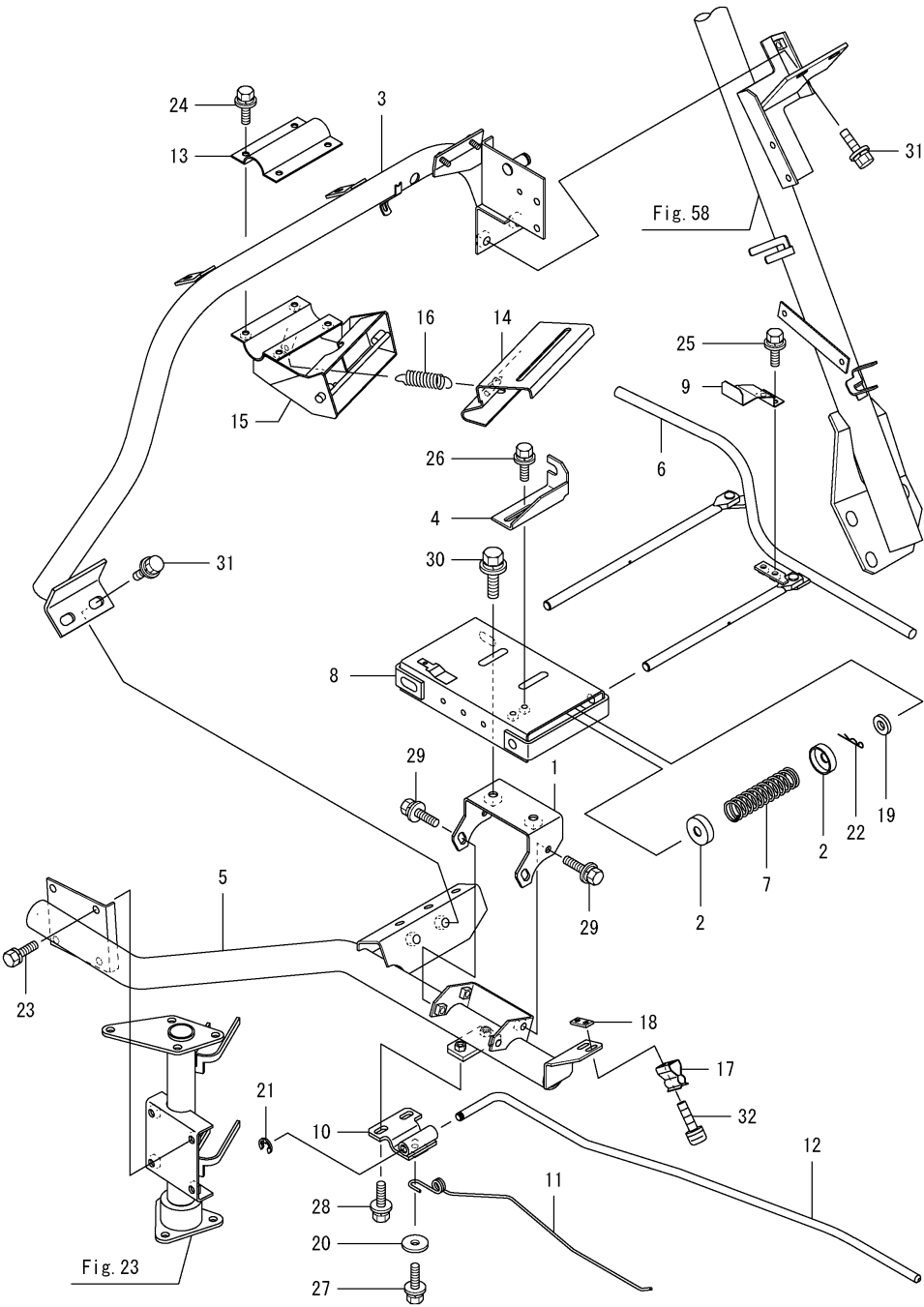
Fig.105. 보조반송가이드
