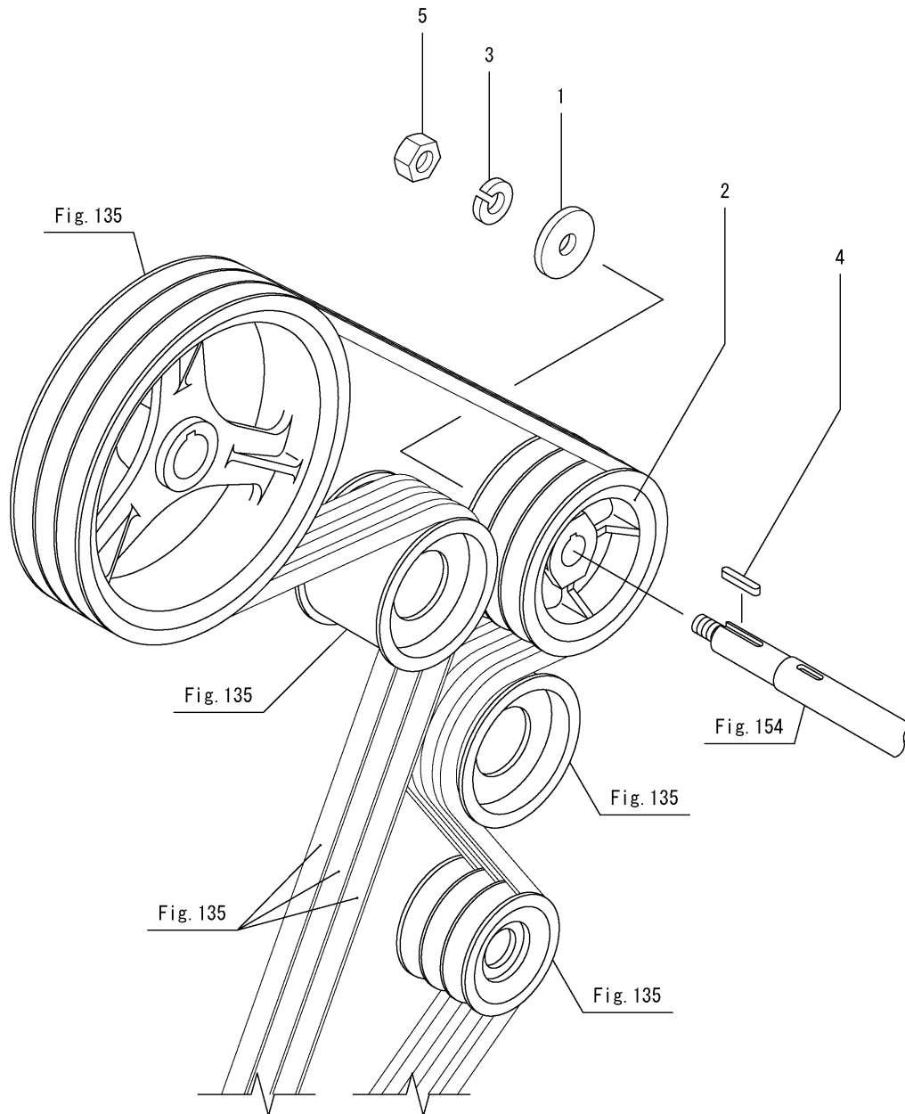
Fig.136. 처리 드럼 벨트
