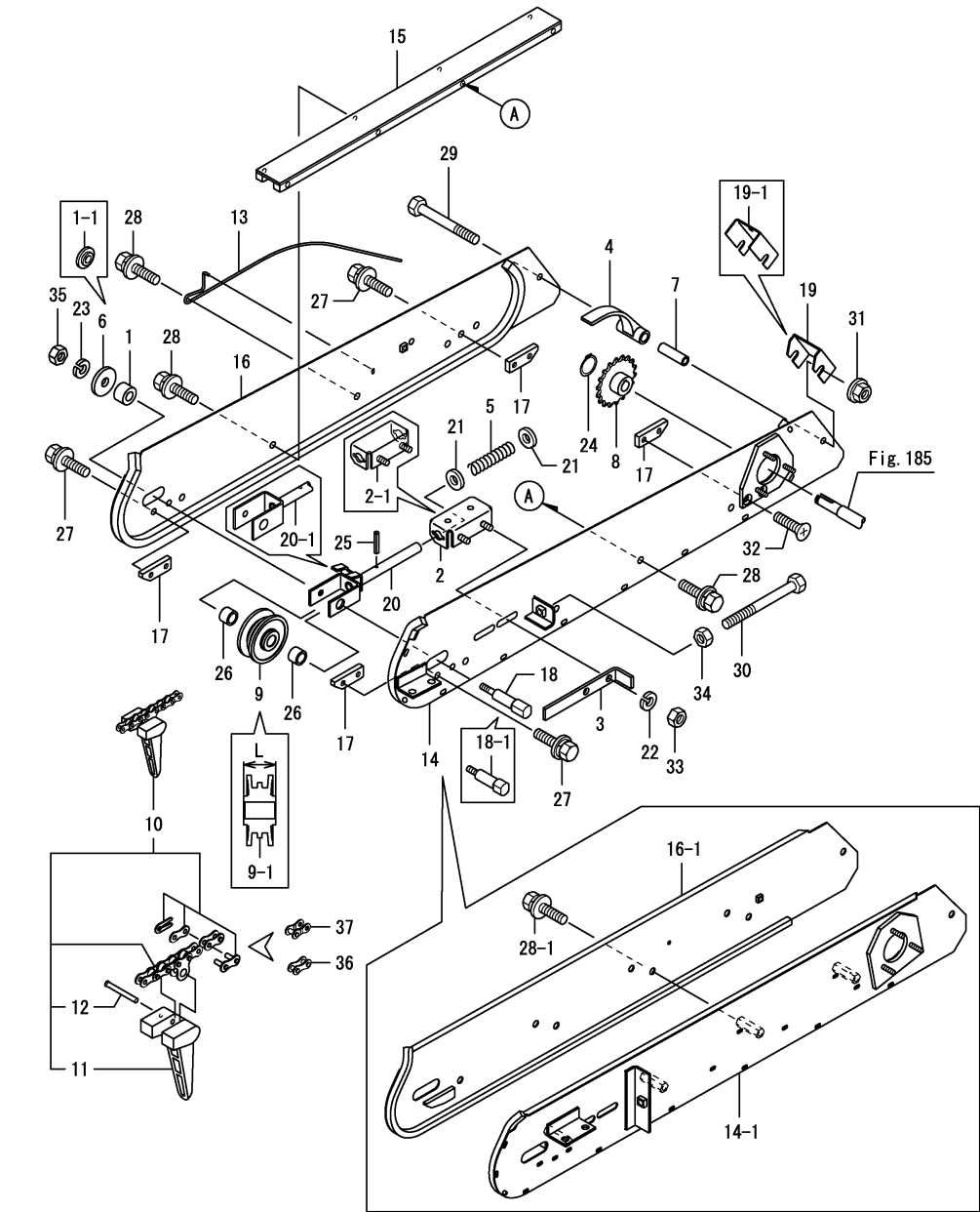
Fig.184. 쟁배출반송(1)
