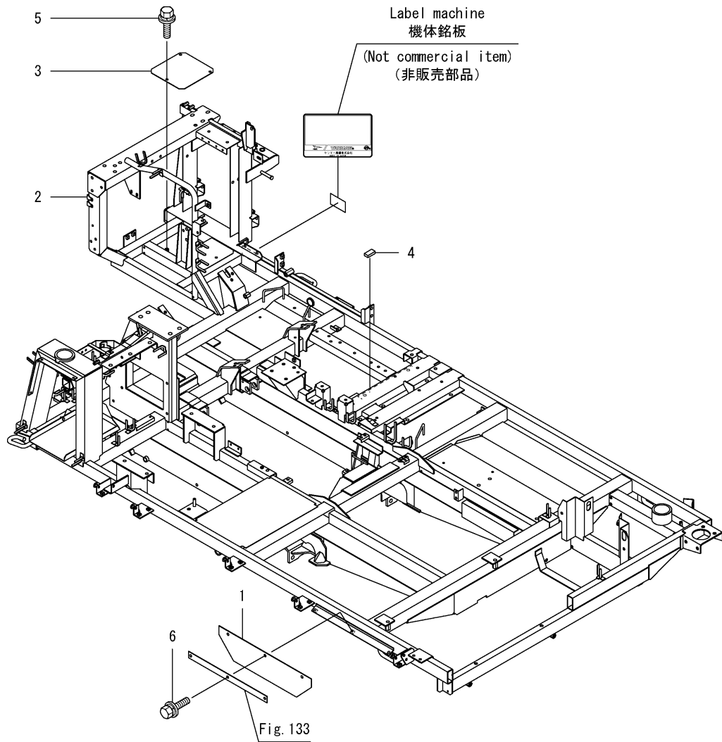
Fig.243. 새시프레임(수평제어)
