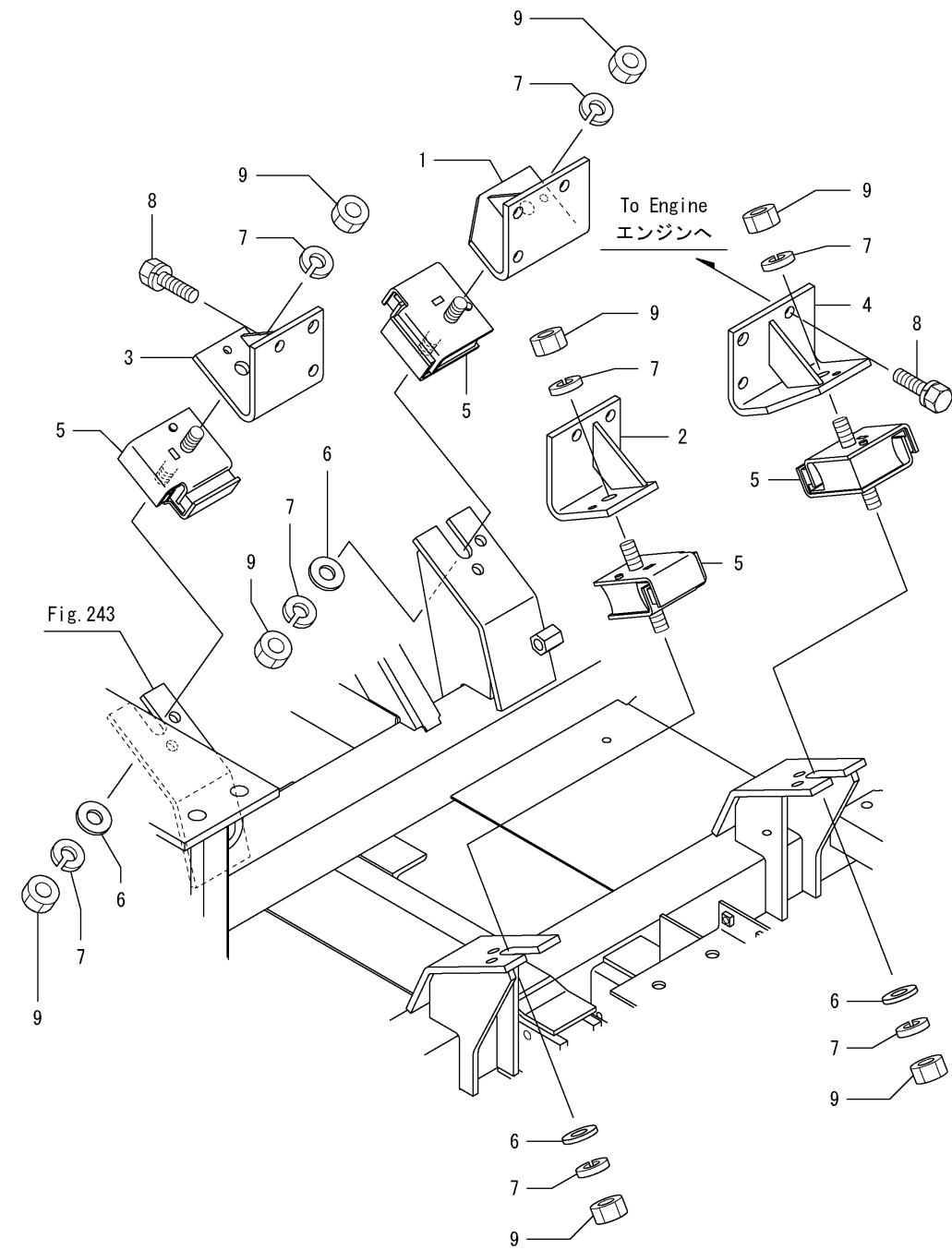
Fig.3. 엔진마운트
