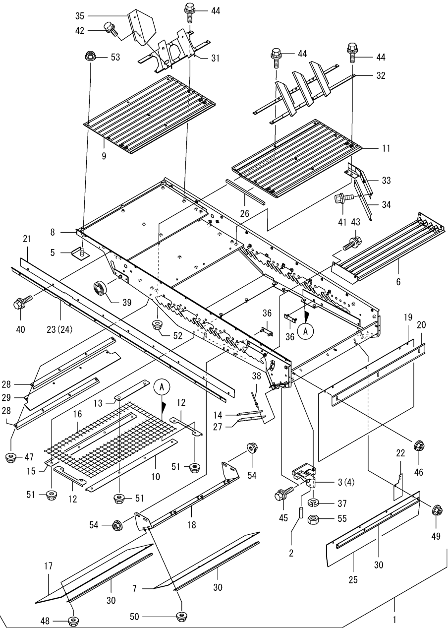
Fig.160. 요동선별판(1)
