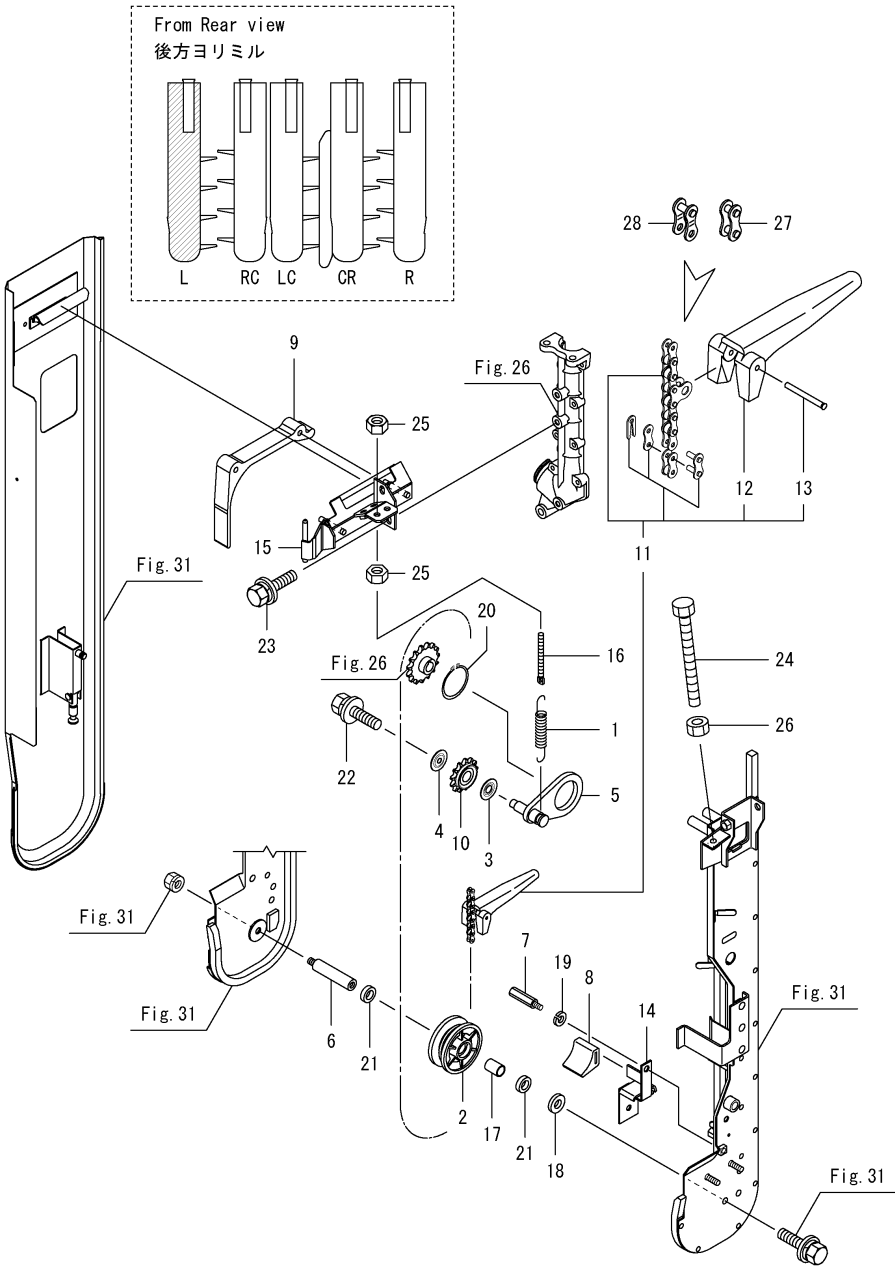
Fig.38. 인기체인롤러(좌)
