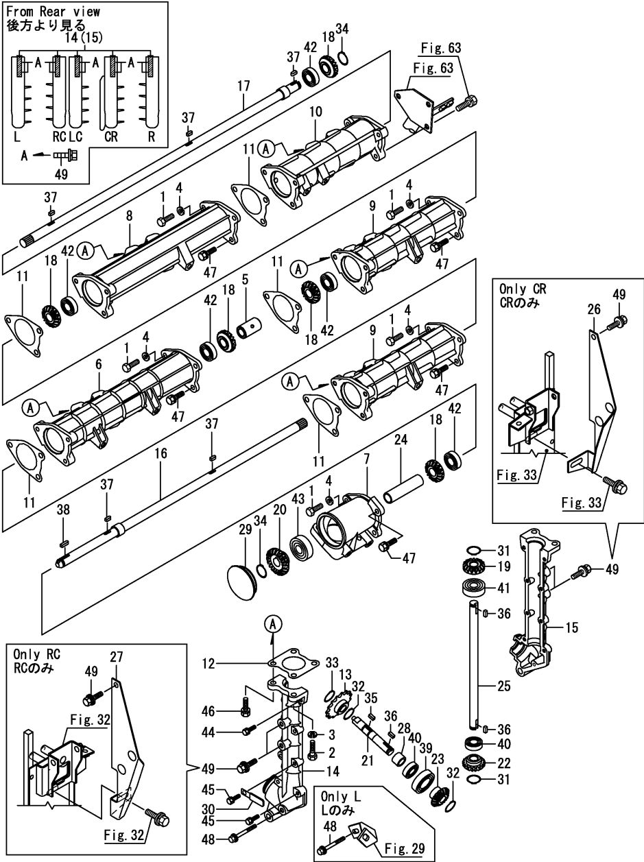
Fig.26. 픽업 수평 드라이브
