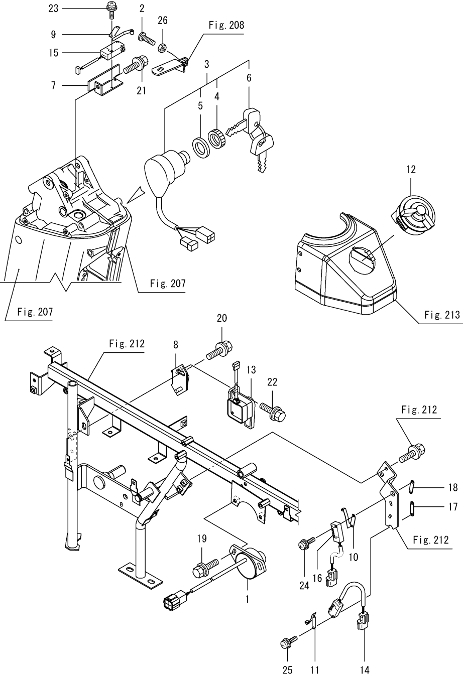
Fig.287. 스위치(곡물탱크)
