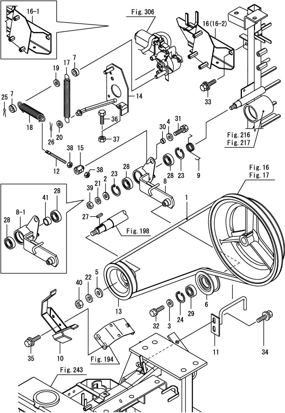
Fig.189. 예취구동벨트
