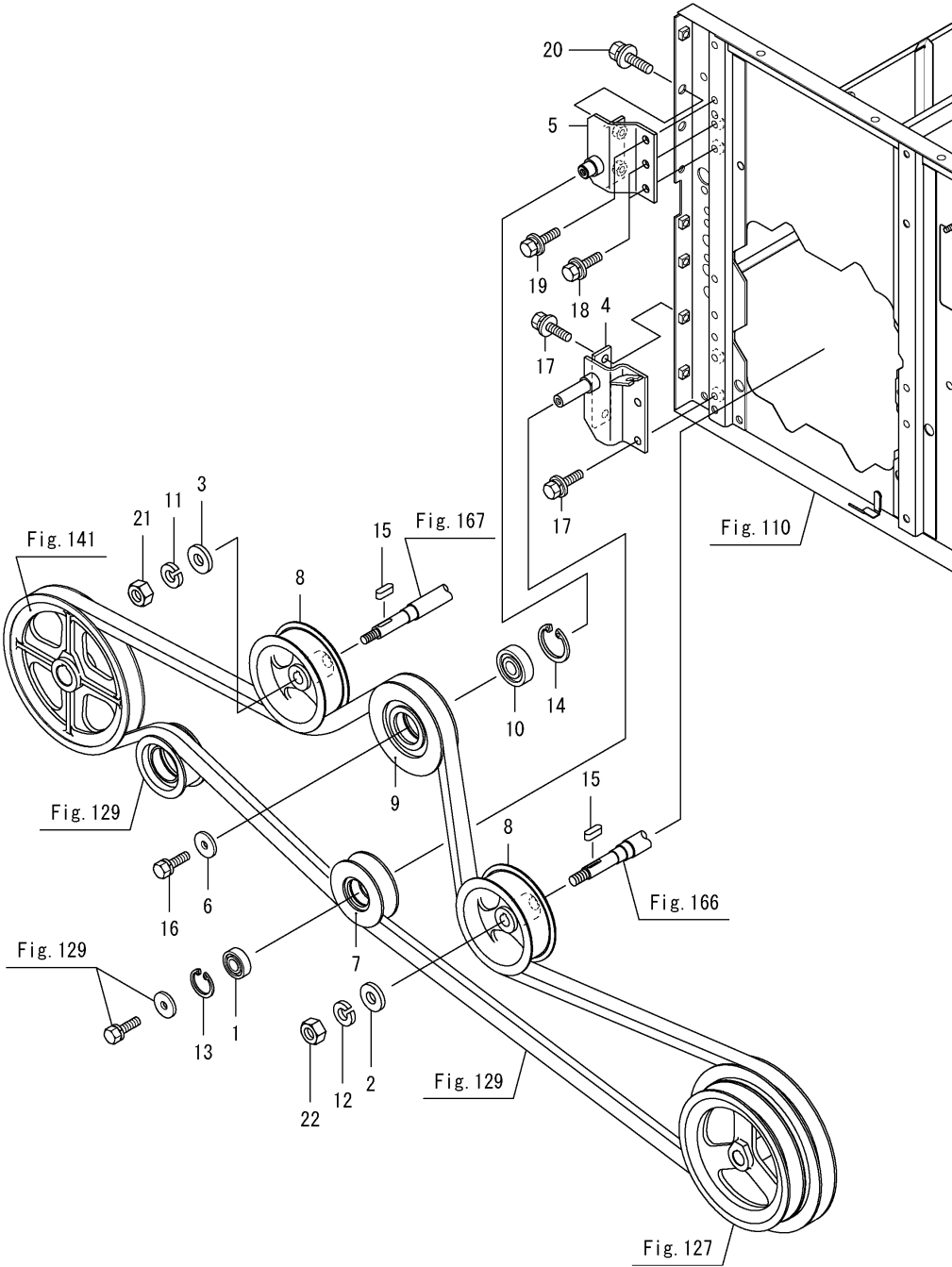
Fig.126. 풍구 벨트
