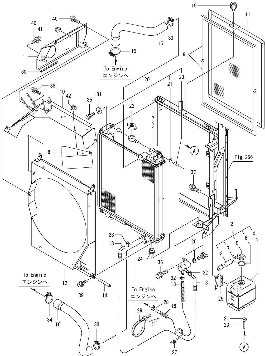
Fig.12. 라디에이터
