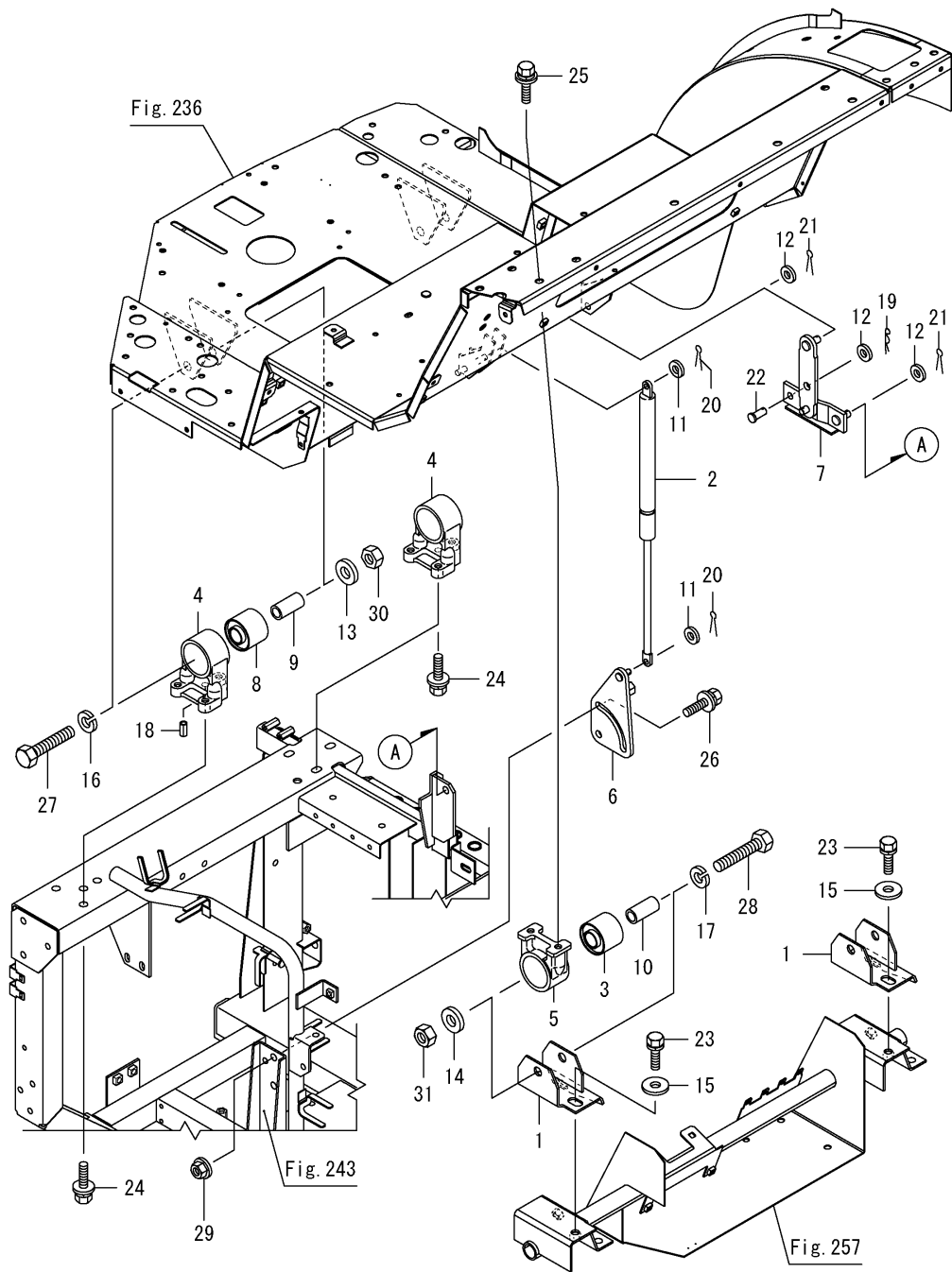
0CNP5-M34400 이동(2) Fig.232. 발판방진(캐빈)
