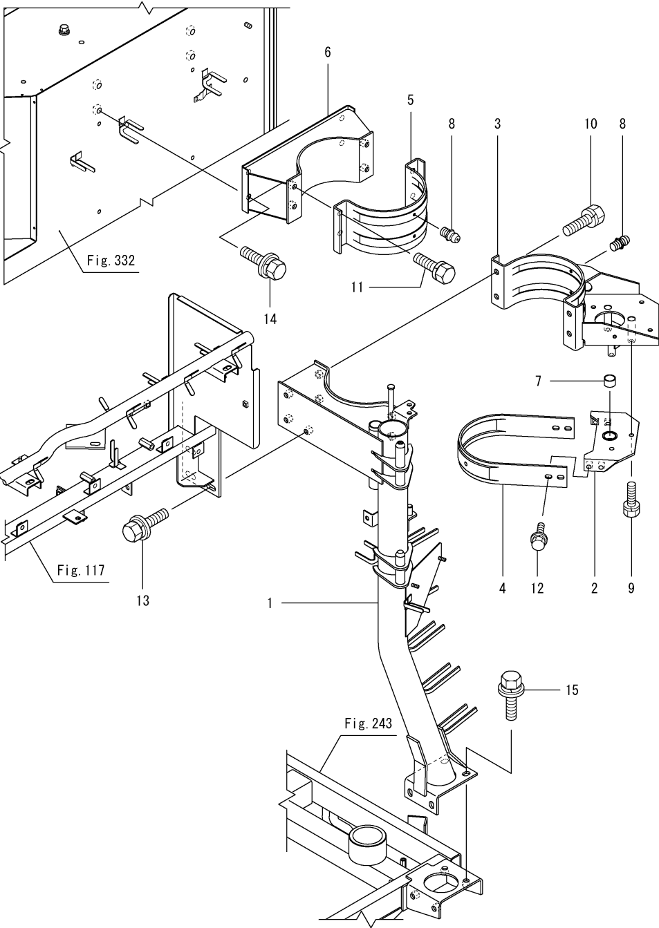
Fig.324. 종오거프레임
