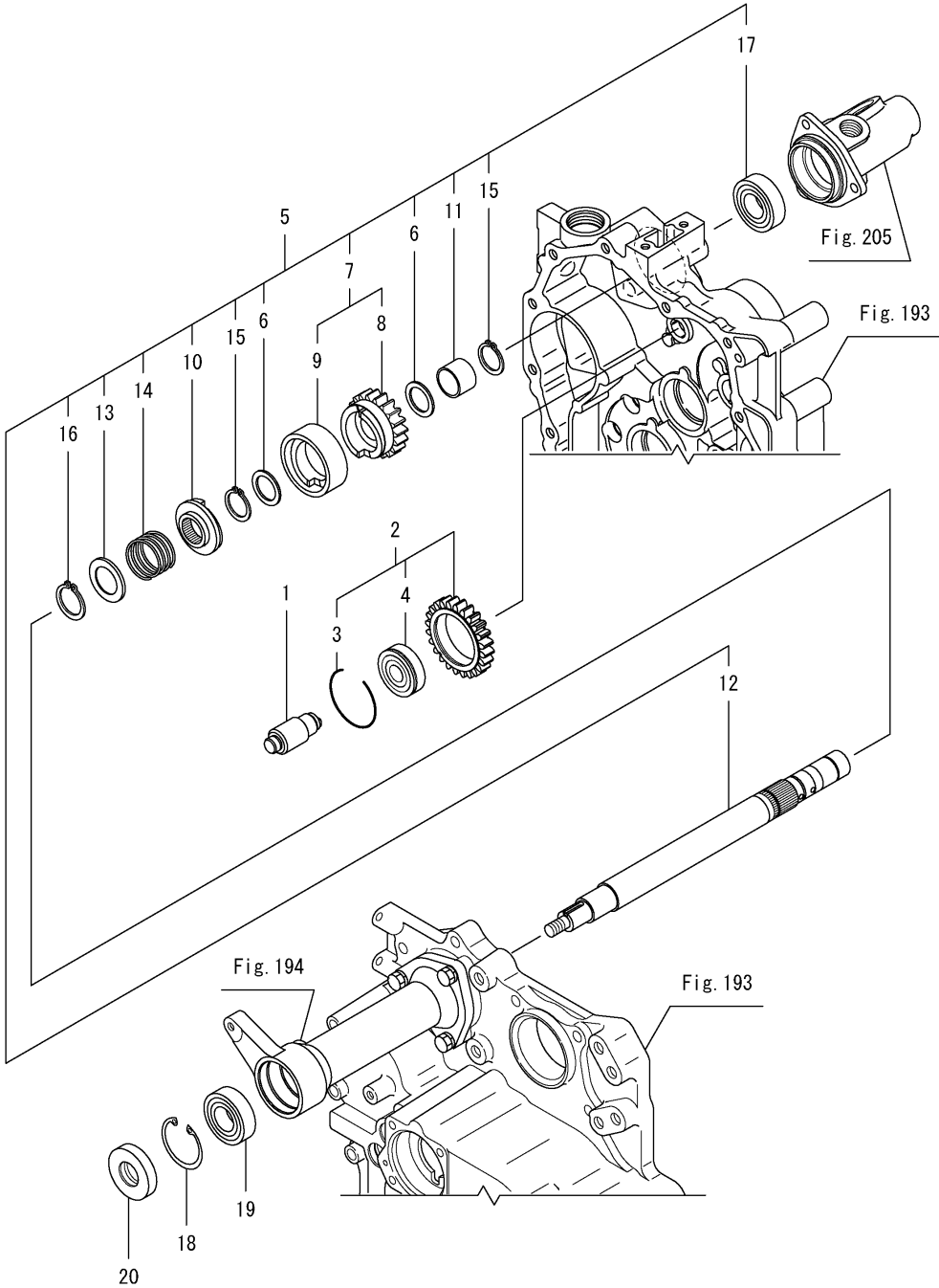
Fig.198. P.T.O. 축
