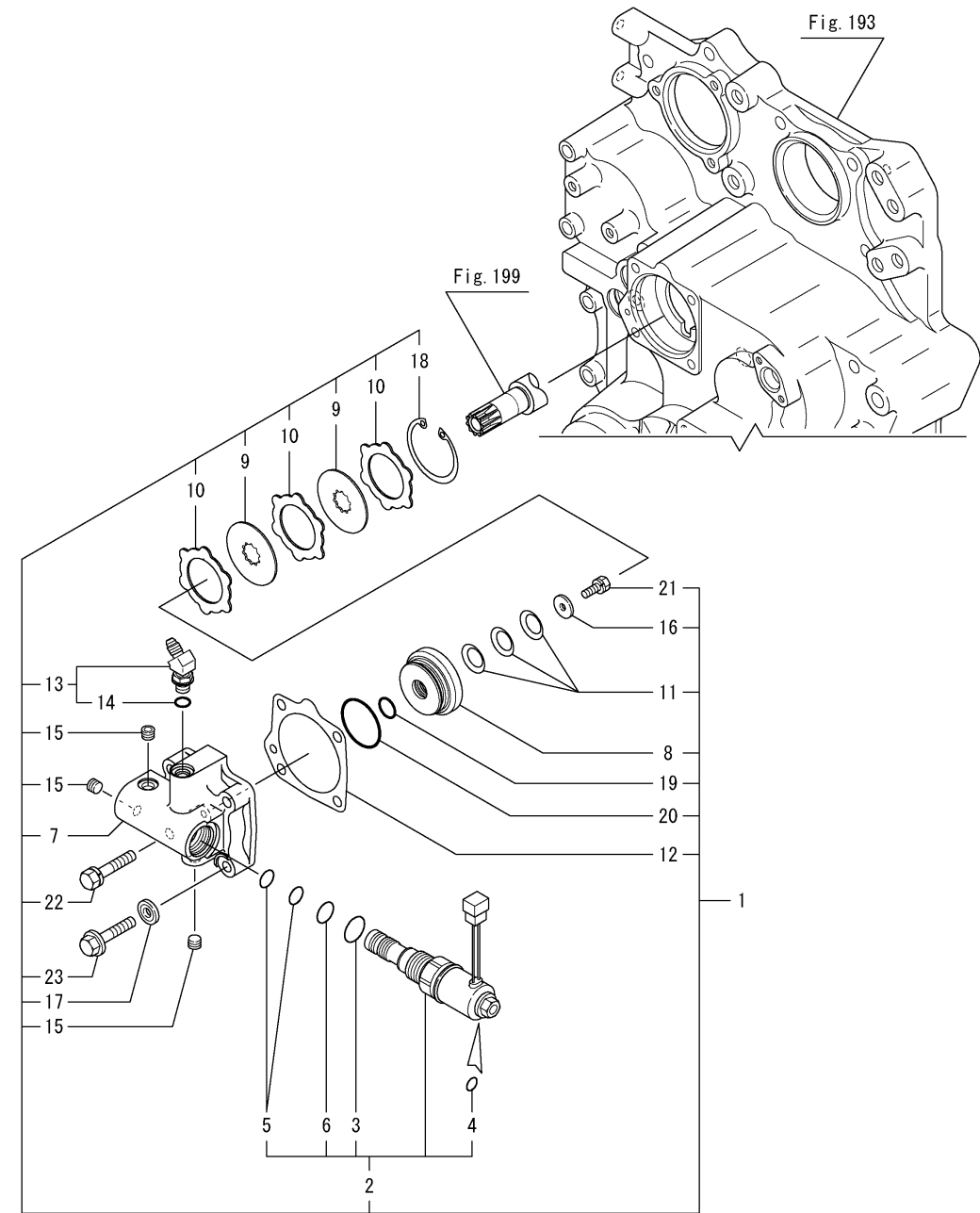
Fig.192. 스티어링 브레이크
