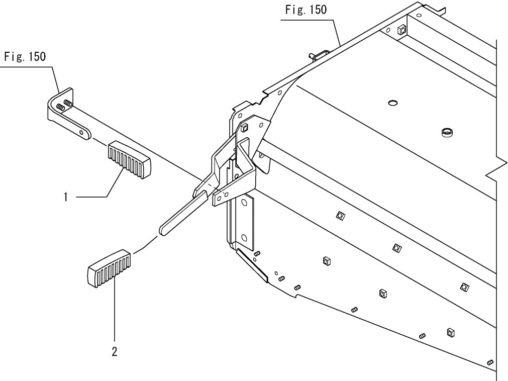
Fig.151. 탈곡실커버(2)
