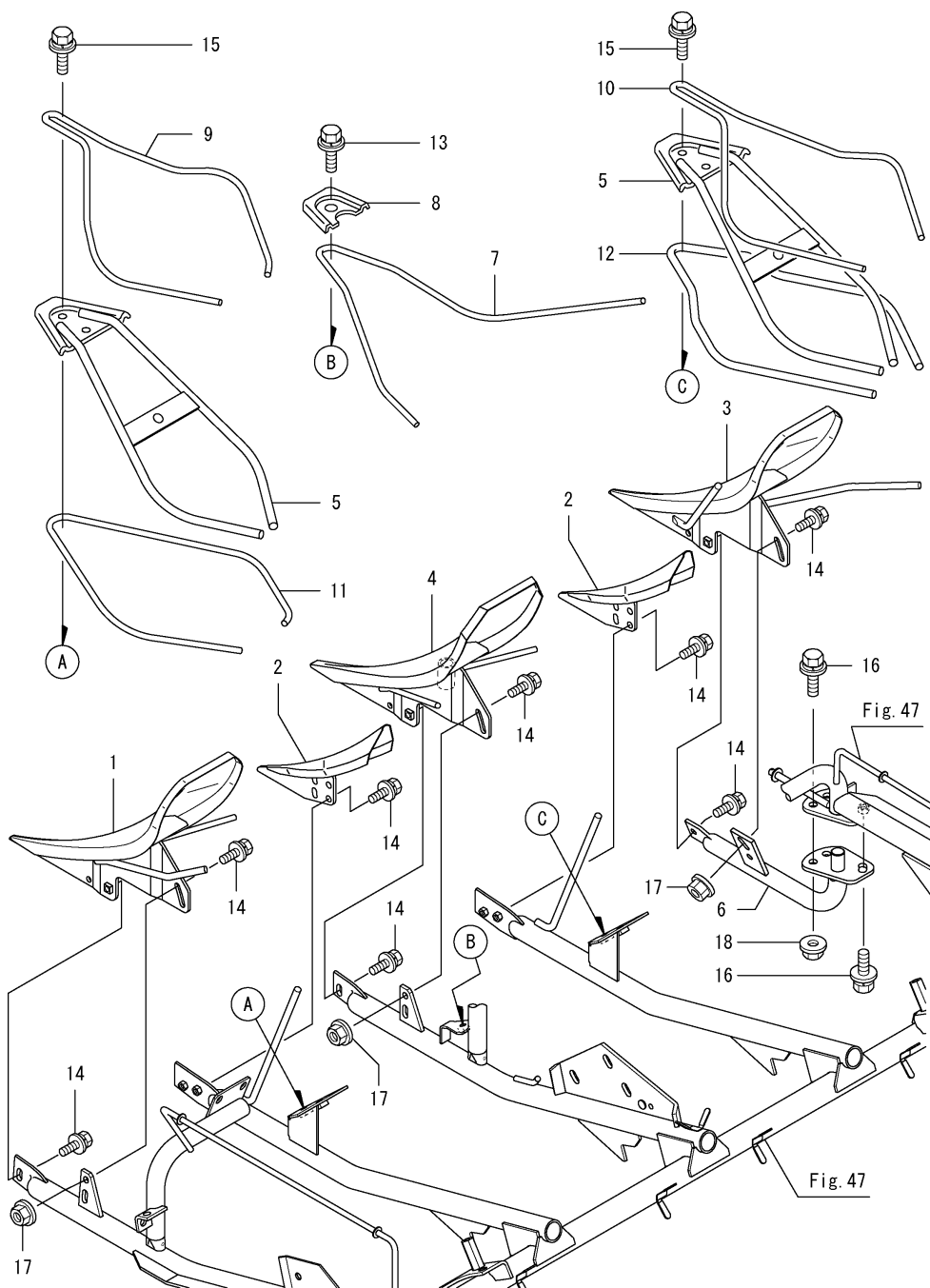
Fig.54. 디바이더판(왼쪽)
