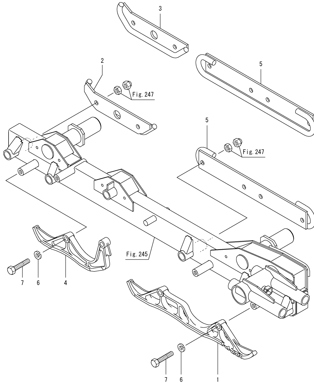
Fig.249. 크롤러 가이드
