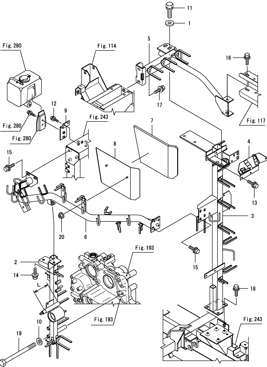
OCNP5-M34400 이동(2) Fig.217. 엔진프레임(뒤)(캐빈)
