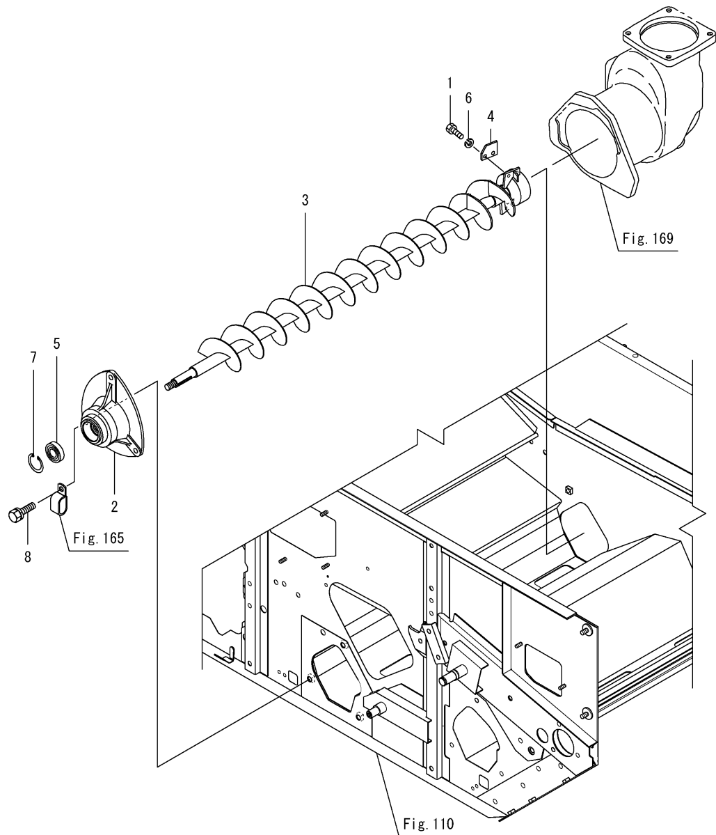
Fig.168. 컨베이어(1차)
