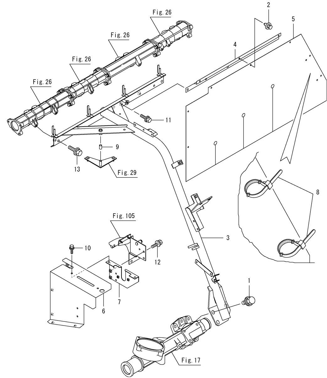
Fig.58. 보조패널
