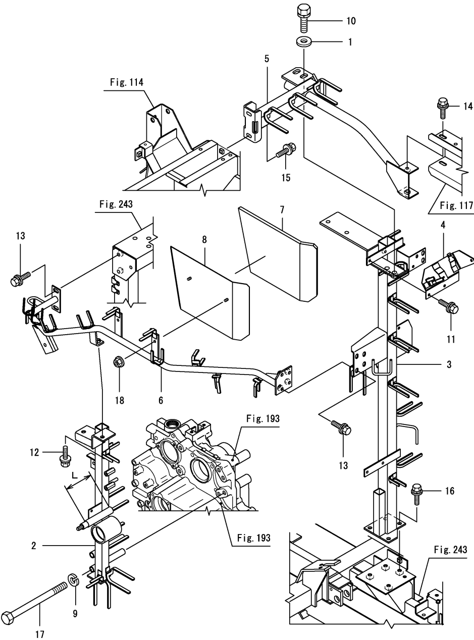
Fig.216. 엔진프레임(뒤)
