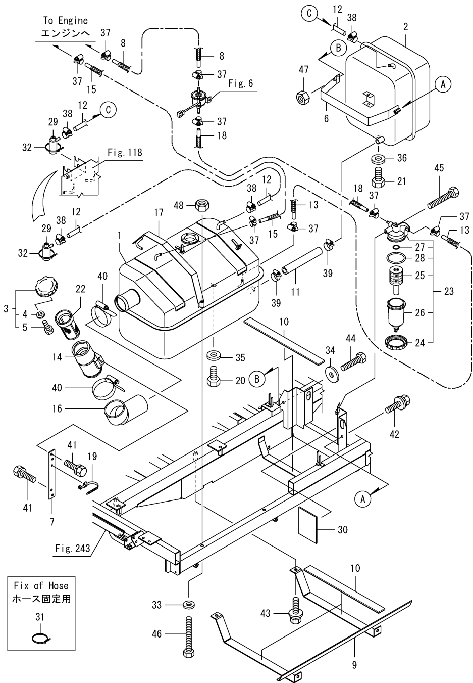
Fig.4. 연료탱크
