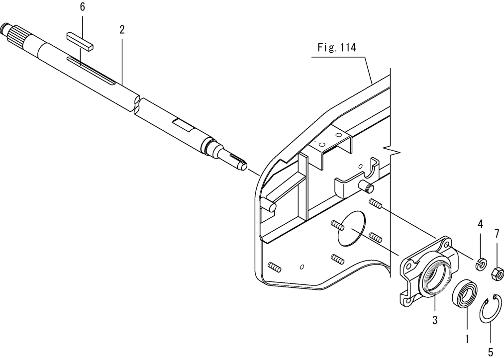
Fig.149. 탈곡통(메탈축)
