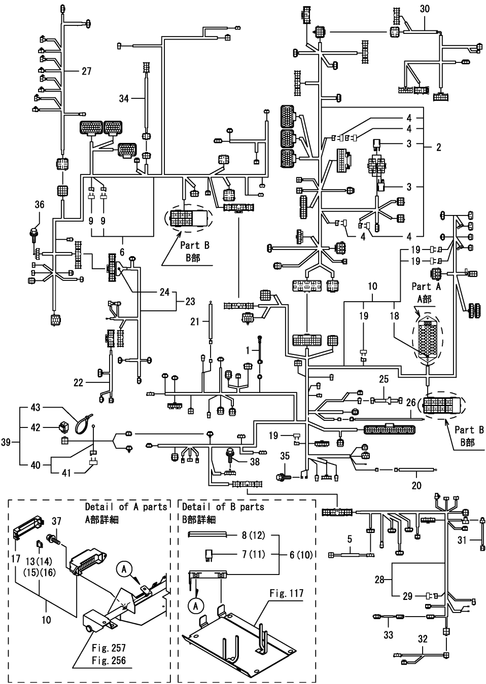
Fig.297. 배선 하네스(1)
