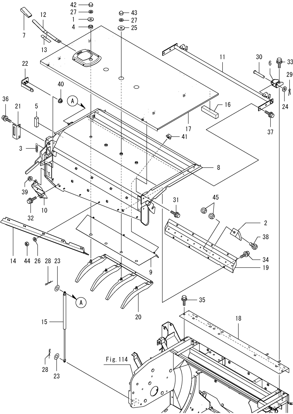
Fig.150. 탈곡실커버(1)
