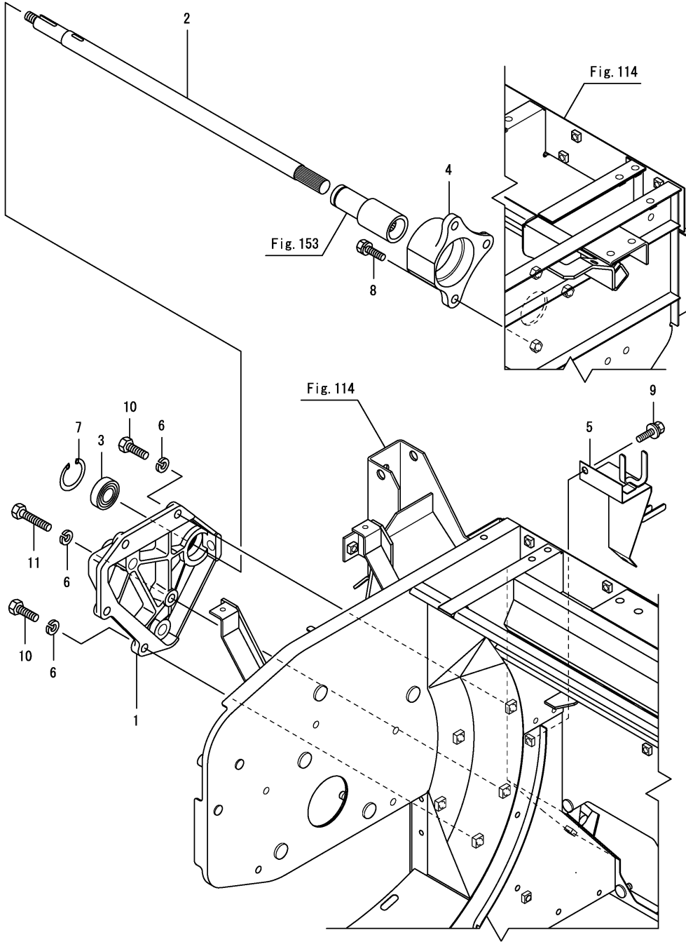
OCNP5-M34400 탈곡(2) Fig.154. 처리 드럼 드라이브 축
