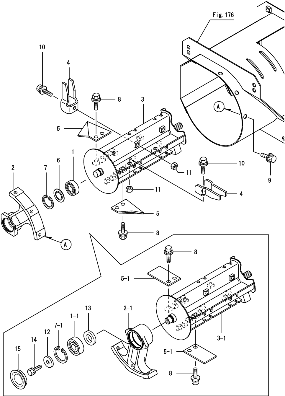
Fig.175. 처리 드럼(2차)
