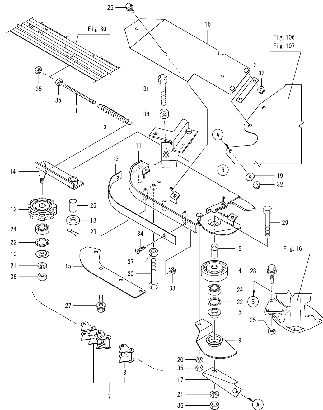
Fig.103. 보조반송
