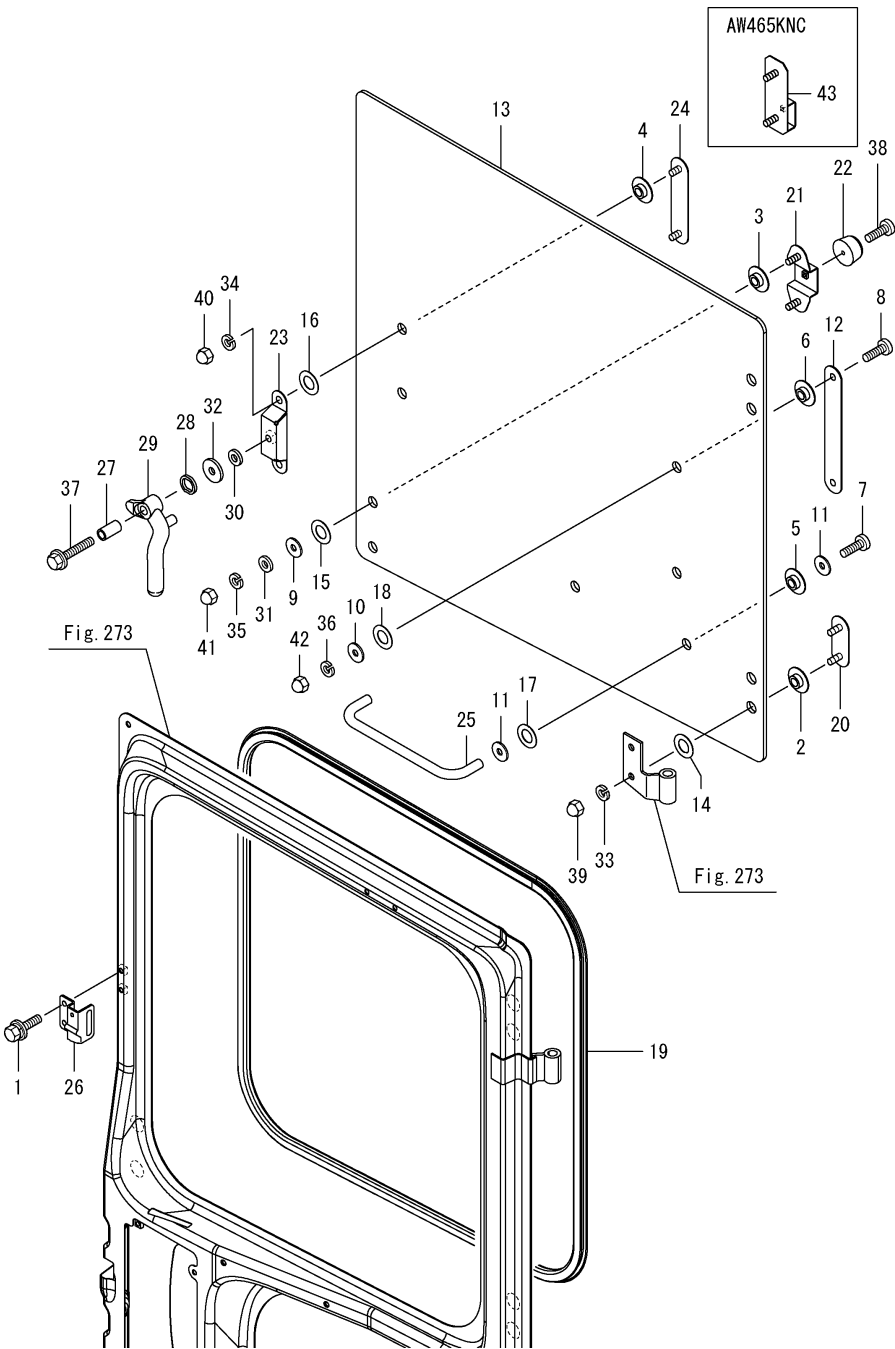
Fig.275. 캐빈(문)(3)
