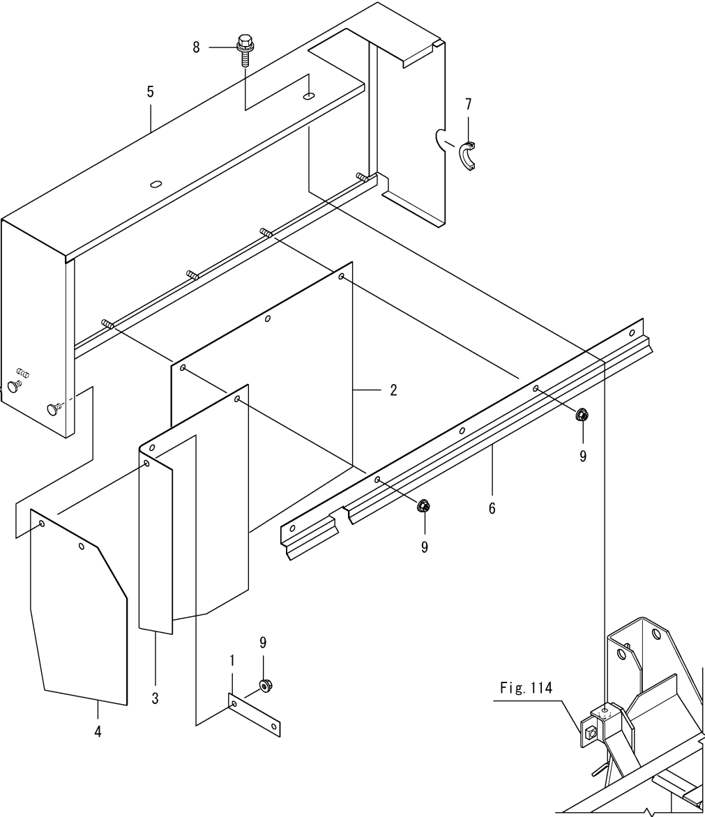
Fig.139. 탈곡통커버(앞)(2)
