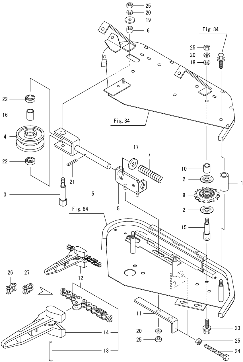
Fig.87. 상반송롤러(좌)
