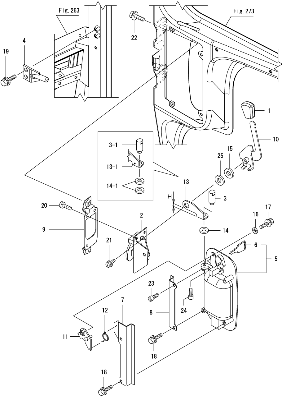
Fig.274. 캐빈(문)(2)
