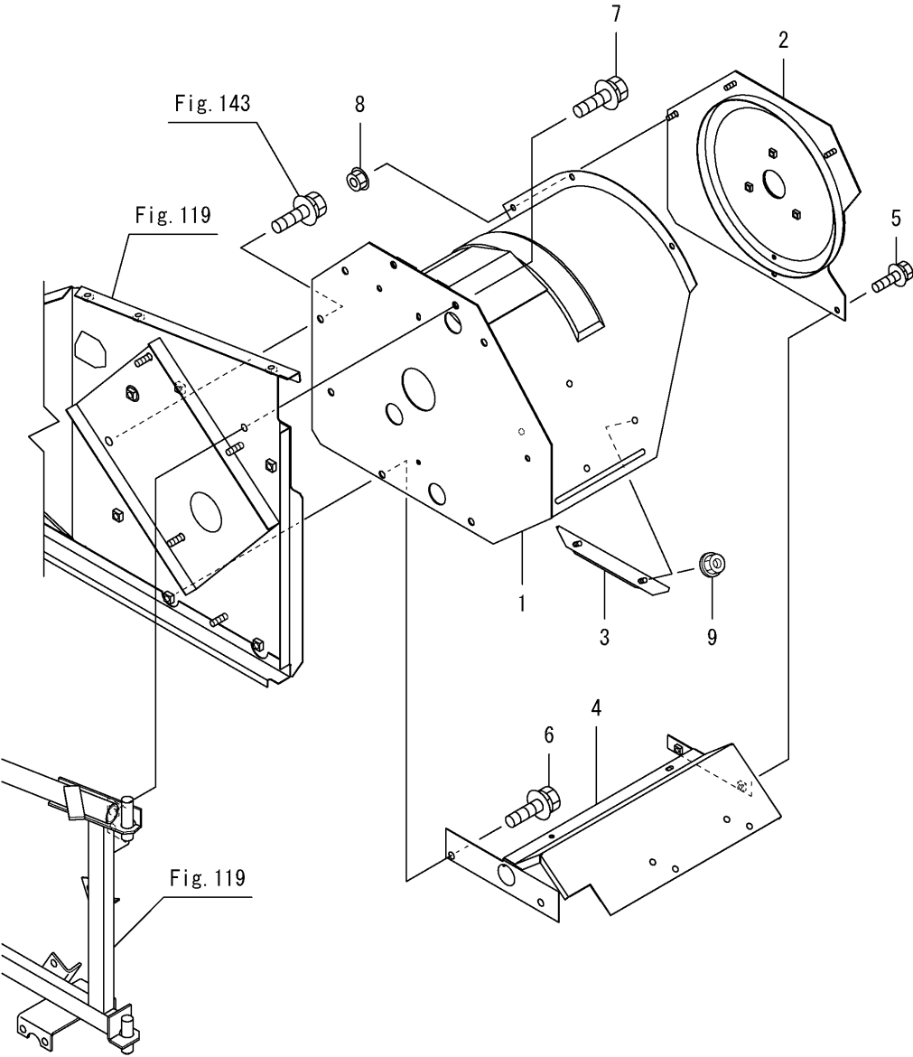
Fig.177. 흡입 드럼
