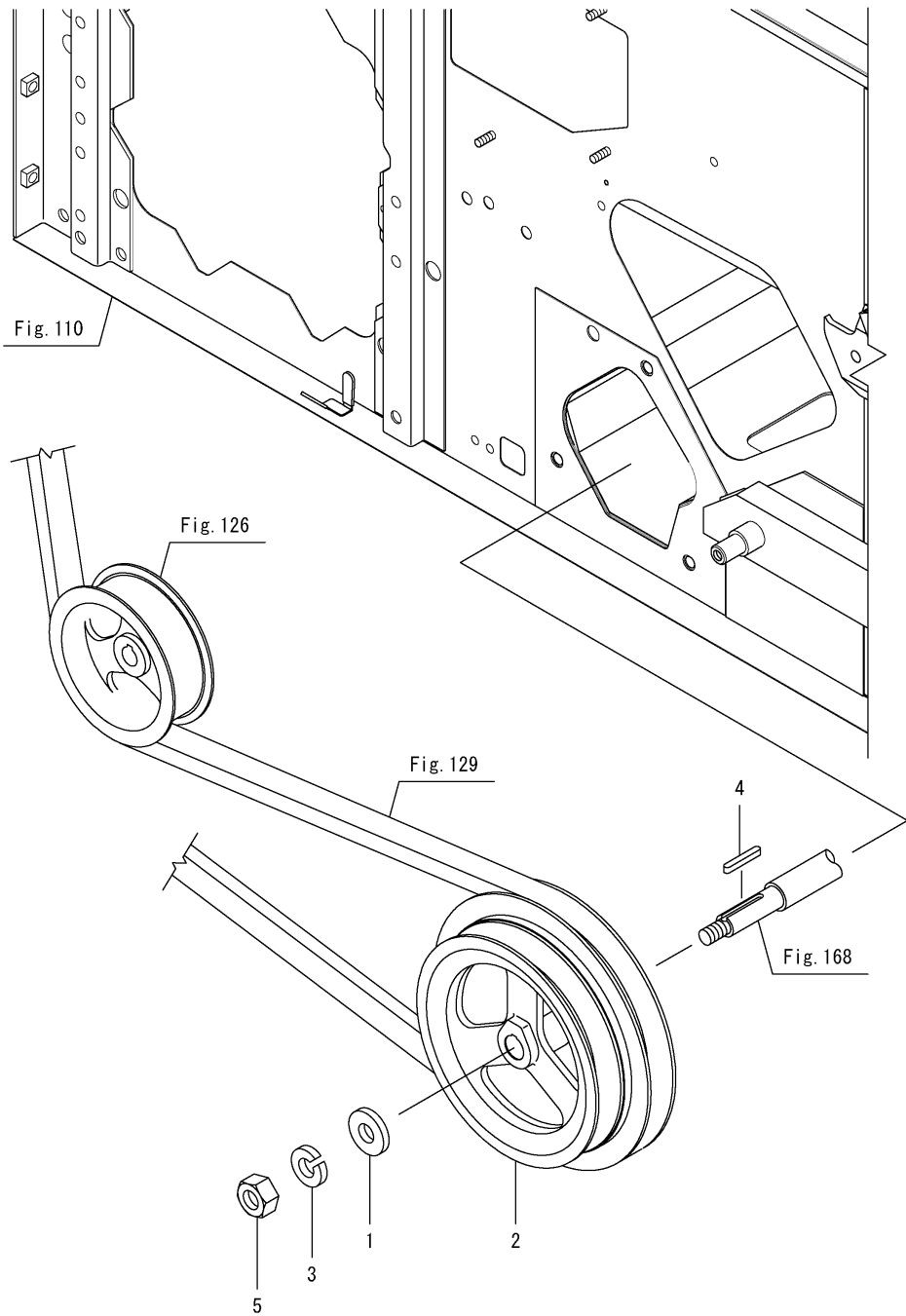
Fig.127. 벨트(1차)
