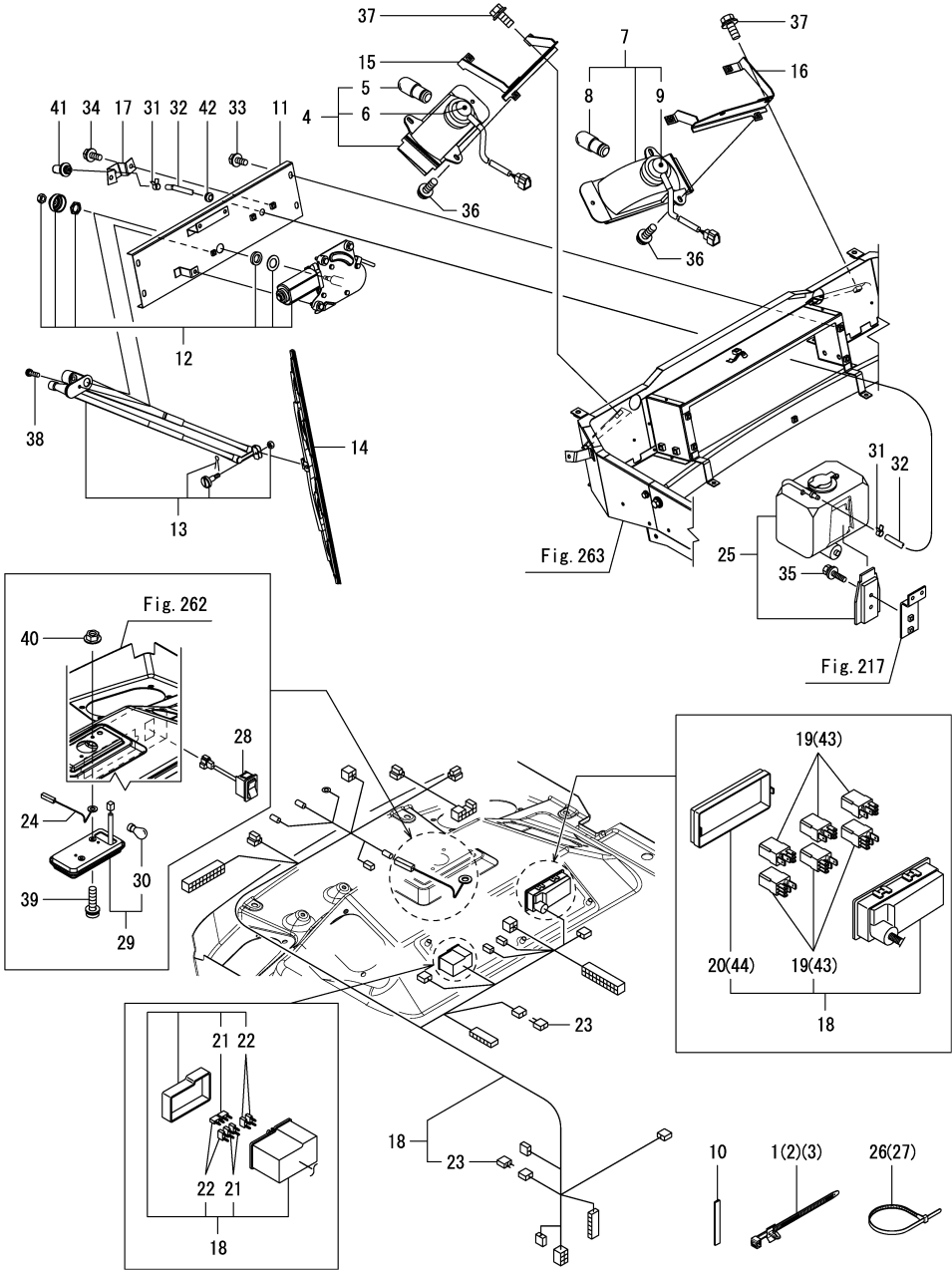
Fig.280. 전장품(캐빈)
