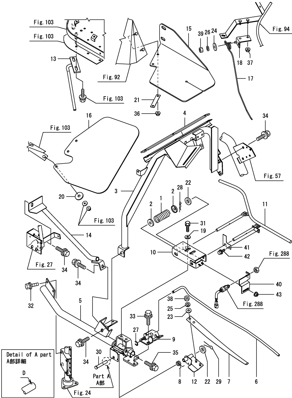
Fig.107. 보조반송가이드
