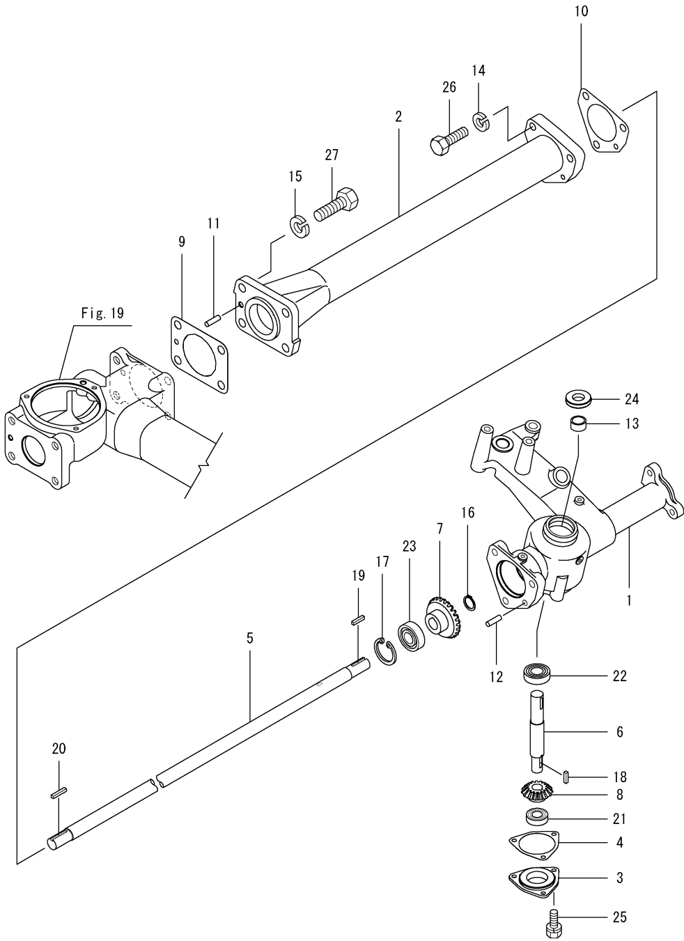
Fig.22. 4번축케이스(우)
