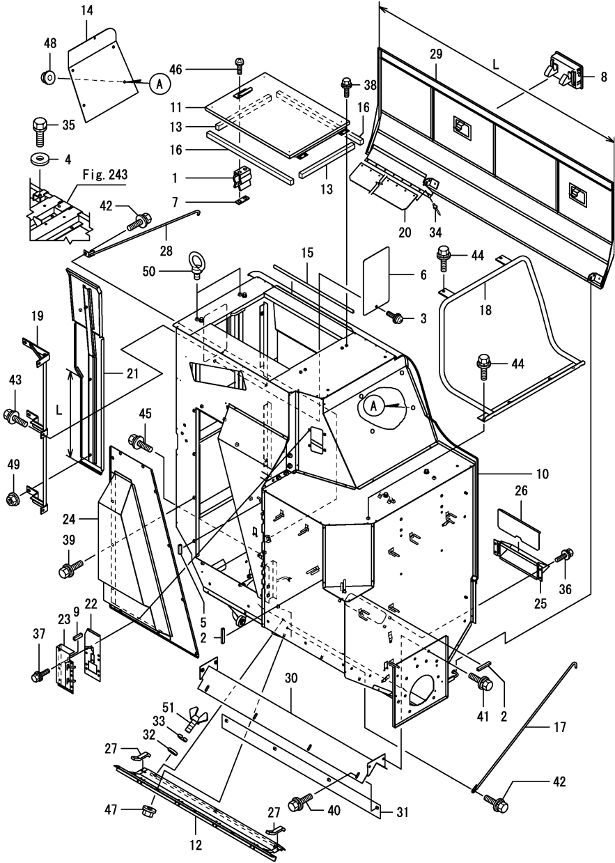
Fig.332. 곡물탱크
