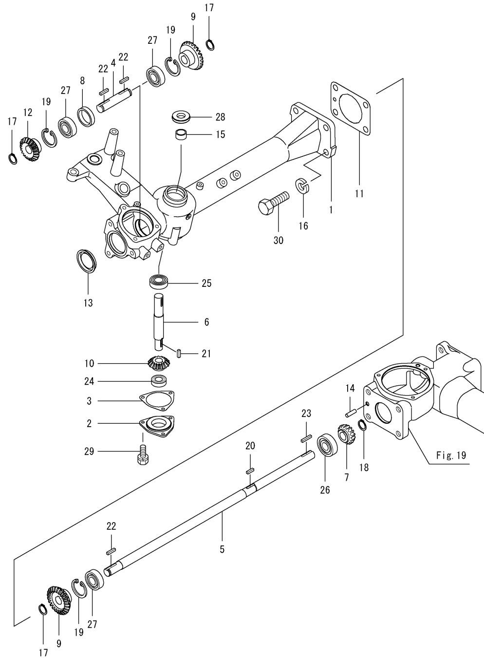
Fig.20. 3번축케이스(좌)
