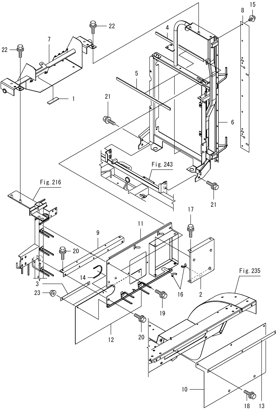
Fig.256. 엔진실프레임
