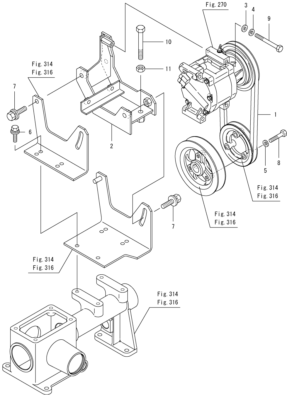
Fig.276. 콤프레셔취부
