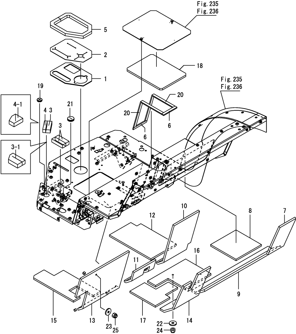
Fig.241. 바닥 시일
