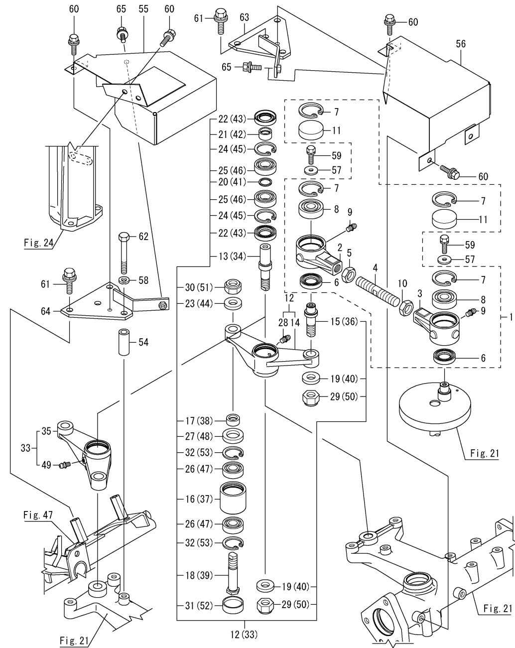
Fig.49. 예취날구동
