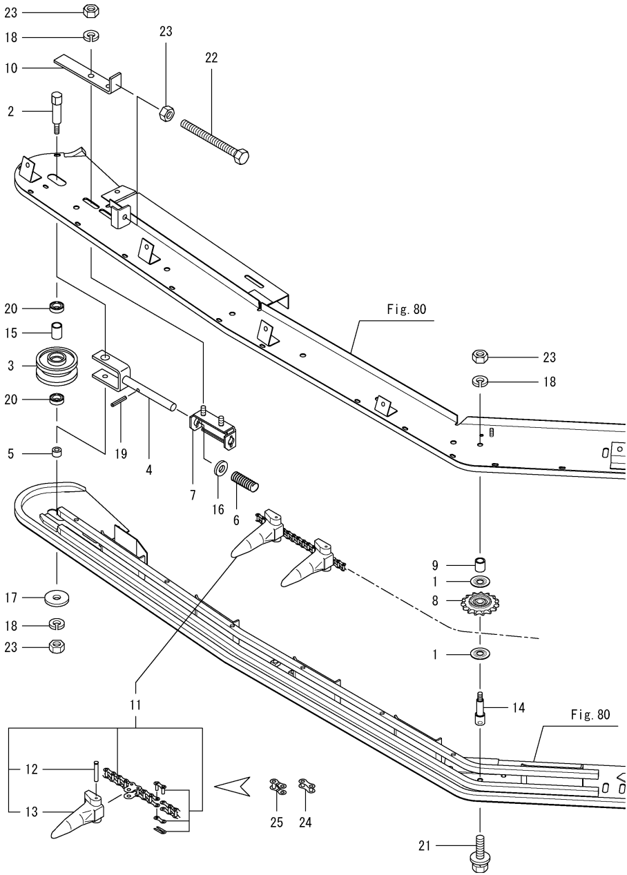
Fig.82. 상반송롤러(우)
