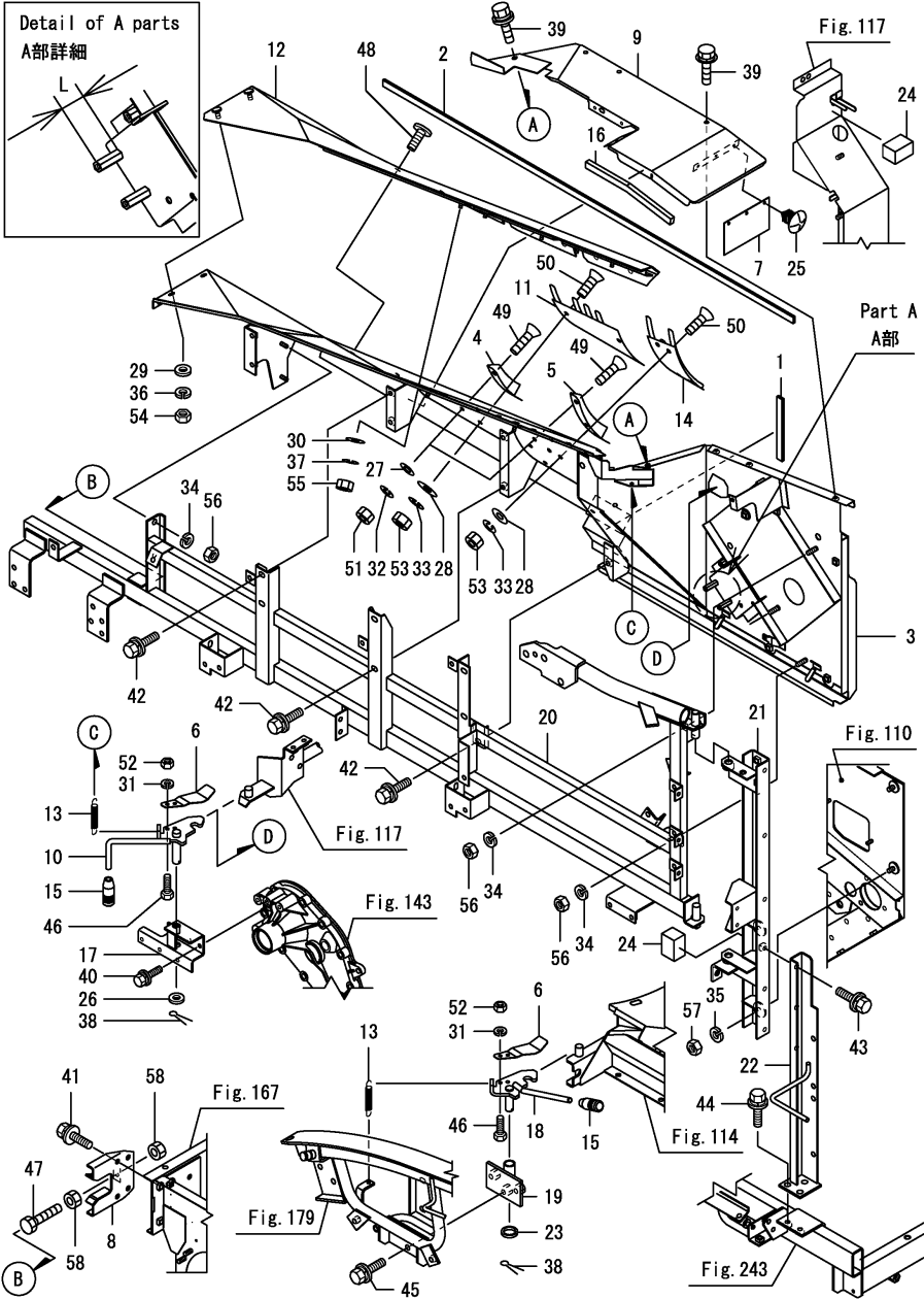
Fig.119. 탈곡실프레임(좌)
