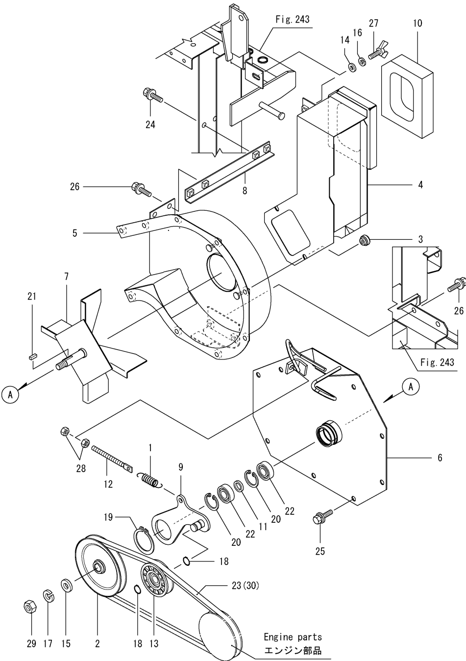
Fig.15. 스크린 흡입기
