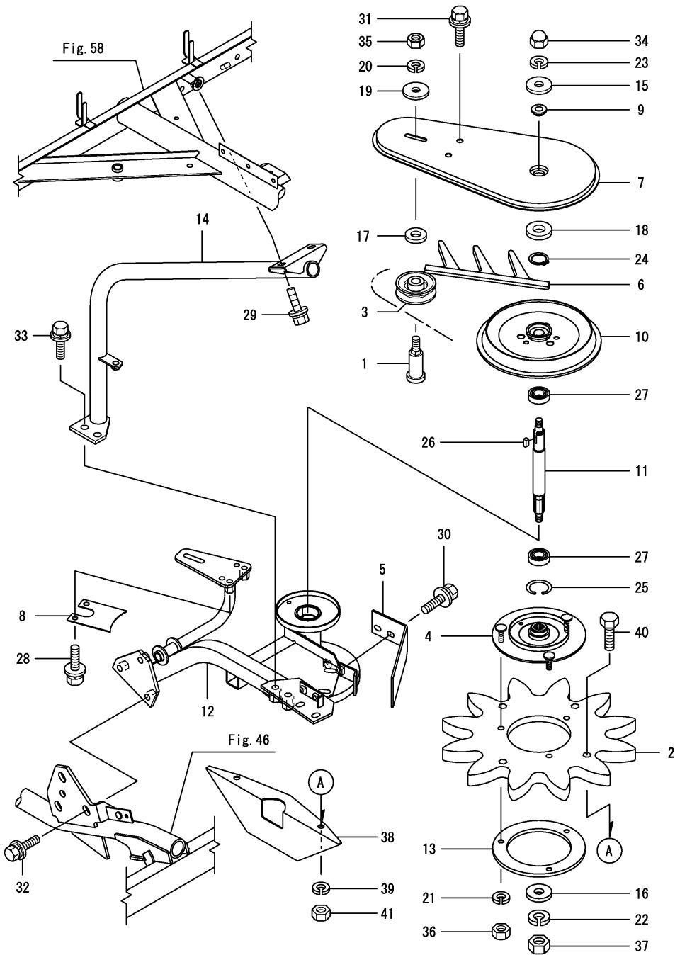
Fig.67. 끌어모음벨트(중-우)
