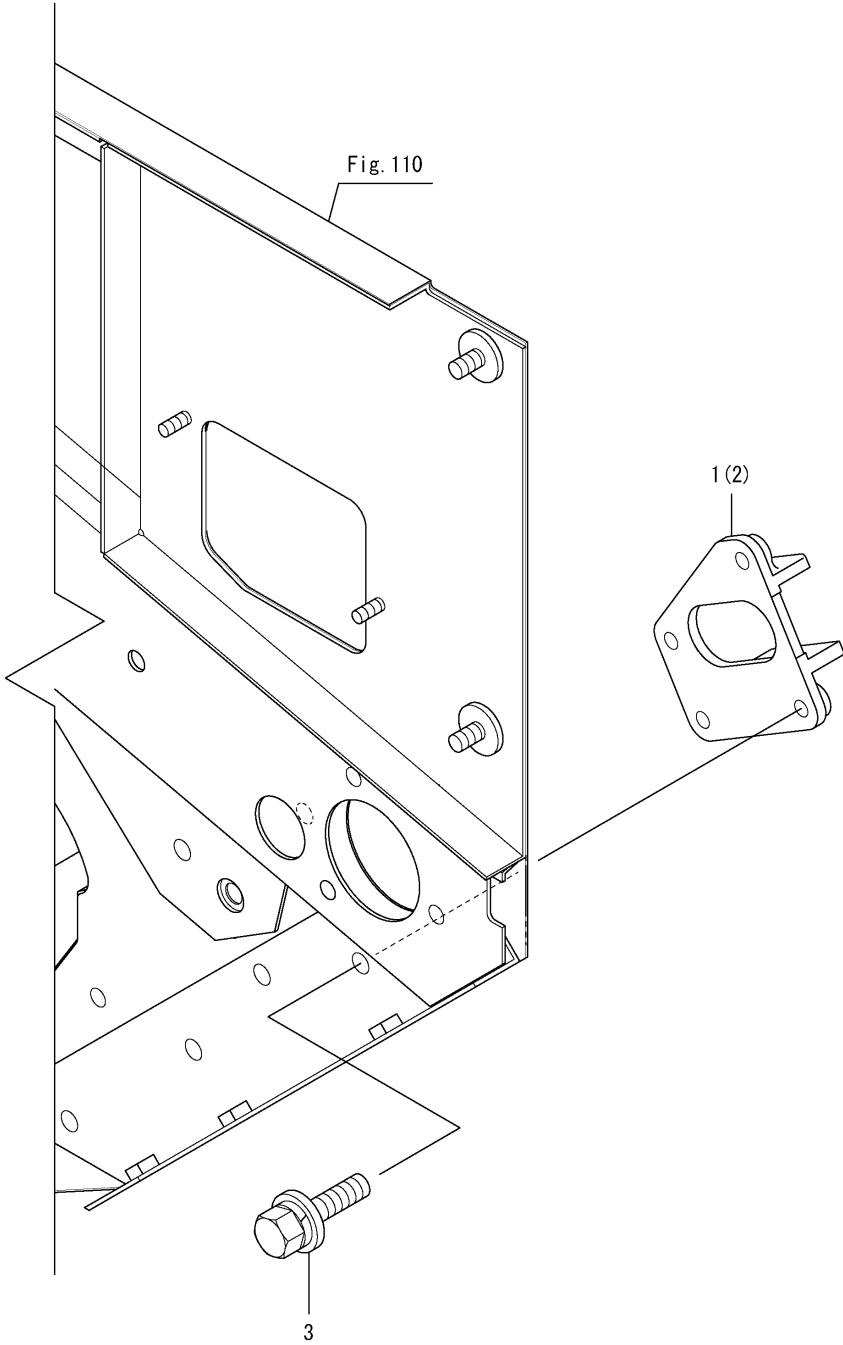
Fig.159. 스윙 암(후면)
