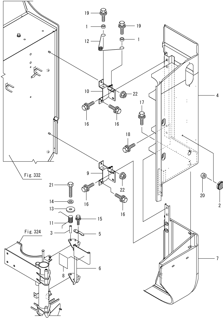
Fig.338. 탱크커버
