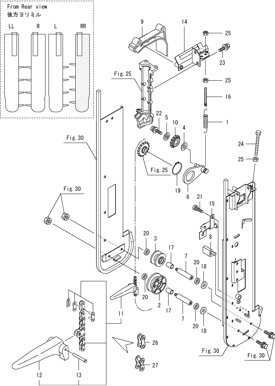
Fig.36. 인기체인롤러(우-우)
