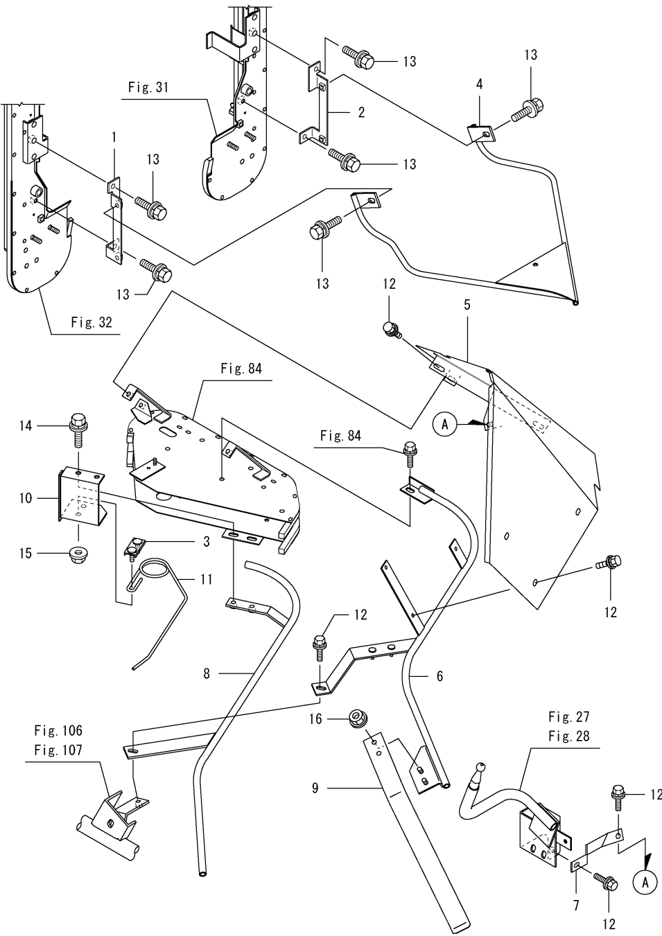
0CNP5-M34400 수확(2) Fig.94. 상단 이송 가이드(왼쪽)
