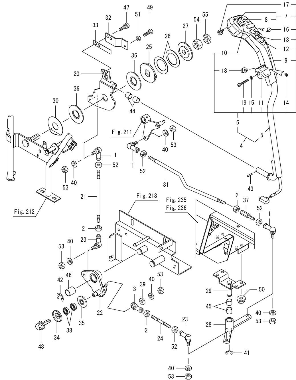
Fig.219. 주변속조작
