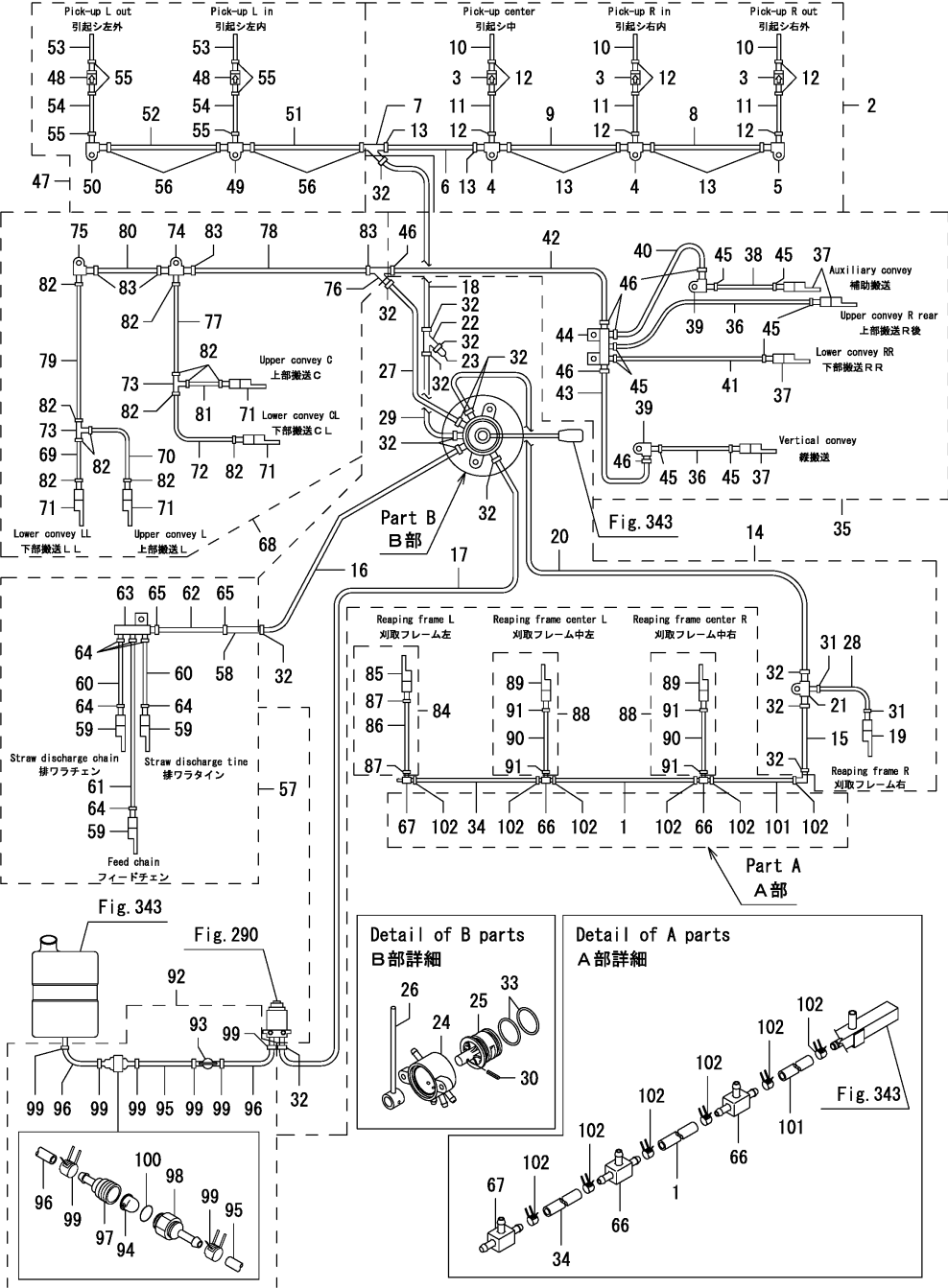
Fig.344. 주유장치(2)
