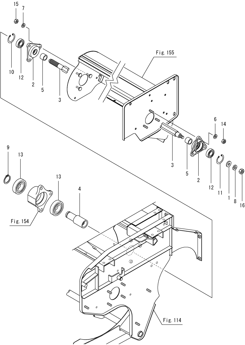
Fig.153. 처리 드럼 축
