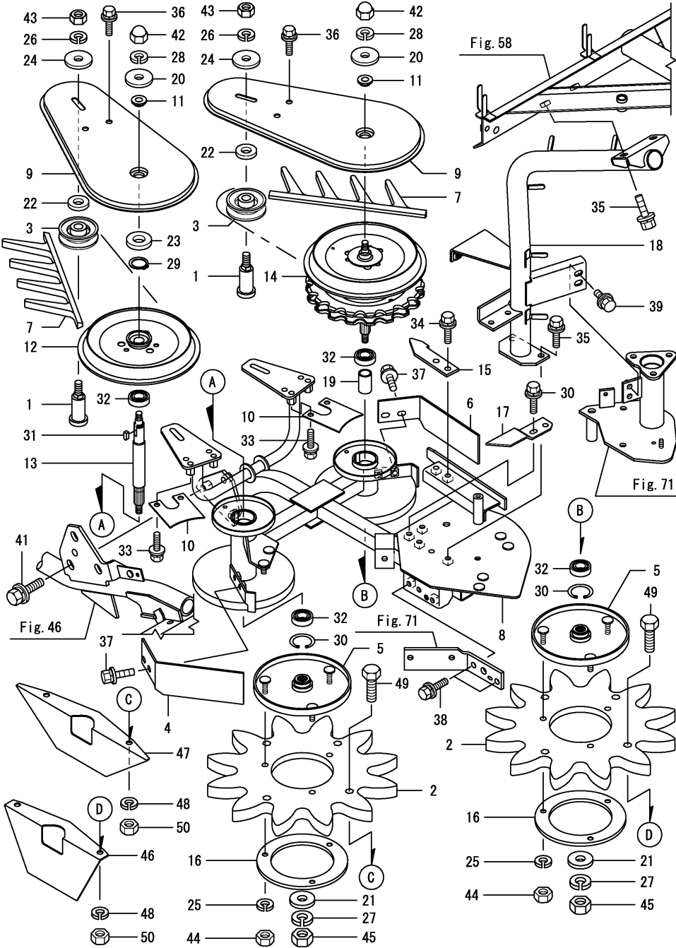
Fig.68. 끌어모음벨트(중-좌)
