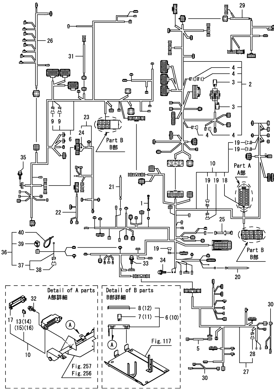
Fig.299. 배선 하네스(1)
