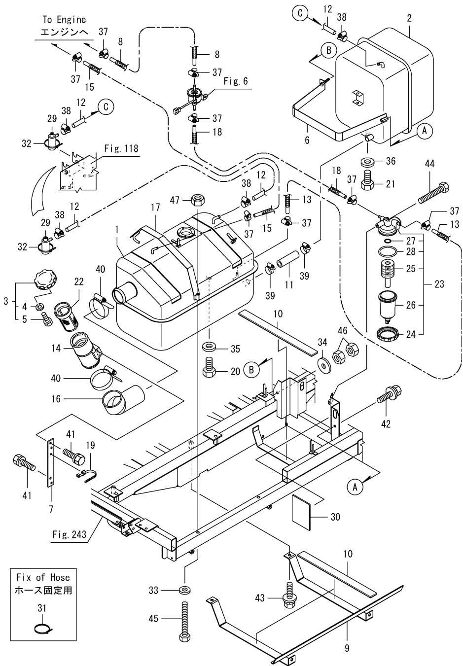
Fig.5. 연료탱크
