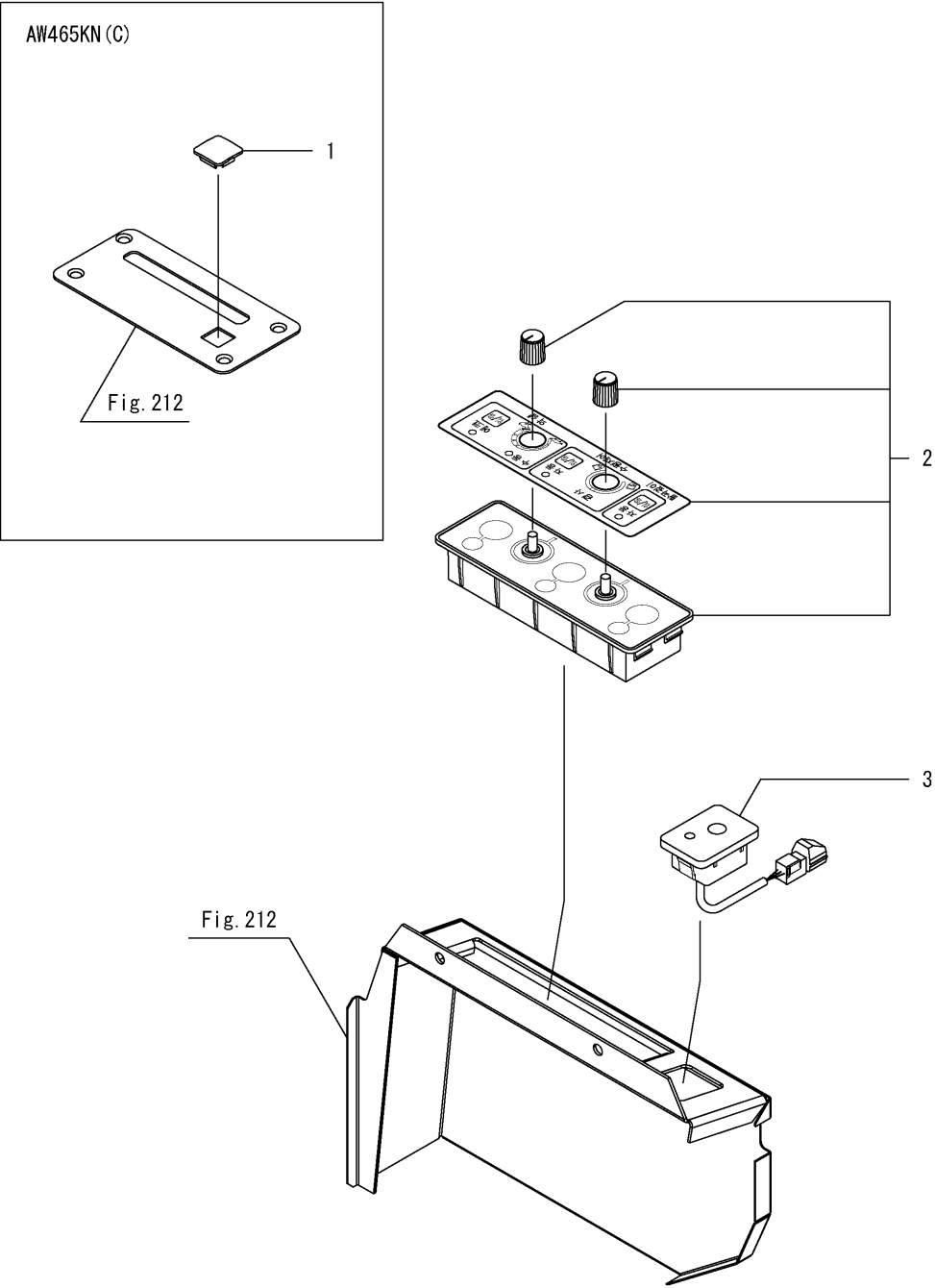
Fig.286. 스위치패널(GU)
