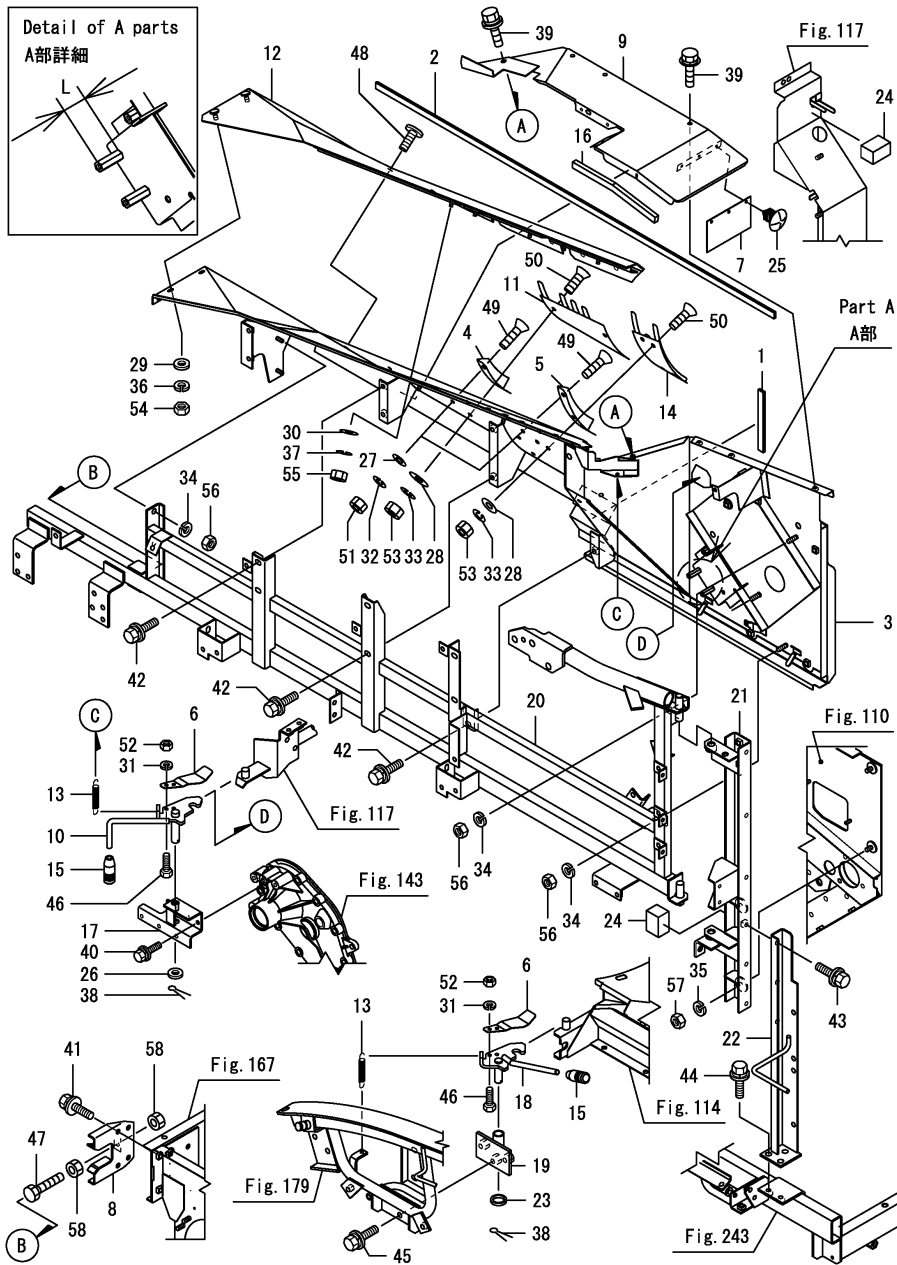
Fig.119. 탈곡실프레임(좌)
