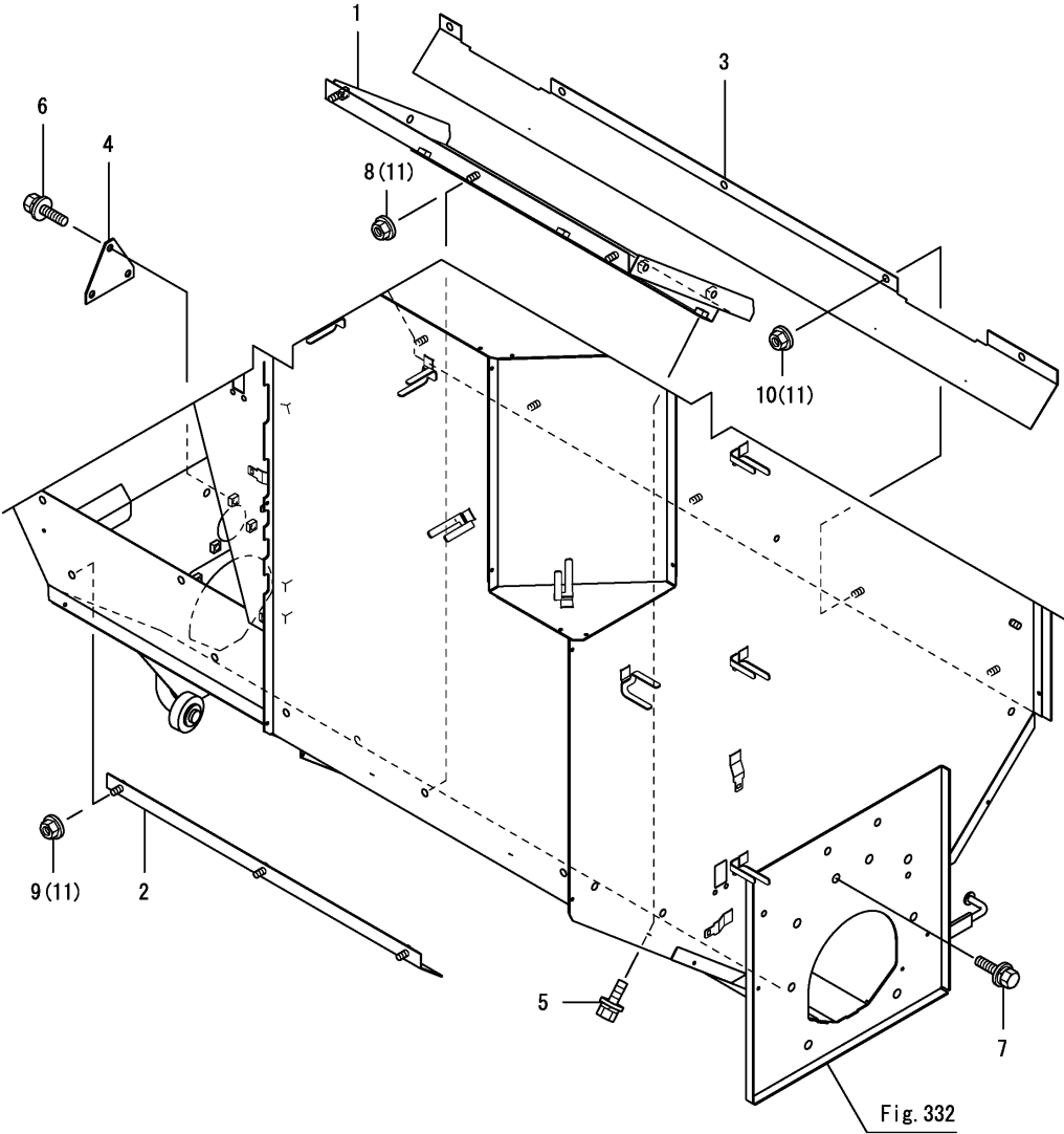
Fig.340. 스윙 플레이트
