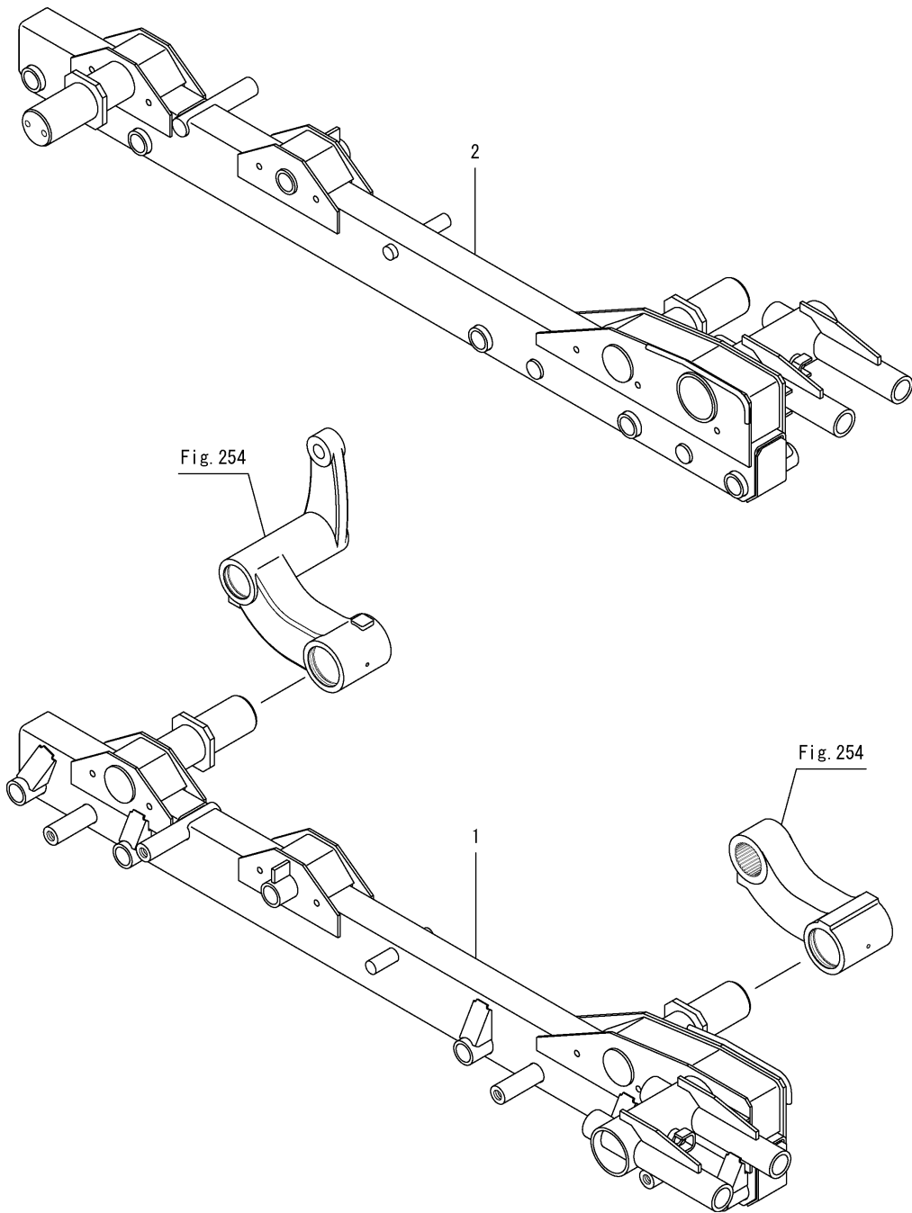
Fig.245. 트랙 프레임
