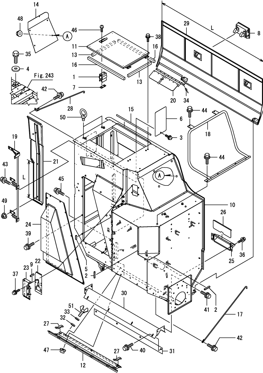
Fig.332. 곡물탱크
