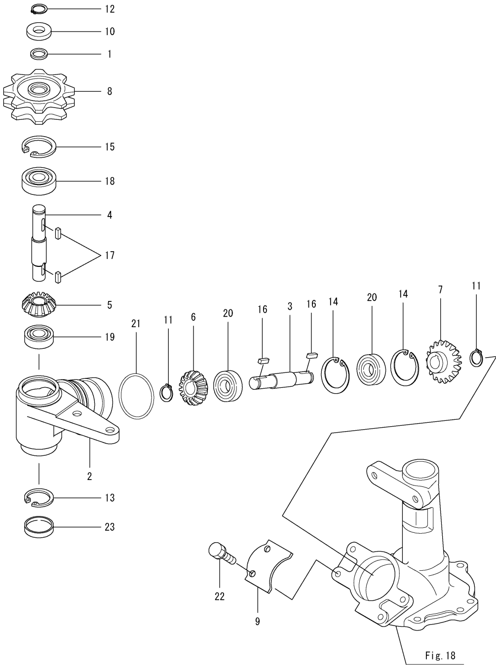
Fig.97. 수직 이송 케이스
