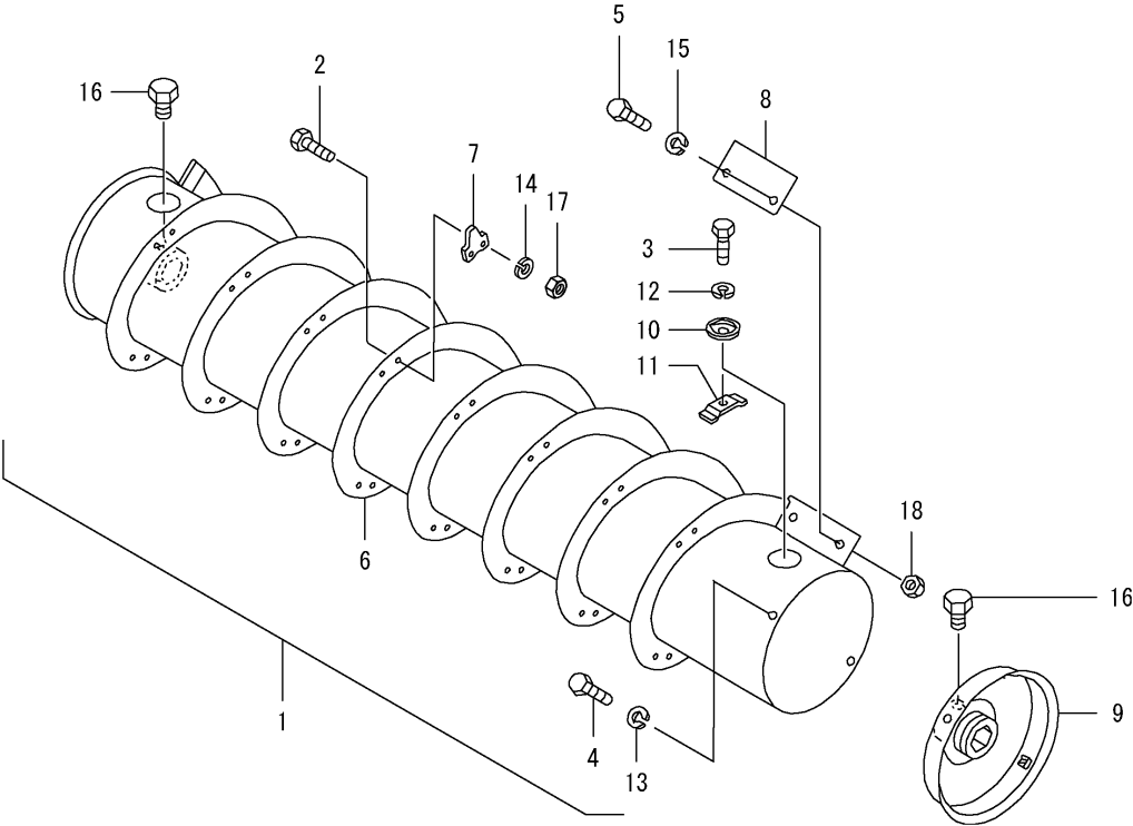
Fig.152. 처리 드럼
