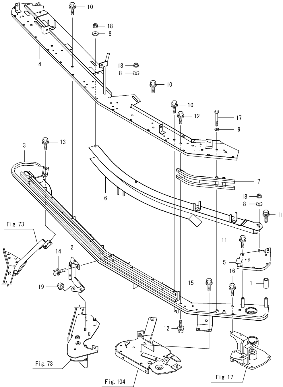
Fig.81. 상단 이송 케이스(오른쪽)
