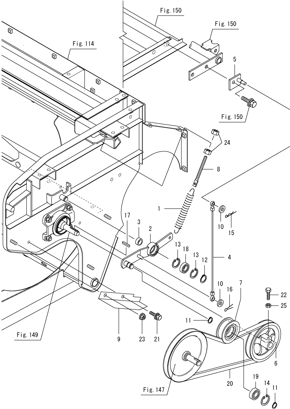
Fig.137. 짚 방출 벨트
