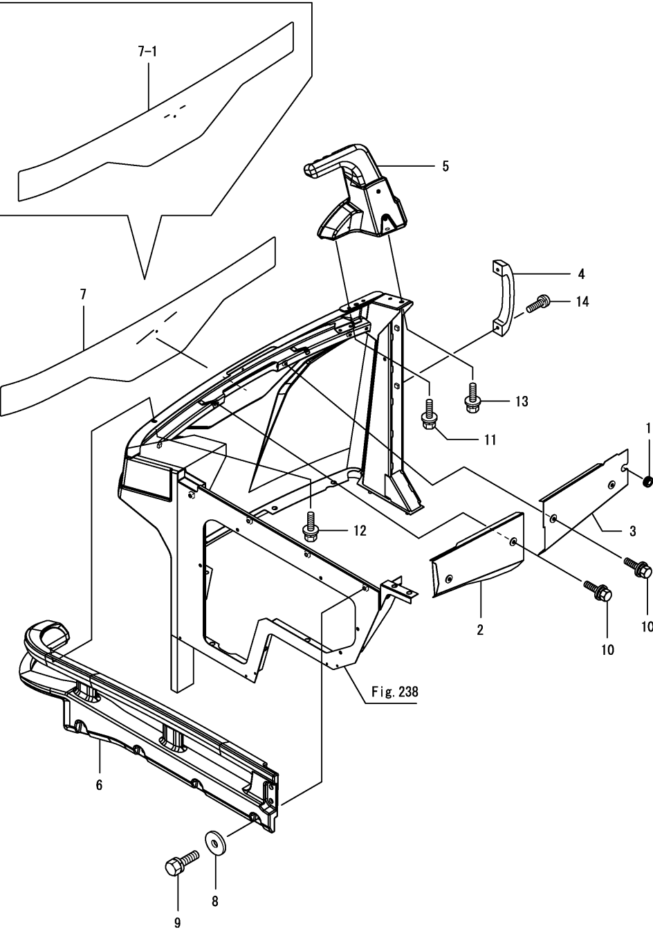
Fig.239. 바닥판의장(상)
