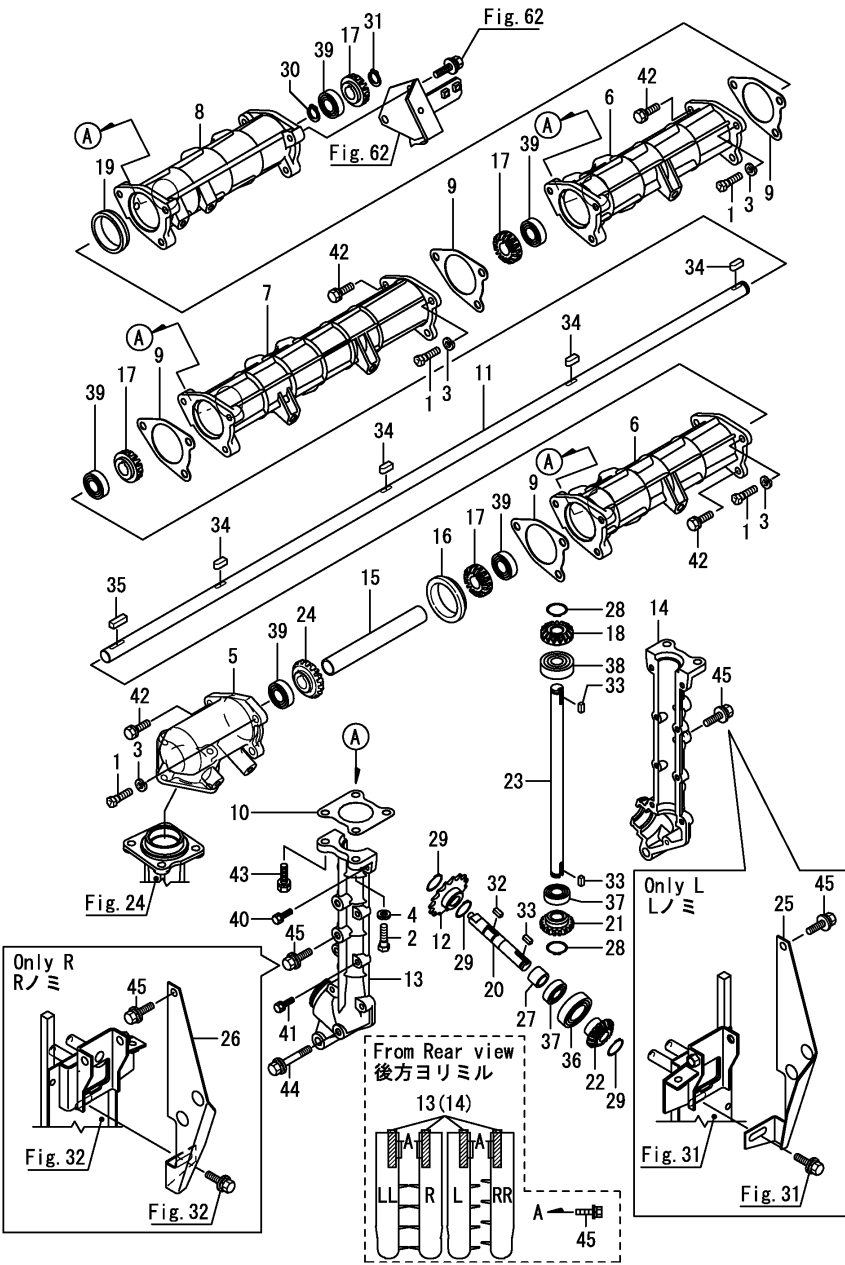
Fig.25. 픽업 수평 드라이브
