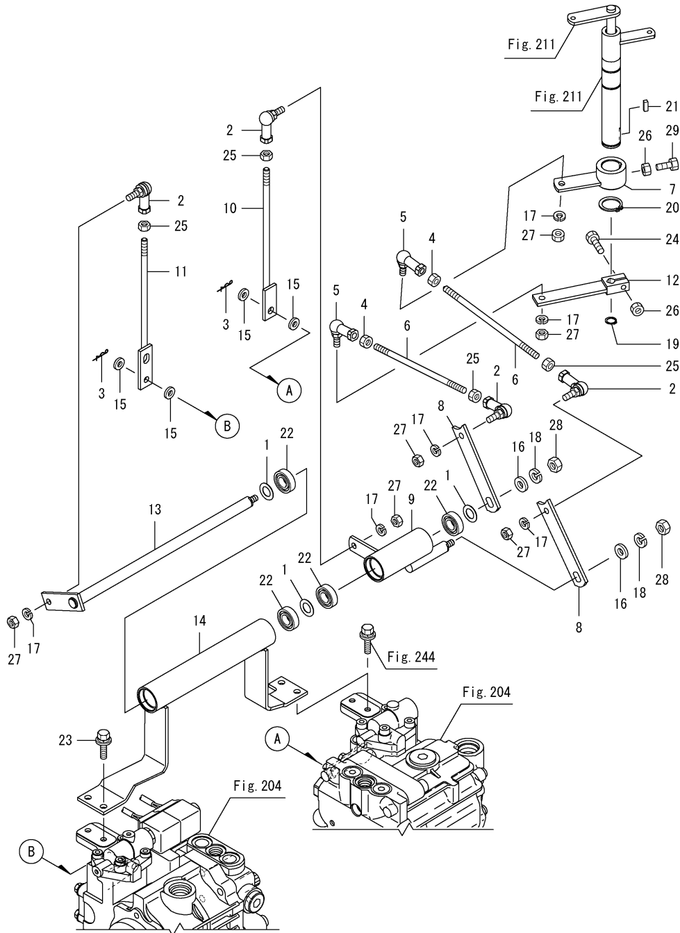
Fig.221. 조작로드
