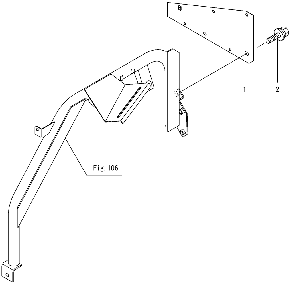
Fig.45. 방진 커버(캐빈)
