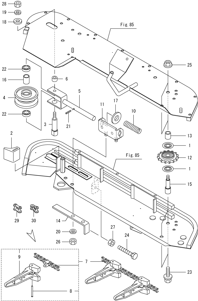
Fig.86. 상반송롤러(좌)
