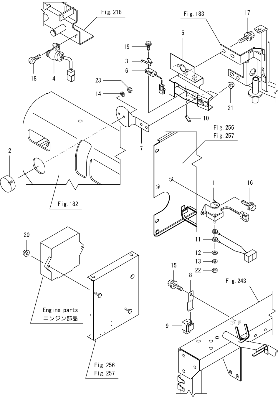
Fig.277. 전장품(엔진)
