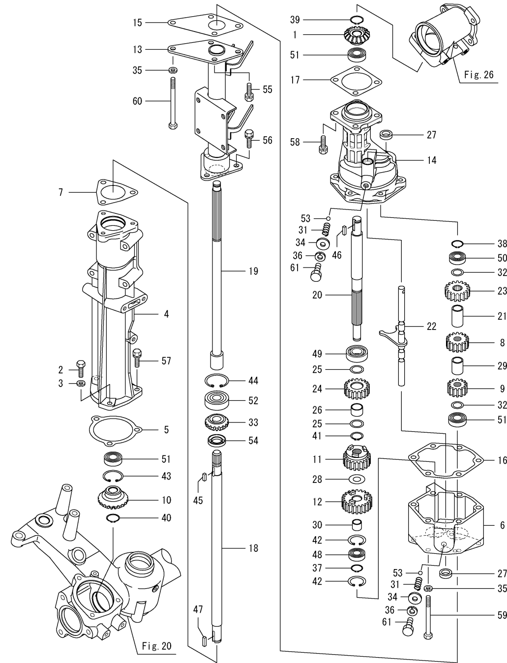
Fig.23. 픽업 수직 드라이브
