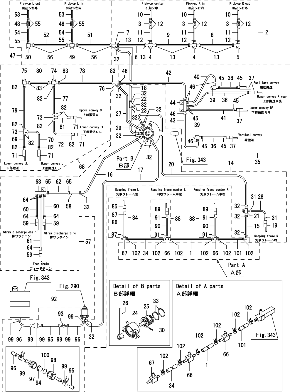
Fig.344. 주유장치(2)
