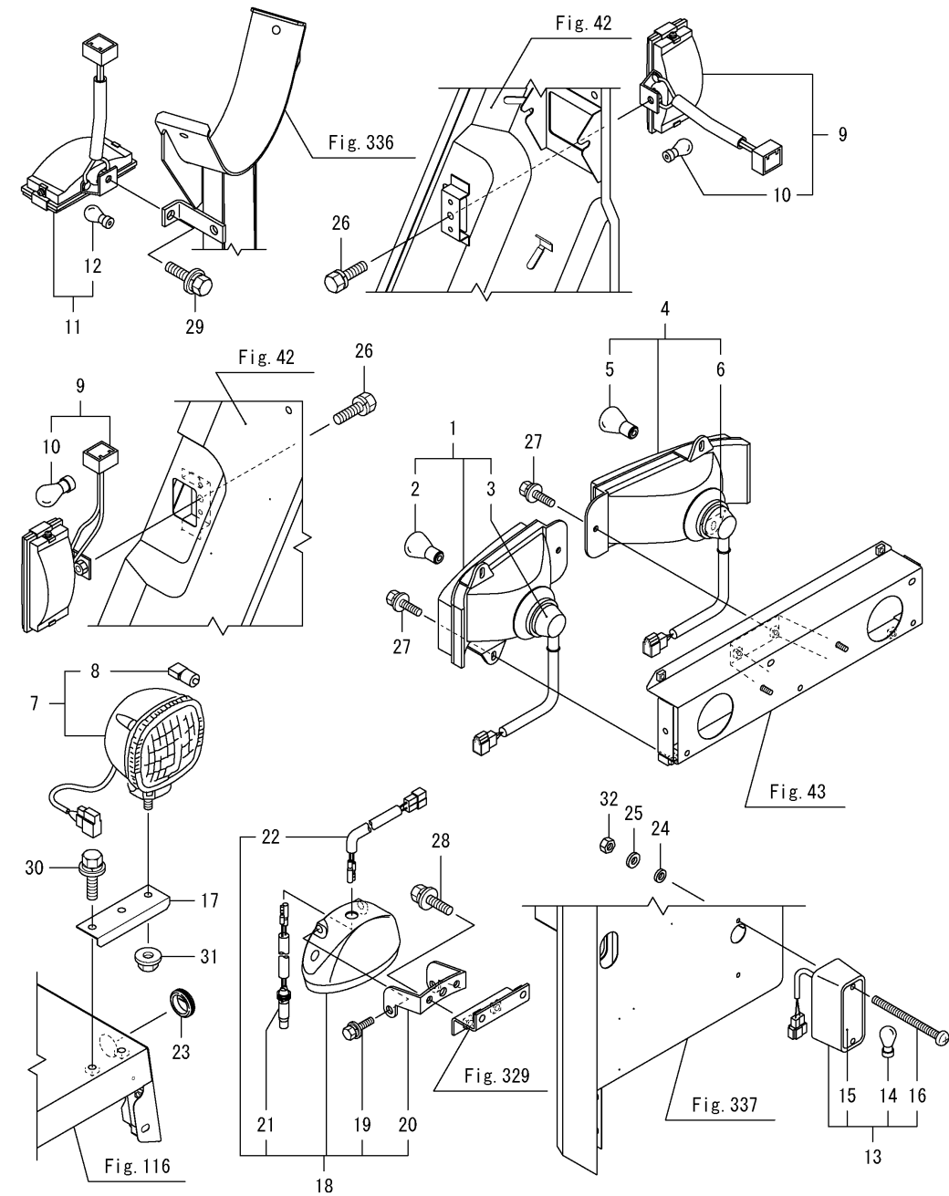
Fig.282. 램프(곡물탱크)
