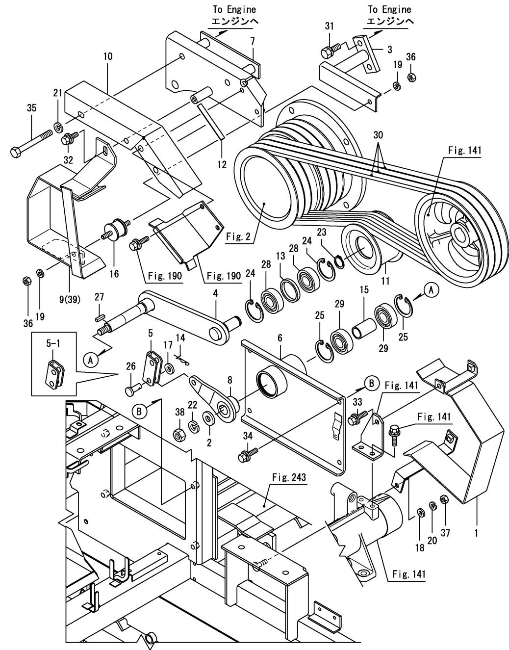
OCNP5-M34400 탈곡(1) Fig.140. 탈곡클러치
