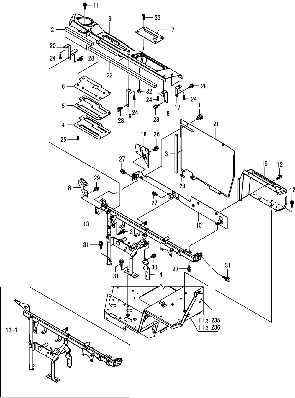
Fig.212. 측면 칼럼
