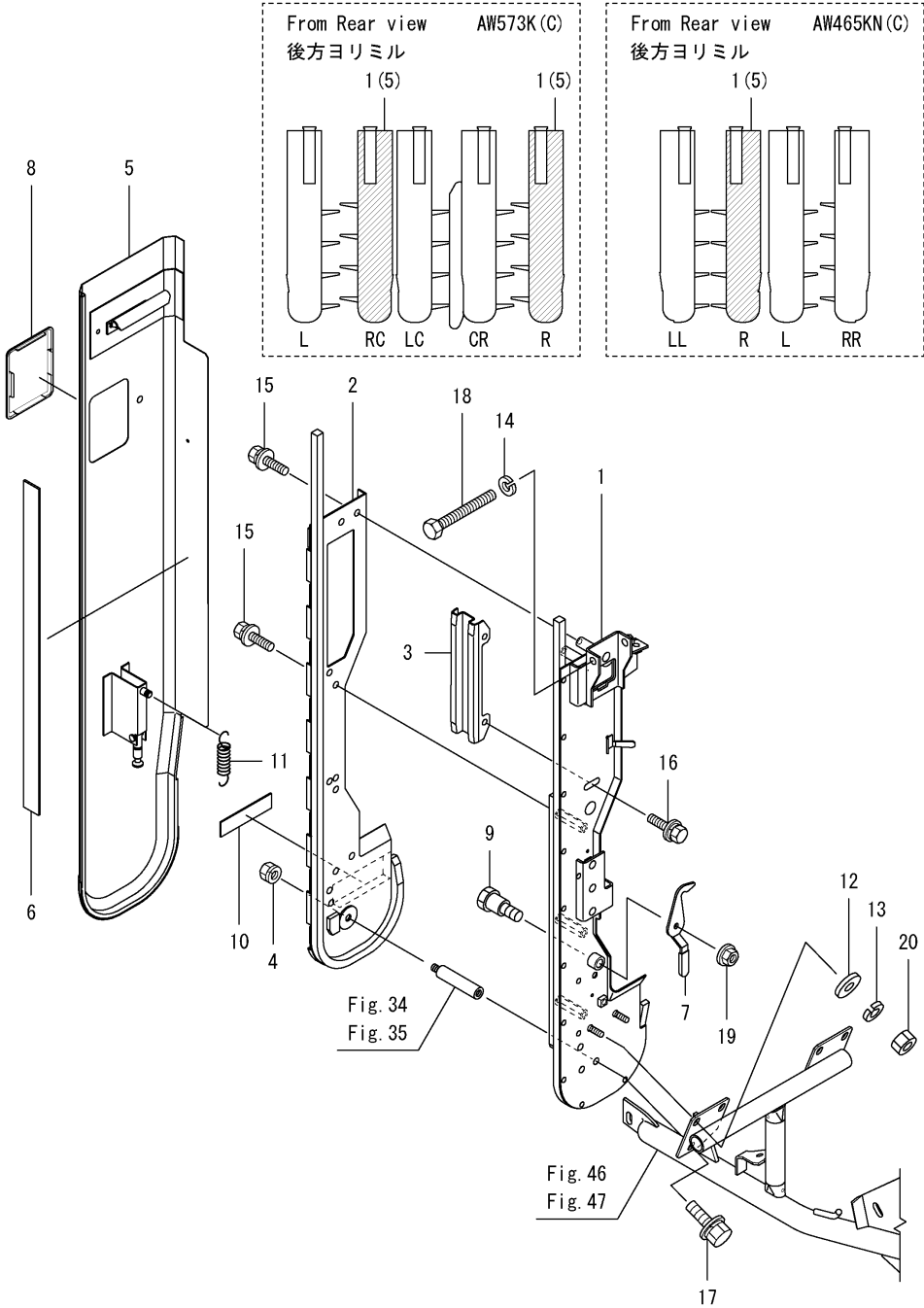
Fig.32. 픽업 케이스(오른쪽)
