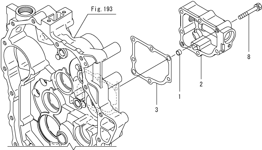
Fig.194. 측면 케이스
