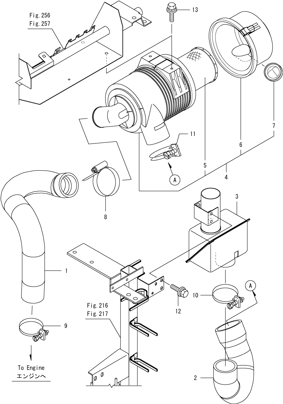
Fig.7. 에어클리너
