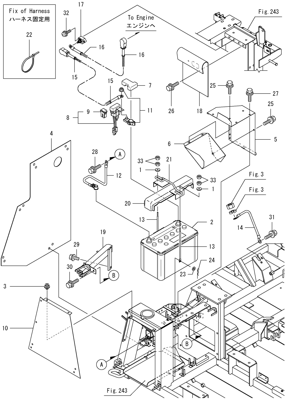
Fig.294. 배터리 및 전력 공급
