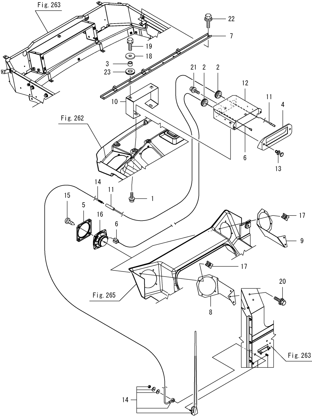
Fig.269. 스테레오
