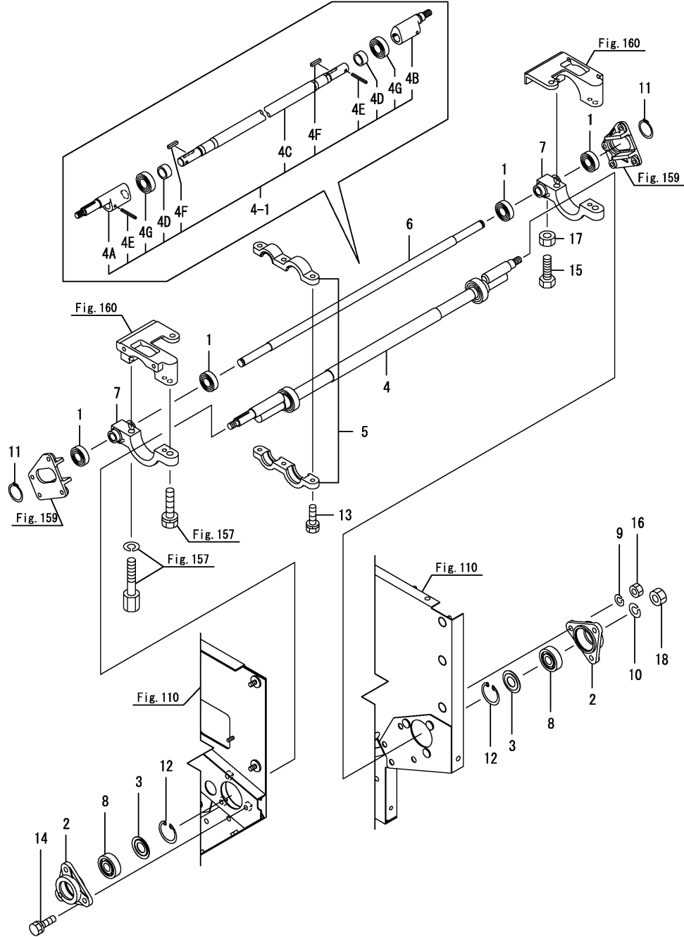
OCNP5-M34400 탈곡(2) Fig.156. 스윙 축(1)
