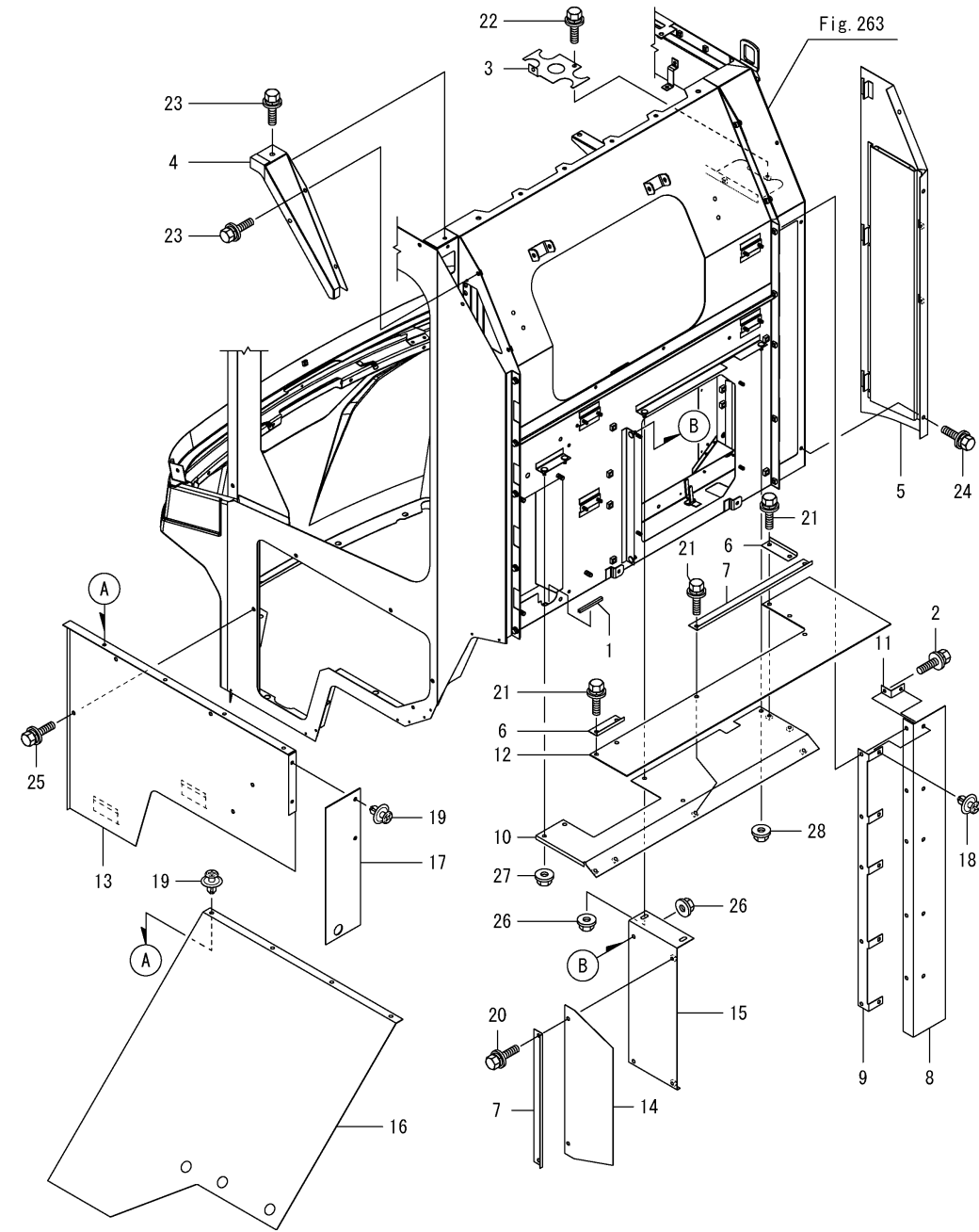
Fig.268. 캐빈시일
