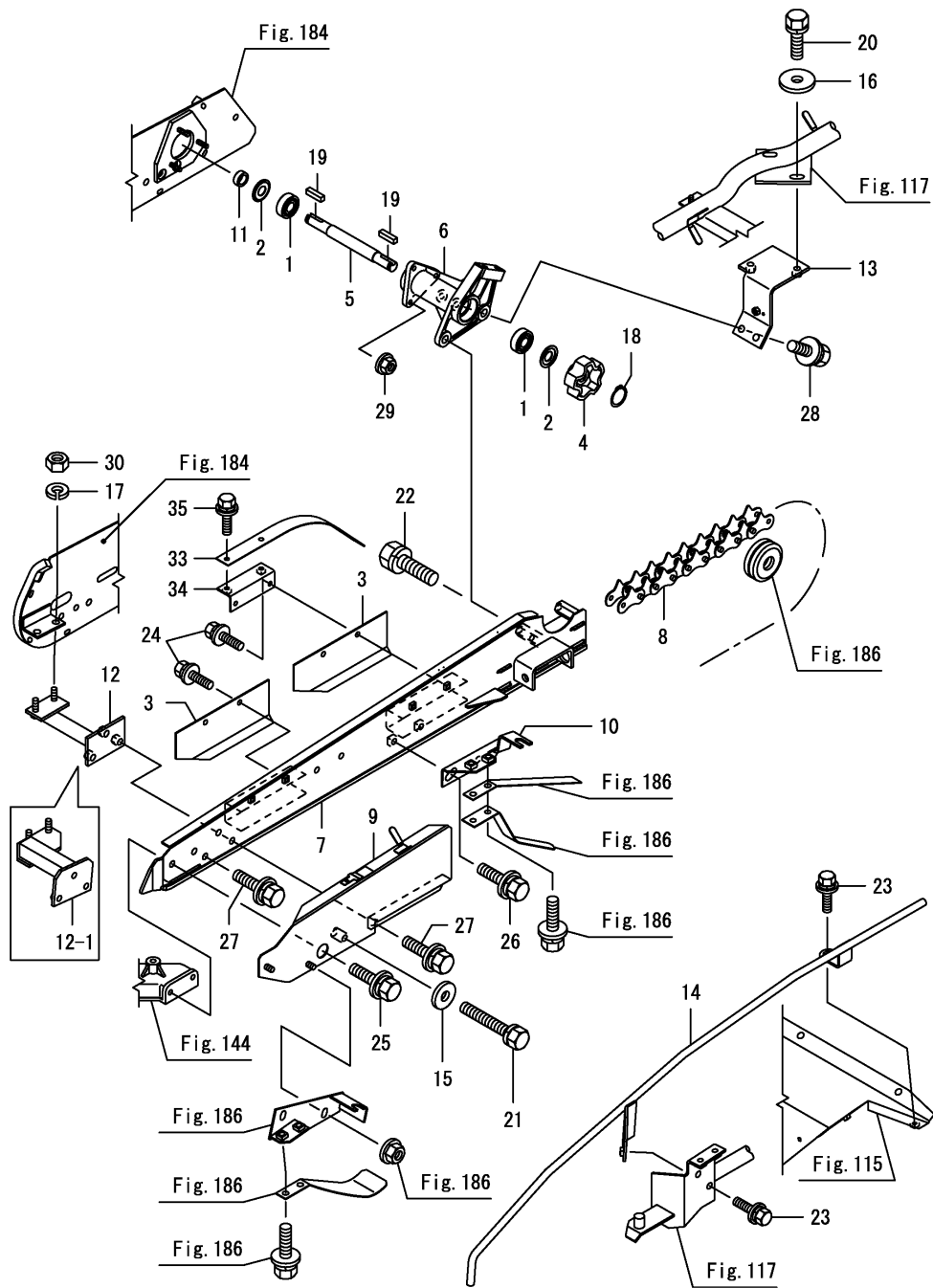
Fig.185. 쟁배출반송(2)
