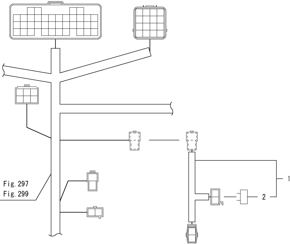
Fig.301. 배선(컴프레서)
