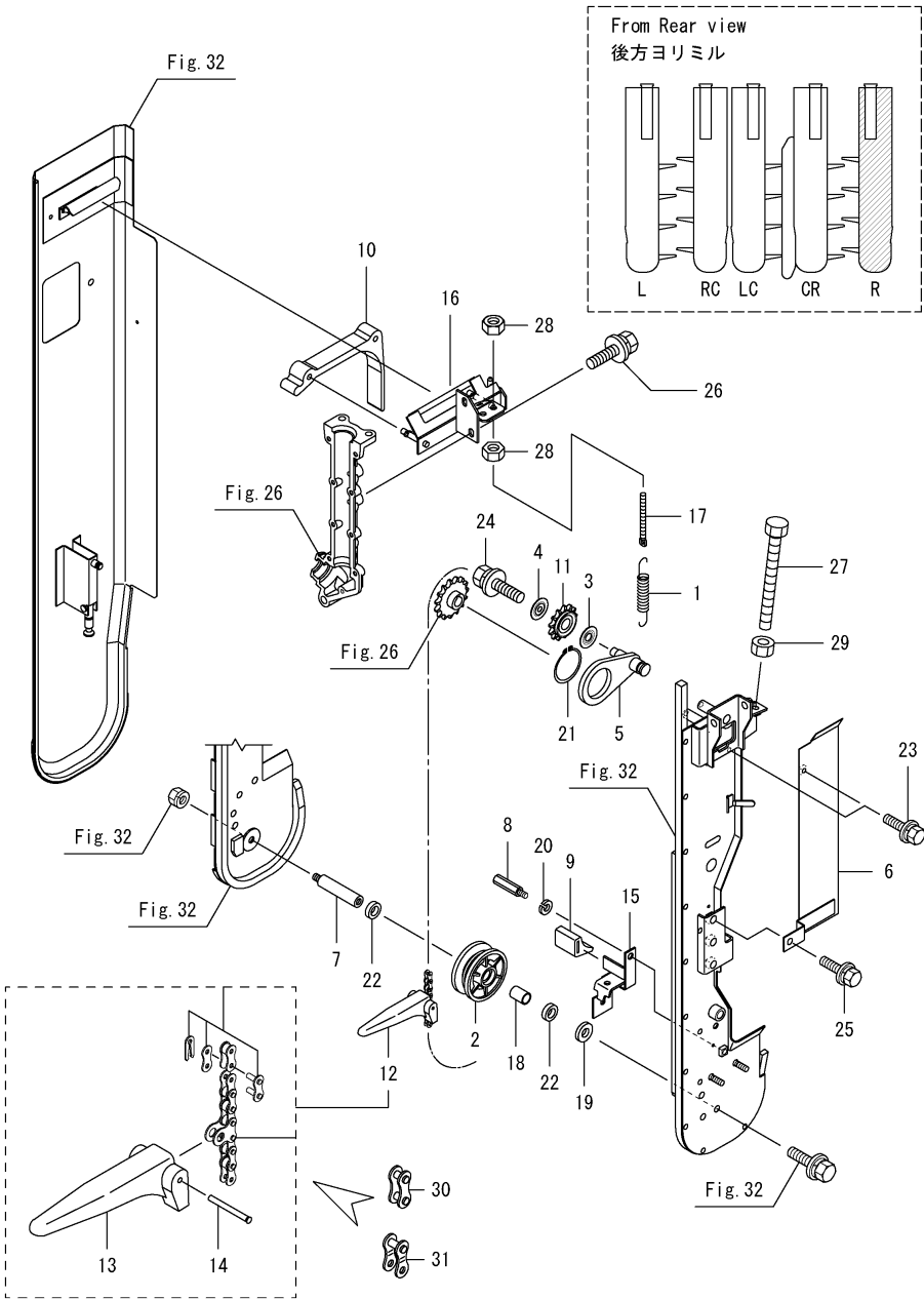
Fig.34. 인기체인롤러(우)
