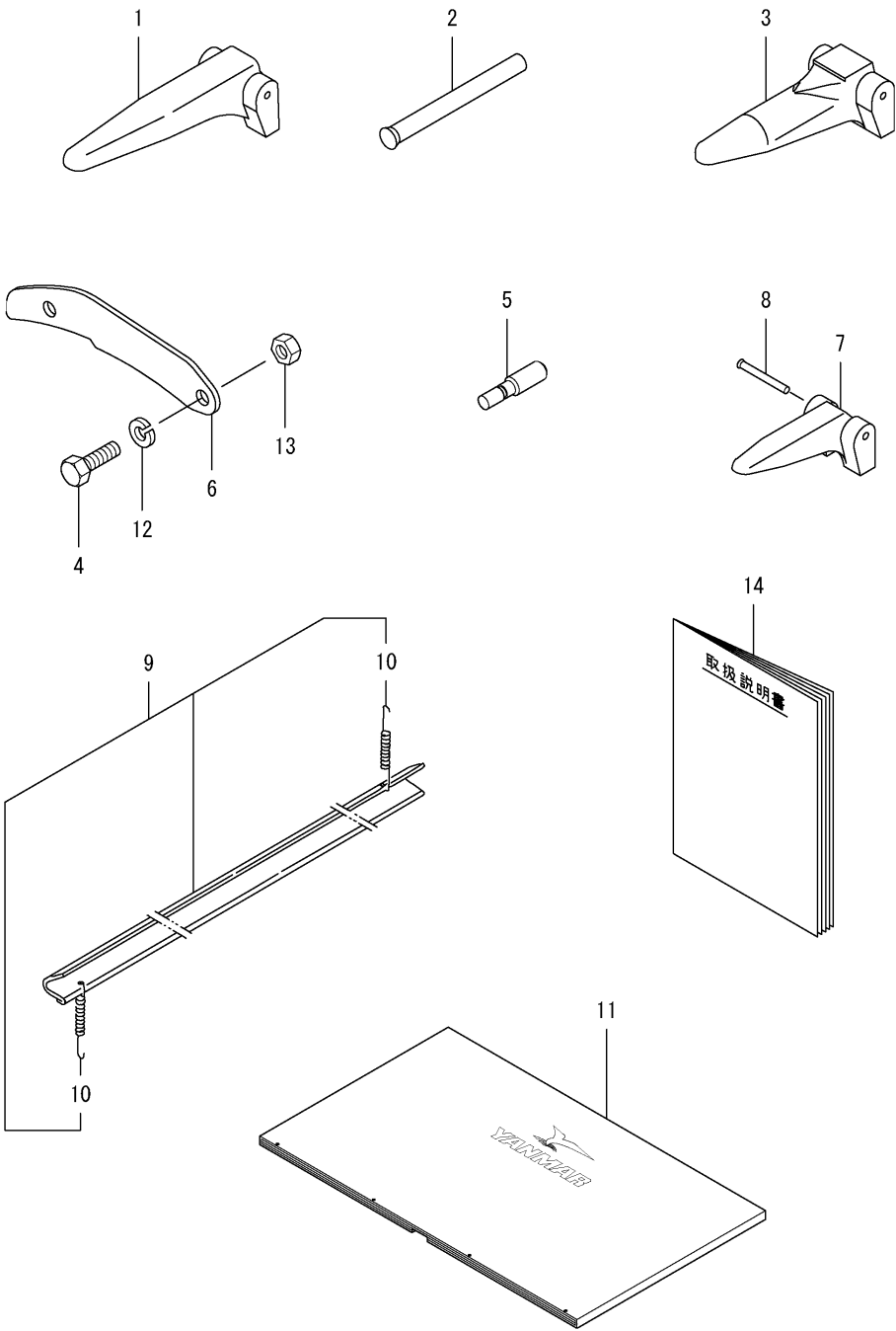
Fig.356. 부대품
