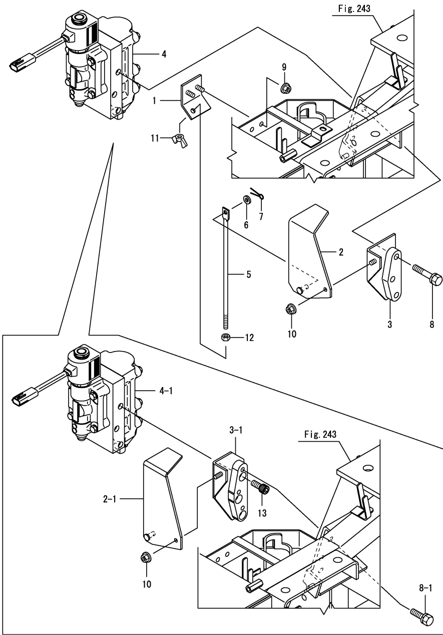
Fig.206. 클러치 실린더
