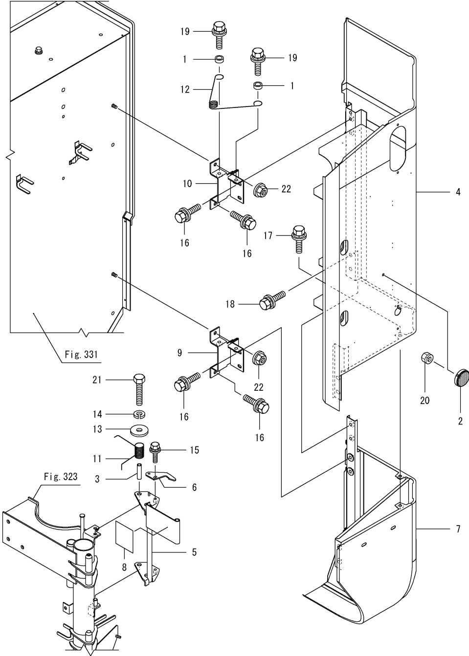
Fig.337. 탱크커버
