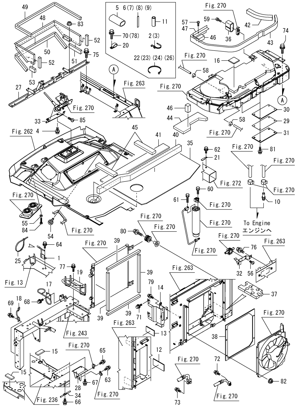
Fig.271. 에어컨취부
