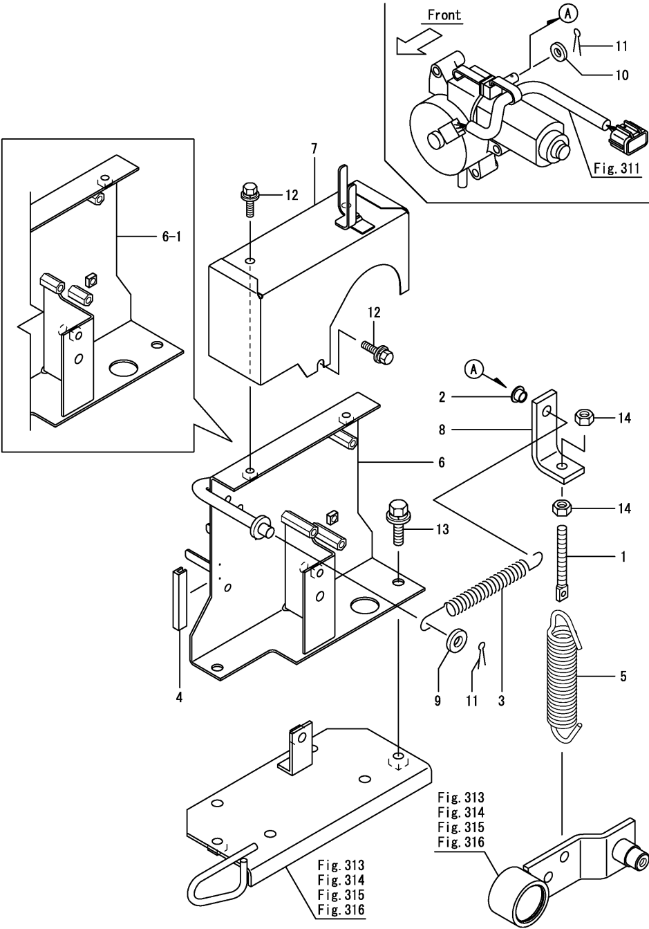
Fig.319. 오거 클러치
