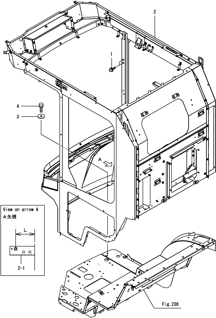
Fig.263. 캐빈(몸체)
