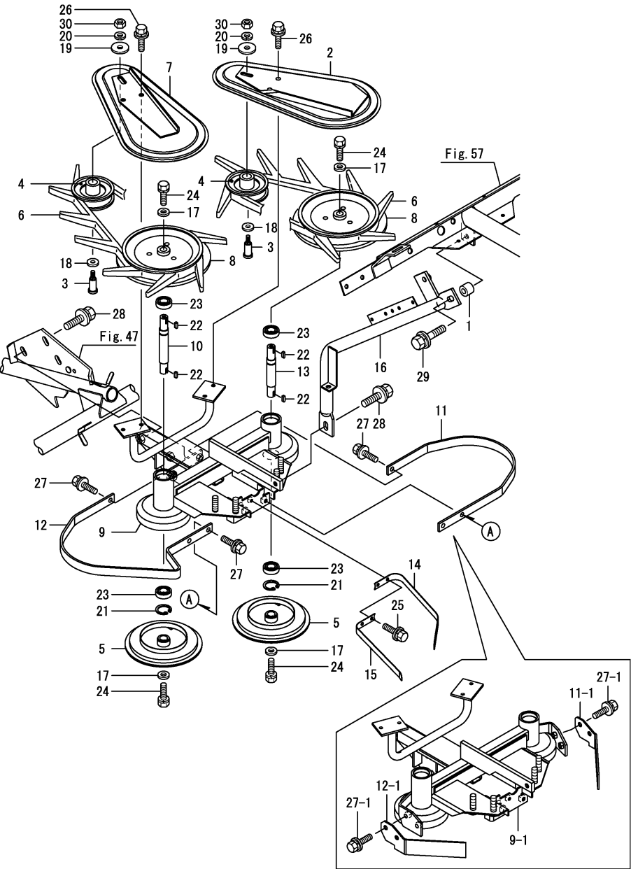
Fig.66. 끌어모음벨트(중)
